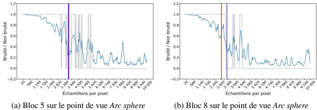
FIGURE 7.7 – Prédictions du modèle pendant le rendu du RNN sélectionné avec les données d'entrée H_{SVD} . La ligne verticale rouge correspond au seuil humain pour le bloc. La courbe bleue correspond aux prédictions du modèle pendant le rendu. La courbe en pointillés bleus fait référence à l'étiquette prédite suivant le critère strict de sélection d'étiquette (Si la probabilité est inférieure à 0,5, alors l'image est considérée comme n'étant plus bruitée, sinon, elle est toujours bruitée). La ligne bleue verticale, fait référence aux seuils prédits obtenus.
