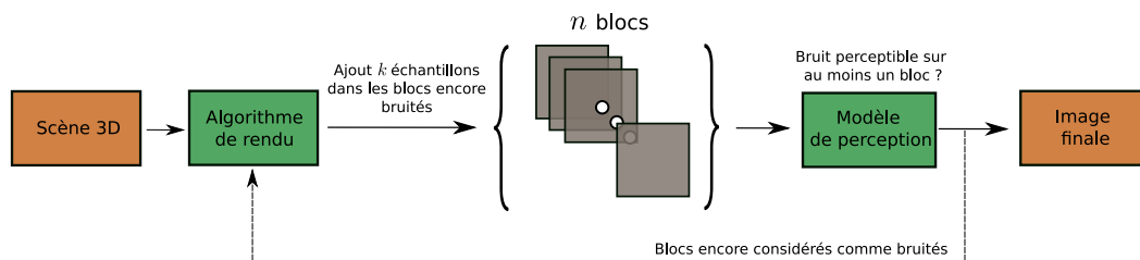
FIGURE 4.6 – Processus de rendu d'une image de synthèse avec interaction et interrogation du modèle de perception sur des parties de l'image pour permettre une meilleure précision et localisation du bruit.
