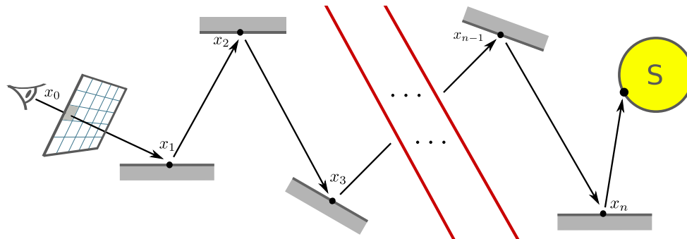
FIGURE 1.6 – Exemple de chemin généré avec la méthode du path tracing classique
