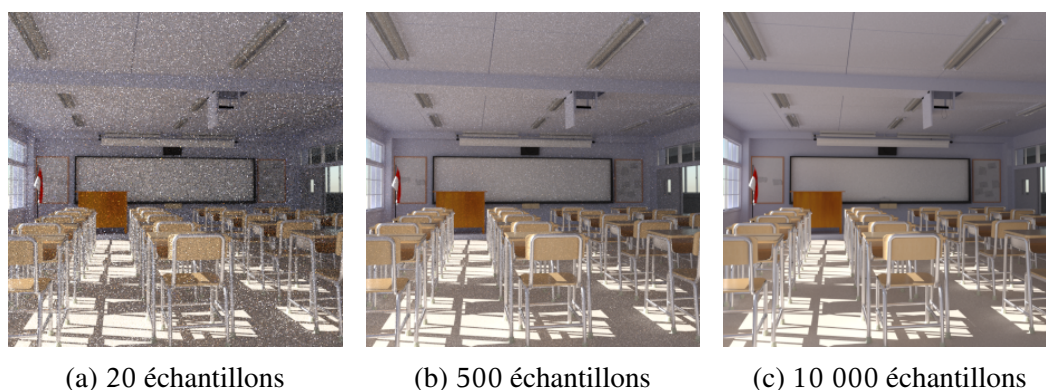
FIGURE 1.8 – Aperçu du bruit de Monte-Carlo généré avec plusieurs niveaux d'échantillons lors du rendu d'une image photo-réaliste avec l'algorithme du tracé de chemins.
