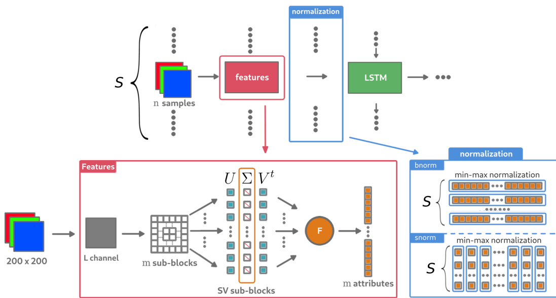
FIGURE 7.5 – Pipeline complet avec architecture RNN et paramètres testés associés. Le terme features est utilisé pour déterminer les caractéristiques (ou encore attributs) extraites de l'image.
