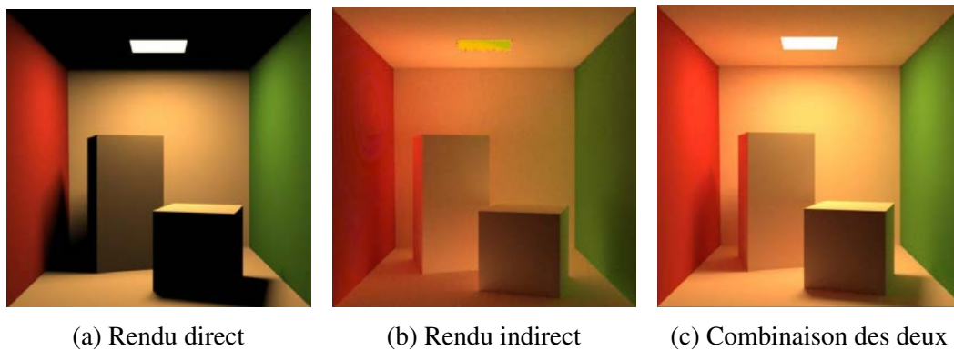
FIGURE 1.5 – Aperçu du rendu direct et indirect puis de la combinaison des deux rendus. La combinaison des deux rendus, offre une image photo-réaliste de bonne qualité permettant de mieux prendre en considération les effets de lumière
