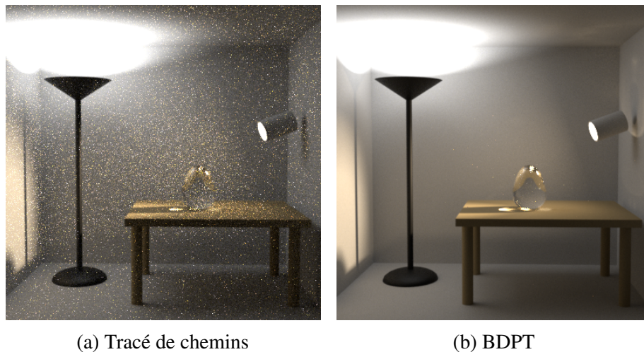
FIGURE 1.10 – Comparaisons de deux méthodes de résolutions de l'algorithme de Monte-Carlo pour 1 000 échantillons. Le tracé de chemins comporte malheureusement une variance trop importante pour estimer correctement les pixels de l'image. Il est possible de rapidement souligner les résultats assez significatifs de l'algorithme BDPT.
