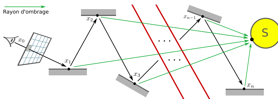
FIGURE 1.7 – Exemple de chemin généré avec la méthode du path tracing avec estimation du pas suivant. À chaque nouvelle intersection x_i , on lance un nouveau rayon d'ombrage en direction de la source lumineuse.
