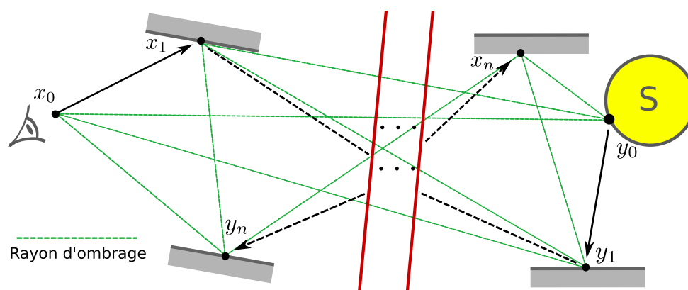
FIGURE 1.9 – Illustration de l'algorithme bidirectionnel où deux chemins sont tracés, l'un partant de la caméra, le second de la source. Les rayons d'ombrages sont générés afin d'essayer d'obtenir des interconnexions.
