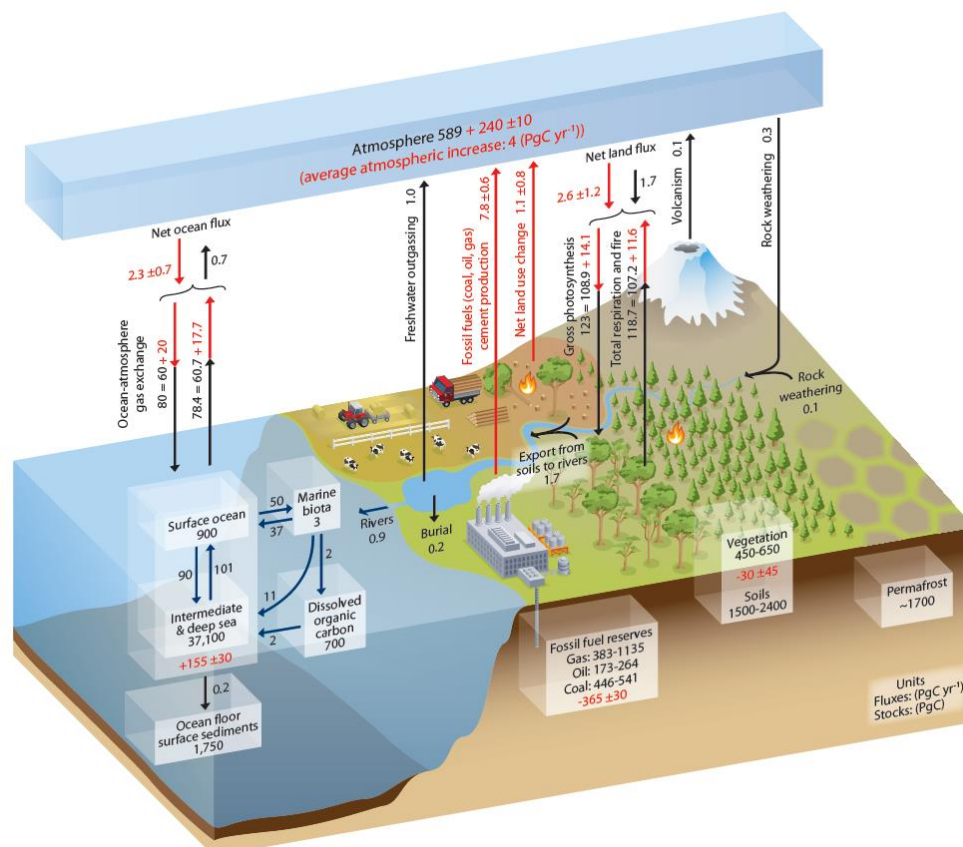
FIGURE 1.2 – Schéma simplifié du cycle global du carbone. Les chiffres représentent les stocks de carbone en Pg C et les flux annuels d'échange de carbone en \text{Pg C an}^{-1} ( 1 \text{ Pg C} = 10^{15} \text{ g C} ). Les nombres et les flèches noirs indiquent les stocks de carbone et les flux d'échange estimés pour la période antérieure à l'ère industrielle. Les flèches et les nombres rouges indiquent les flux « anthropiques » annuels en moyenne sur la période 2000-2009. Source : GIEC [2013].
