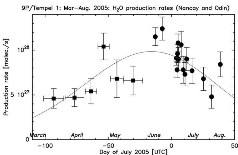
FIG. 2.3 – Les taux de production de l'eau basés à la fois sur les observations du radical OH à Nancay (carrés) et sur les observations Odin de la bande de l'eau à 557 GHz (cercles). La ligne continue correspond au taux de production déduit par un ajustement du \chi^2 . Crédit : Biver et al. (2007)
