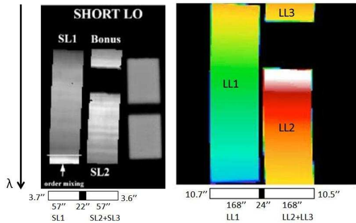
FIG. 2.16 – Les modules SL (gauche) et LL (droite) de IRS sur le détecteur. Crédit : IRS Instrument Handbook
