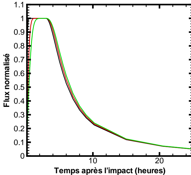
FIG. 3.23 – Evolution temporelle du flux thermique à \lambda = 5.86 \text{ } \mu\text{m} normalisé par rapport au maximum. Les sursauts sont de type gaussien de durée 1000 s (noir), 3000 s (rouge) et 5000 s (vert). Le champ de vue est de 5 \times 5 pixels. Pour la vitesse v_{ref} = 230 \text{ m s}^{-1} et q_v = 0.55 et pour la distribution en taille q = 3.3 et a_{min} = 0.1 \text{ } \mu\text{m} .
