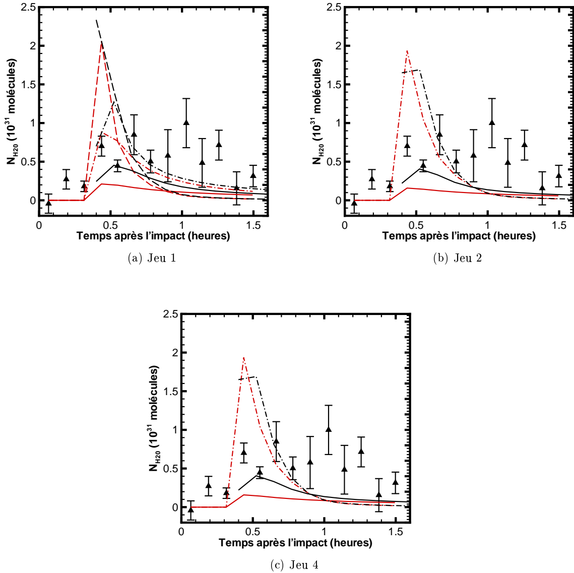
FIG. 5.21 – Modèles d'évolution temporelle de N_{\text{H}_2\text{O}} ajustés à la valeur maximale des données de Spitzer observée à \text{TI} + 0.67 \text{ h} ( (3.5 \pm 0.8) \times 10^{31} molécules). Les données de DiSanti et al. (2007) sont indiquées par des triangles. Le champ de vue est de 560 \times 560 \text{ km} . Les courbes rouges et noires correspondent respectivement au 1er et au 2ème cas limite. Les calculs ont été faits pour des grains de glace pure (trait continu), bicouches glacés (Ol) (trait long), bicouches glacés (C) (trait point) et tricouches glacés (trait-point-point).
