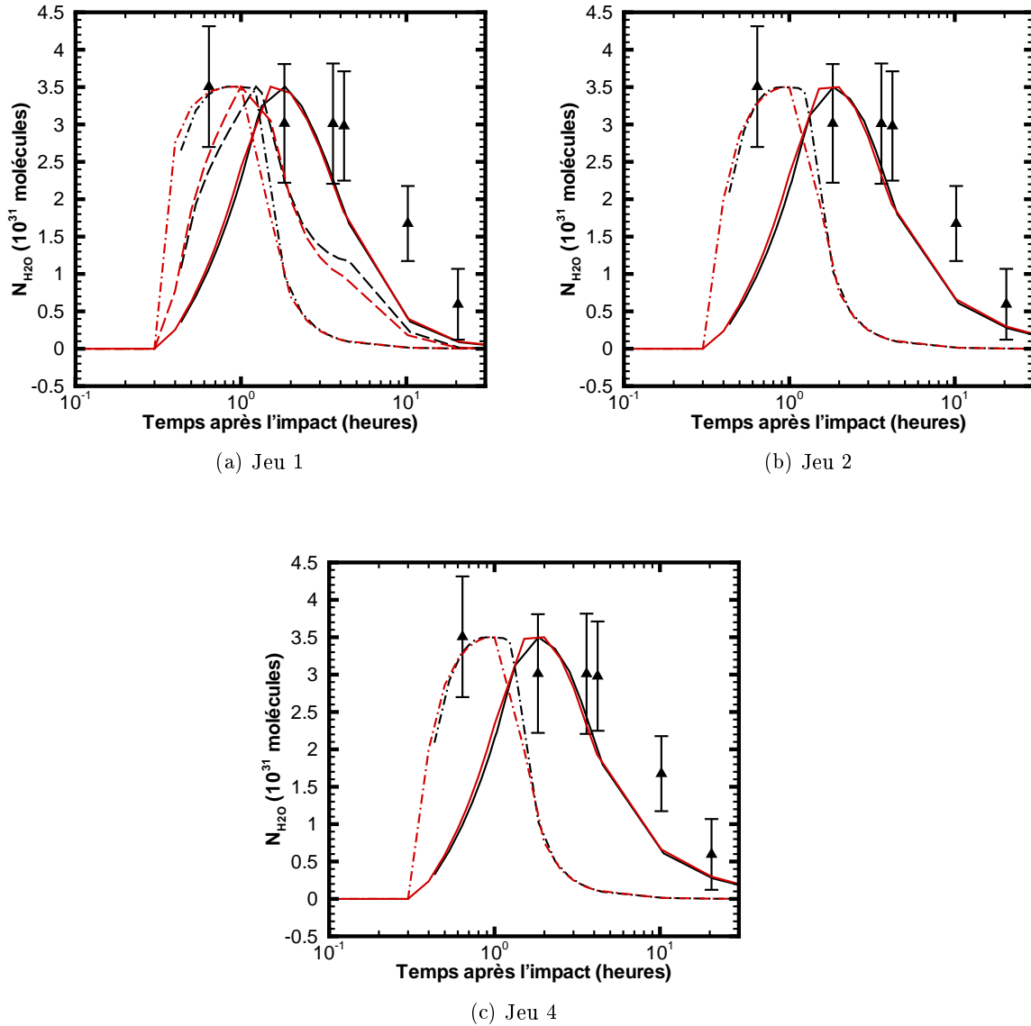
FIG. 5.20 – Modèles d'évolution temporelle de N_{\text{H}_2\text{O}} ajustés à la valeur maximale observée à \text{TI} + 0.67 \text{ h} ( (3.5 \pm 0.8) \times 10^{31} molécules). Les données sont indiquées par des triangles. Le champ de vue est de 5 \times 5 pixels. Les courbes rouges et noires correspondent respectivement au 1er et au 2ème cas limite. Les calculs ont été faits pour des grains de glace pure (trait continu), bicouches glacés (O1) (trait long), bicouches glacés (C) (trait point) et tricouches glacés (trait-point-point).
