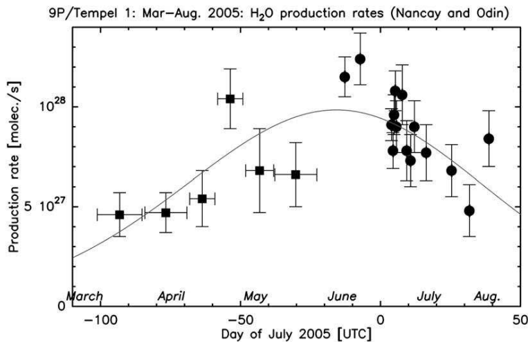
FIG. 2.3 – Les taux de production de l'eau basés à la fois sur les observations du radical OH à Nancay (carrés) et sur les observations Odin de la bande de l'eau à 557 GHz (cercles). La ligne continue correspond au taux de production déduit par un ajustement du \chi^2 . Crédit : Biver et al. (2007)
