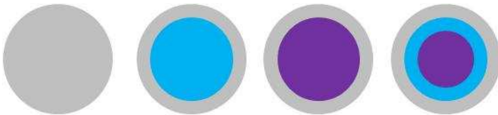
FIG. 5.6 – Représentation schématique des grains glacés d'eau pure, bicouches et tricouches. La glace d'eau est en gris, le carbone amorphe en bleu et l'olivine amorphe en violet.
