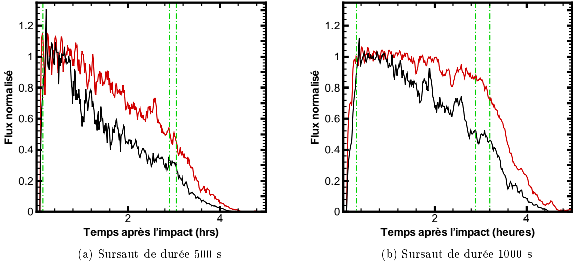
FIG. 3.20 – Evolution temporelle du Flux thermique à \lambda = 5.86 \mu\text{m} par rapport au maximum avec la procédure d'intégration de NAG. Les sursauts sont de type porte (noir) et de type gaussien (rouge). Le champ de vue est de 5 \times 5 pixels. Pour la vitesse v_{ref} = 230 \text{ m s}^{-1} et pour la distribution en taille q = 3.3 et a_{min} = 0.1 \mu\text{m} .
