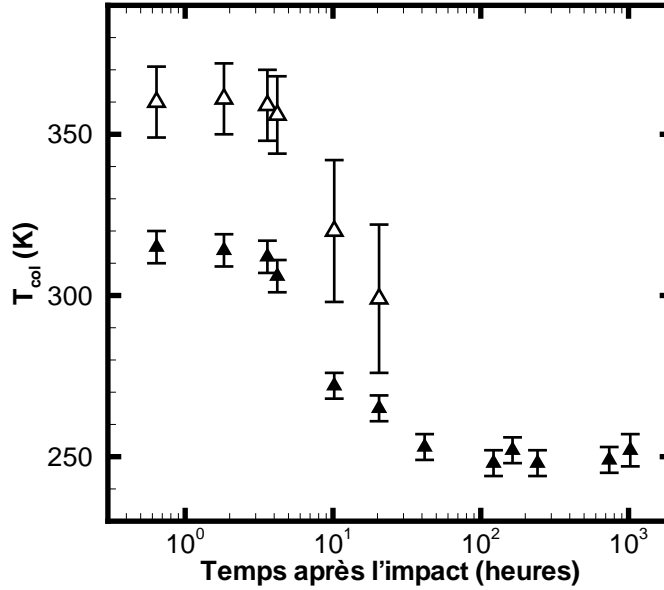
FIG. 3.3 – Température de couleur en fonction du temps après l'impact, des poussières de 9P/Tempel 1 déterminée à partir des données Spitzer par la méthode analytique pour : l'ensemble de la coma de poussière (coma ambiante et éjectas) (noir) et les éjectas de poussière (blanc). Le champ de vue est de 5 \times 5 pixels centré sur le noyau.
