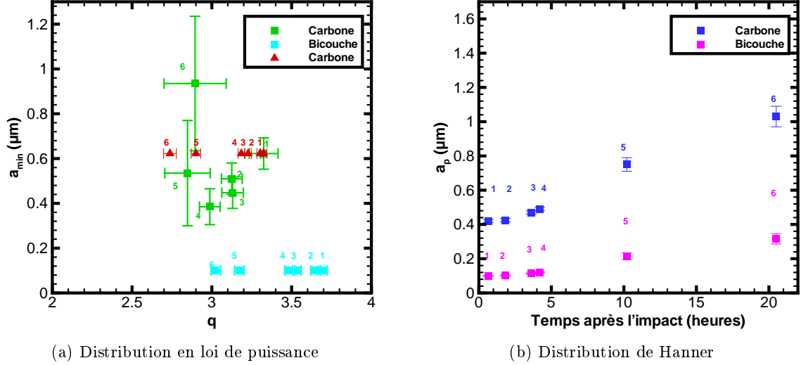
FIG. 3.17 – Paramètres pour les lois de distribution en taille obtenus par les ajustements du modèle au continuum des éjectas de poussière dans les spectres de Spitzer . Nombre 1 = TI + 0.67 h, Nombre 2 = TI + 1.83 h, Nombre 3 = TI + 3.6 h, Nombre 4 = TI + 4.2 h, Nombre 5 = TI + 10.2 h, Nombre 6 = TI + 20.5 h.
