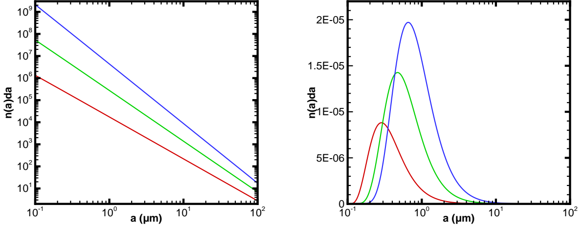
(a) Distribution en loi de puissance avec q = 2.9 (rouge), q = 3.3 (vert) et q = 3.7 (bleu) (b) Distribution de Hanner avec M_h = 5 (rouge), M_h = 10 (vert) et M_h = 15 (bleu)
