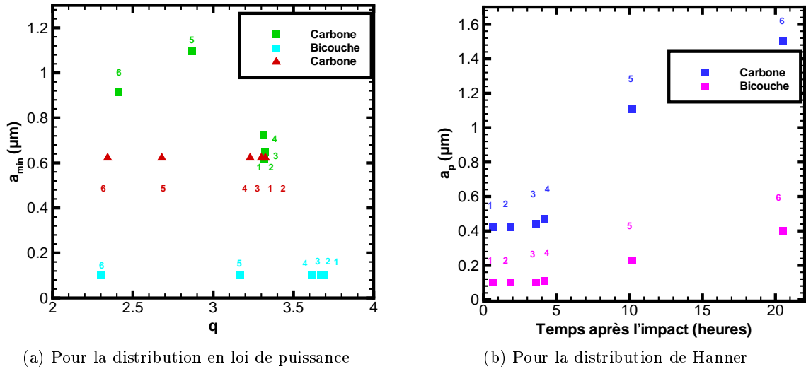
FIG. 3.31 – Paramètres théoriques pour les lois de distribution en taille obtenus par les ajustements du modèle au continuum des éjectas de poussière. Nombre 1 = TI + 0.67 h, Nombre 2 = TI + 1.83 h, Nombre 3 = TI + 3.6 h, Nombre 4 = TI + 4.2 h, Nombre 5 = TI + 10.2 h, Nombre 6 = TI + 20.5 h.
