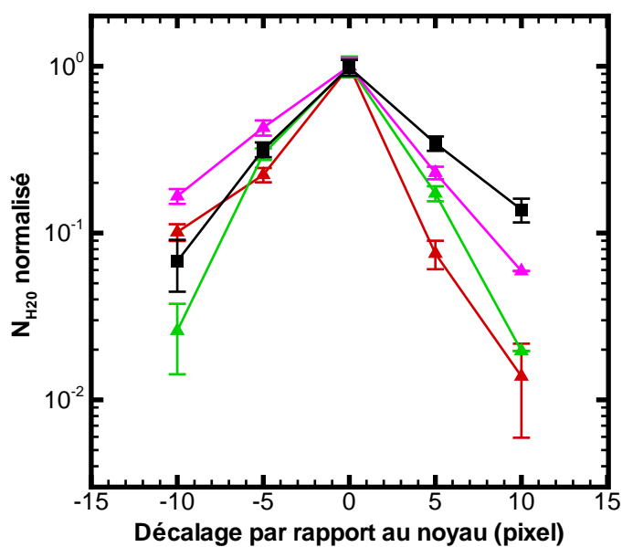
FIG. 4.11 – Nombre de molécules d'eau total pour un champ de vue de 5 \times 5 pixels de Spitzer , à \text{TI} + 0.67 h (rouge), à \text{TI} + 3.6 h (vert), à \text{TI} + 10.2 h (rose) et pour la moyenne des deux temps avant l'impact (noir).
