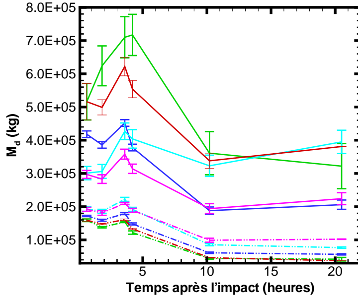
FIG. 3.18 – Evolution temporelle de la masse des éjectas de poussière ( M_d ) dans le champ de vue de Spitzer centré sur le noyau ( 5 \times 5 pixels). Les masses dans le domaine de taille a_{min}-10 \mu\text{m} ( a_{min}-100 \mu\text{m} ) sont reliées par des pointillés (respectivement des traits continus). Les différentes couleurs correspondent aux deux distributions en taille et aux deux compositions de grains : la distribution en taille en loi de puissance avec des grains de carbone amorphe lorsque a_{min} est un paramètre libre (vert), lorsque a_{min} = 0.62 \mu\text{m} et avec des grains bicouches (cyan) ; la distribution en taille de type Hanner avec des grains de carbone amorphe (bleu) et avec des grains bicouches (rose).
