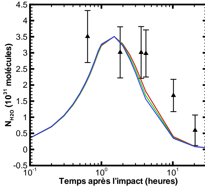
FIG. 5.13 – Modèles d'évolution temporelle de N_{\text{H}_2\text{O}} ajustés à la valeur maximale observée à TI + 0.67 h ( (3.5 \pm 0.8) \times 10^{31} molécules). Le champ de vue est de 5 x 5 pixels. Les résultats sont obtenus pour le modèle dense avec pour la distribution en taille en loi de puissance a_{min} = 0.1 \mu\text{m} et q = 3.7 et pour la loi de vitesse q_v = 0.55 et v_{ref} = 210 \text{ m s}^{-1} (rouge), 230 \text{ m s}^{-1} (vert) et 250 \text{ m s}^{-1} (bleu).
