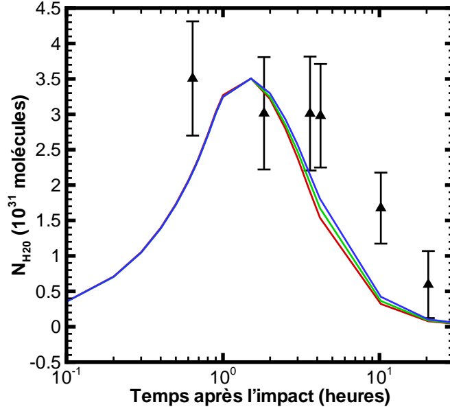
FIG. 5.14 – Modèles d’évolution temporelle de N_{\text{H}_2\text{O}} ajustés à la valeur maximale observée à TI + 0.67 h ( (3.5 \pm 0.8) \times 10^{31} molécules). Le champ de vue est de 5 x 5 pixels. Les résultats sont obtenus pour le modèle dense avec pour la distribution en taille en loi de puissance a_{min} = 0.1 \mu\text{m} et q = 3.7 et pour la loi de vitesse v_{ref} = 230 \text{ m s}^{-1} et q_v = 0.3 (rouge), 0.4 (vert) et 0.5 (bleu).
