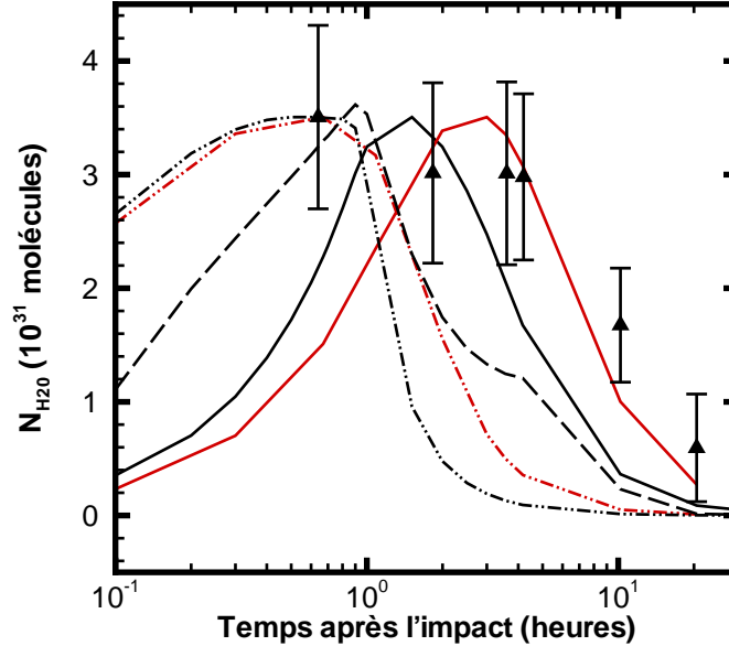
FIG. 5.18 – Modèles d'évolution temporelle de N_{\text{H}_2\text{O}} ajustés à la valeur maximale observée à \text{TI} + 0.67 \text{ h} ( (3.5 \pm 0.8) \times 10^{31} molécules). Les données sont indiquées par des triangles. Le champ de vue est de 5 \times 5 pixels. Pour la distribution en taille en loi de puissance a_{\text{min}} = 0.1 \mu\text{m} et q = 3.7 et pour la loi de vitesse v_{\text{ref}} = 230 \text{ m s}^{-1} et q_v = 0.4 . Les calculs ont été effectués dans l'approximation dense (noir) et raréfié (rouge) et pour des grains de glace d'eau pure (trait continu), des grains tricouches glacés avec \alpha_{\text{ice}} = 0.9 (trait-point-point) et des grains bicouches glacés avec un cœur d'olivine amorphe et \alpha_{\text{ice}} = 0.98 (trait long).
