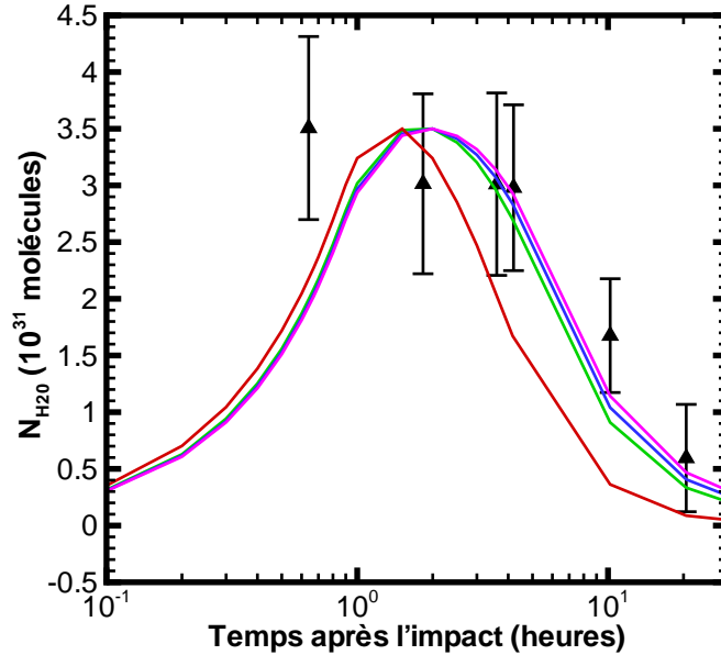
FIG. 5.12 – Modèles d'évolution temporelle de N_{\text{H}_2\text{O}} ajustés à la valeur maximale observée à \text{TI} + 0.67 \text{ h} ( (3.5 \pm 0.8) \times 10^{31} molécules). Le champ de vue est de 5 \times 5 pixels. Les résultats sont obtenus pour le modèle dense avec pour la loi de vitesse v_{ref} = 230 \text{ m s}^{-1} et q_v = 0.4 et pour la distribution de Hanner M_h = 0 (rouge), 8 (vert), 12 (bleu) et 16 (rose) (correspondant respectivement à a_p = 0.1 \mu\text{m} , 0.3 \mu\text{m} , 0.4 \mu\text{m} et 0.5 \mu\text{m} ).
