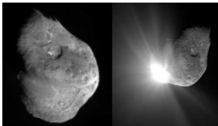
FIG. 2.10 – Noyau de la comète 9P/Tempel 1 avant (gauche) et après (droite) l'impact de Deep Impact . Crédit : NASA/JPL-Caltech/UMD.
