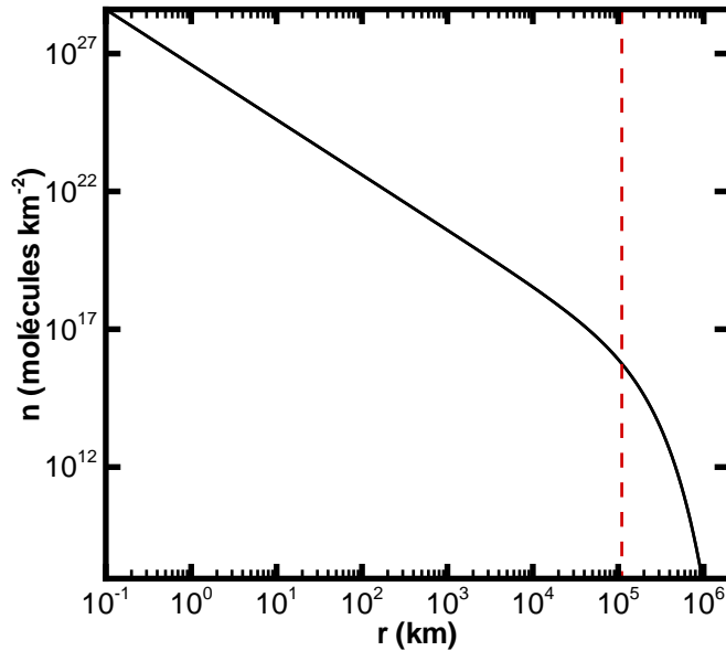
FIG. 4.6 – Evolution de la densité n d' \text{H}_2\text{O} en fonction de la distance au noyau r (noir) à r_h = 1 UA avec v_{exp} = 0.75 km s ^{-1} et Q = 5.0 \times 10^{27} molécules s ^{-1} et la longueur d'échelle L_{\text{H}_2\text{O}} (rouge).
