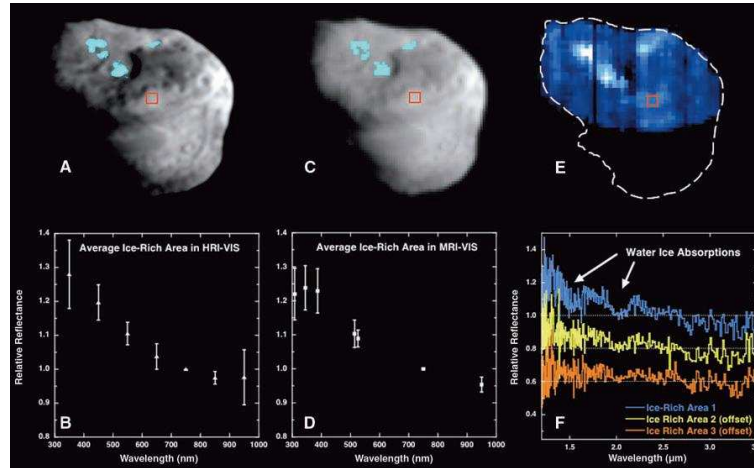
FIG. 5.3 – Cartes et spectres, obtenus à partir des instruments à bord de la sonde Deep Impact , des zones riches en glace par rapport aux régions pauvres en glace du noyau de la comète 9P/Tempel 1. A et B sont obtenus avec les données dans le visible de HRI, C et D avec les données dans le visible de MRI et E et F avec les données dans l'infrarouge de IR. Trois régions riches en glace (bleu clair) ont été localisées près des régions localement froides avec respectivement des températures d'environ 285, 290 et 295 K. Crédit : Sunshine et al. (2006).
