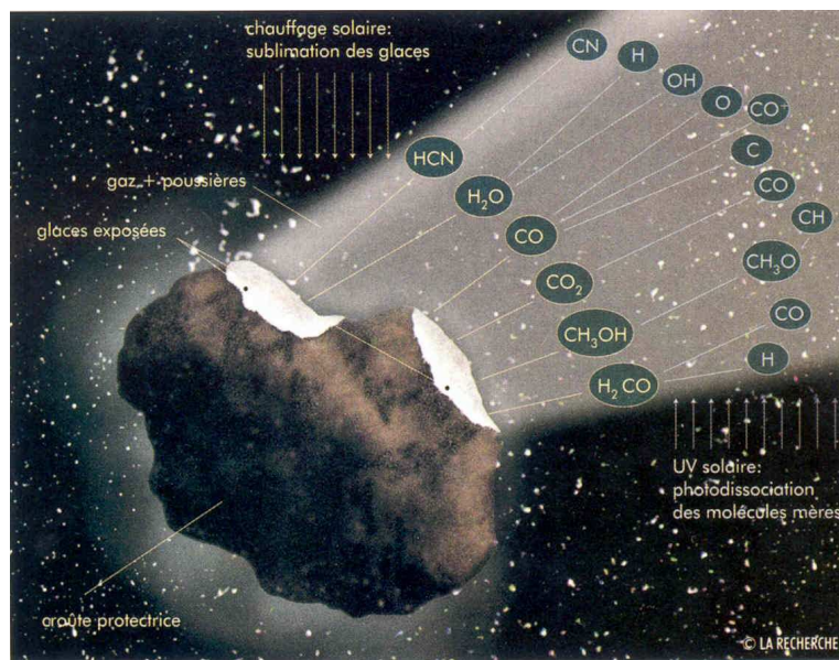
FIG. 1.5 – Processus physiques de l'activité cométaire.
