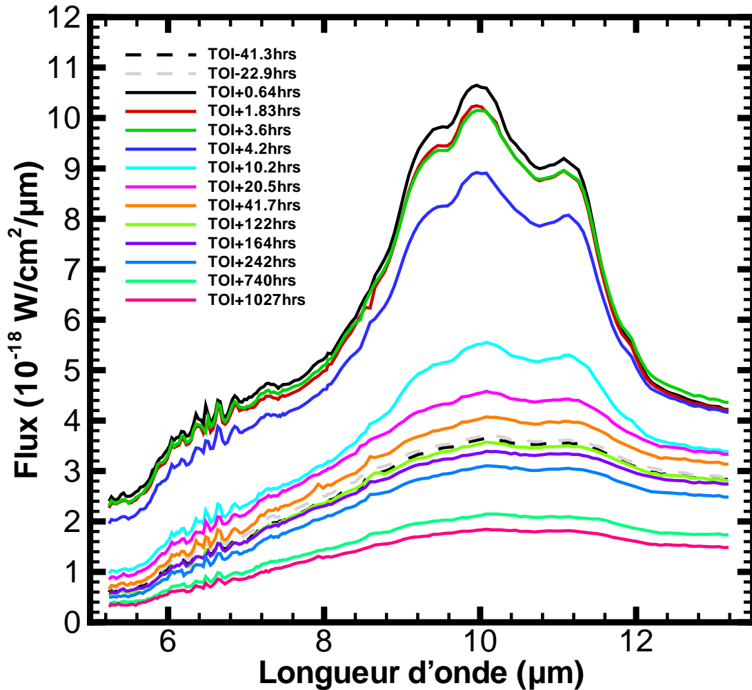
FIG. 2.19 – Spectre de la coma après soustraction de l'émission du noyau pour un champ de vue de 5 \times 5 pixels ( 9.25'' \times 9.25'' ) centré sur le noyau pour les données de SL1, SL2 et SL3.
