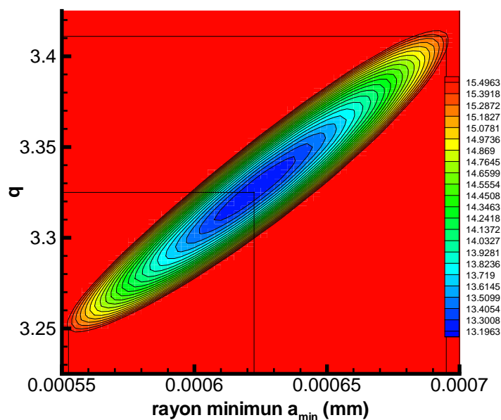
FIG. 3.15 – Courbe d'isocontour de \chi^2 obtenus pour les paramètres a_{\min} et q de la distribution en taille en loi de puissance dans le cas de grains de carbone amorphe. Le spectre analysé est celui des éjectas de poussière obtenu pour une extraction de 5 \times 5 pixels centrée sur le noyau à TI + 0.67 h. L'échelle de couleur du rouge au bleu correspond aux valeurs décroissantes du \chi^2 .
