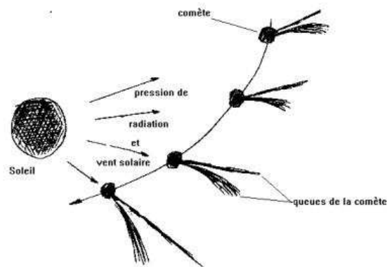
FIG. 1.6 – Orientation des queues cométaires par rapport au Soleil.
