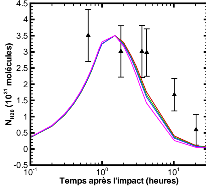
FIG. 5.11 – Modèles d'évolution temporelle de N_{\text{H}_2\text{O}} ajustés à la valeur maximale observée à \text{TI} + 0.67 \text{ h} ( (3.5 \pm 0.8) \times 10^{31} molécules). Le champ de vue est de 5 \times 5 pixels. Les résultats sont obtenus pour le modèle dense avec pour la loi de vitesse v_{ref} = 230 \text{ m s}^{-1} et q_v = 0.4 et pour la distribution en taille en loi de puissance a_{min} = 0.1 \mu\text{m} et q = 3.5 (rouge), 3.7 (vert), 3.9 (bleu) et 4.5 (rose).
