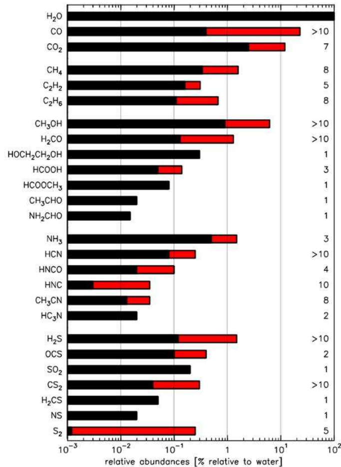
FIG. 1.4 – Les molécules mères cométaires : abondances minimale (noir) et maximale (rouge) mesurées. Le nombre indiqué à droite est celui de comètes dans lesquelles la molécule a été observée. L'abondance d'une molécule est le rapport de son taux de production à celui de l'eau. Crédit : Bockelée-Morvan et al. (2004).
