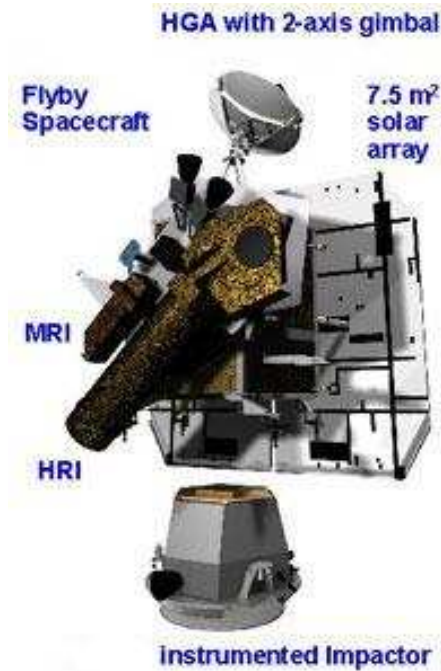
FIG. 2.6 – Le système de vol de Deep Impact . Crédit : NASA.
