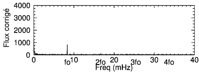
Figure 3-47 : Spectre de Fourier de la photométrie calculée sur toute la fenêtre étoile après les corrections de fond de ciel et d'offset en ppm. L'échelle de l'axe y est prolongée à 4000 ppm pour permettre la comparaison avec la photométrie d'ouverture de la Figure 3-51. f_0 et ses multiples sont indiqués sur l'axe des x pour simplifier leur identification.
