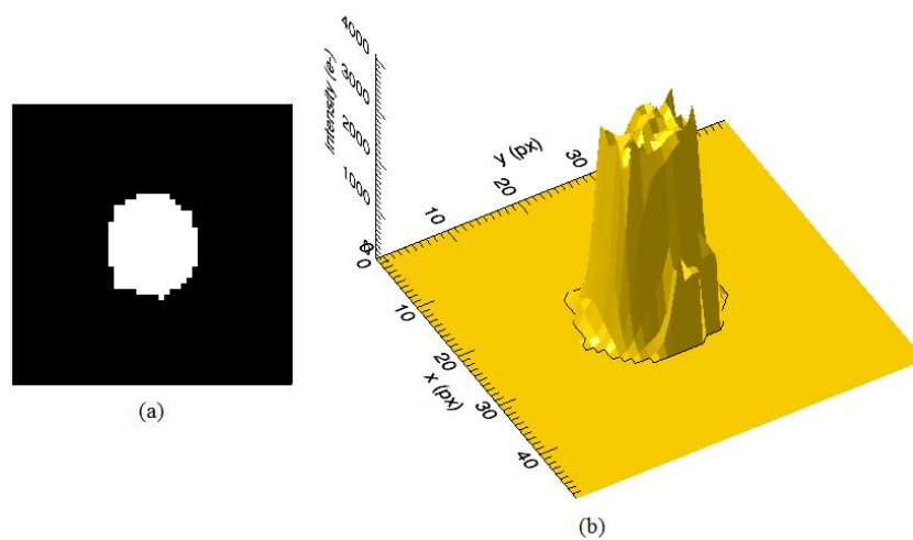
Figure 5-22 : (a) Masque grossier. (b) Masque grossier appliqué à l'étoile cible de m_v = 9 . A comparer à la Figure 5-18.
