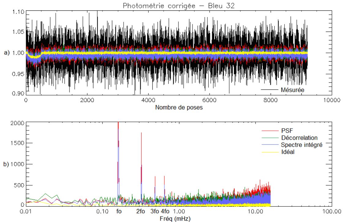
Figure 3-39 : a) Photométries d'ouverture 32 sec dans le bleu corrigées du jitter comparées à l'idéal et b) leurs spectres de Fourier. La figure a) contient aussi le flux mesuré en noir à titre de comparaison avec ceux corrigés. Le spectre de Fourier ne contient pas le transit stellaire, ce qui nous permet d'évaluer précisément le bruit du jitter.
