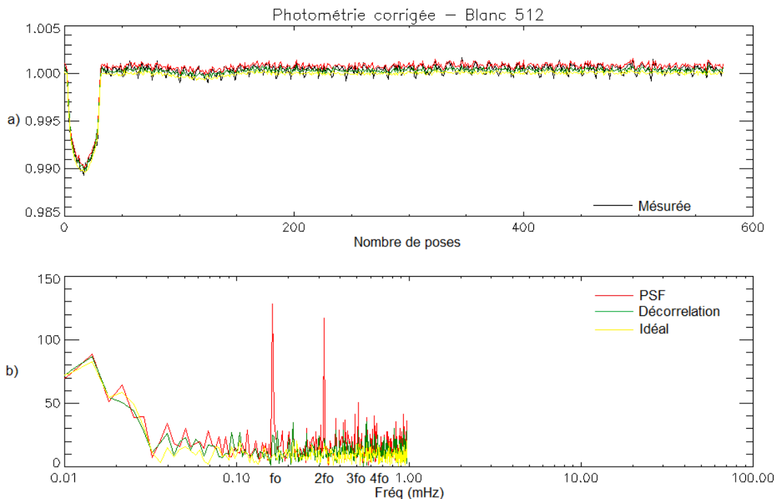
Figure 3-44: a) Photométries d'ouverture 512 sec dans le blanc corrigées du jitter comparées à l'idéale et b) les spectres de Fourier correspondant en ppm.
