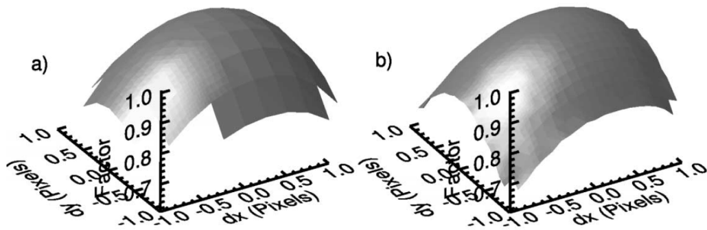
Figure 6-6 : Surfaces de correction pour HD61199 basées sur a) la PSF à haute résolution et b) la décorrélation. Les résolutions de grille sont de 0.25 pixels et 0.1 pixels, respectivement
