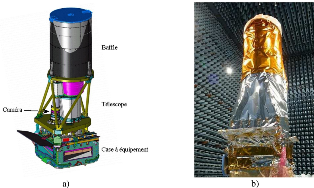
Figure 2-7 : Schéma de l'instrument a) sur lequel nous pouvons voir le télescope, la caméra et la case à équipement. A droite b) nous pouvons voir une photo de l'instrument intégré lors des essais de compatibilité électromagnétique.
