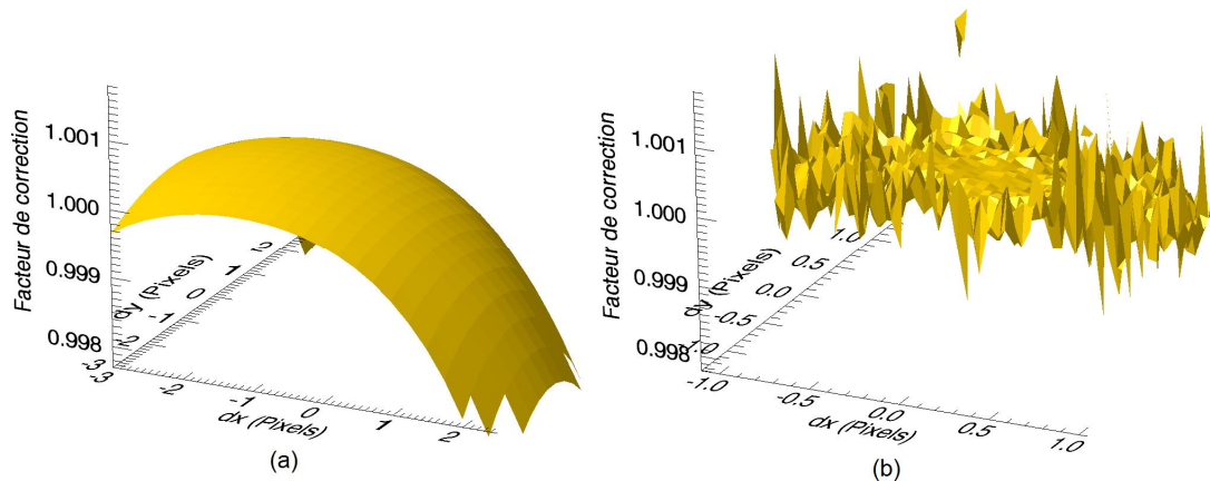
Figure 6-45 : Etoile CoRoT ID 116 - surfaces de correction basées sur a) la PSF à haute résolution et b) la décorrélation. Les résolutions de grille sont de 0.25 pixels et de 0.05 pixels, respectivement.
