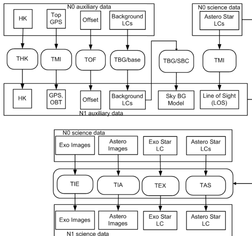
Figure 2-17 : Organigramme général de la chaîne de traitement N0 → N1 . Des données auxiliaires N1 sont produites et utilisée dans les traitements scientifiques TIE , TIA , TEX et TAS .
