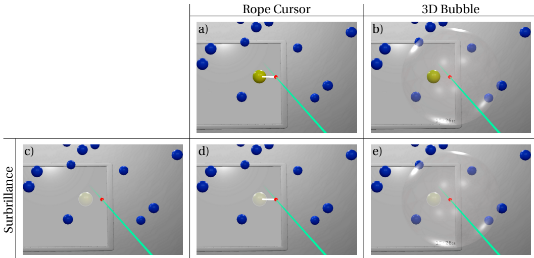
FIGURE II.3 – RayCursor avec différents retours visuels. Le curseur est rouge et le rayon est cyan. (c,d,e) Surbrillance : la cible la plus proche est mise en surbrillance. (a,d) Rope Cursor [35] : une ligne blanche relie le curseur à la cible la plus proche. (b,e) 3D Bubble [94] : une bulle 3D centrée sur le curseur, adapte son rayon pour englober la cible la plus proche.
