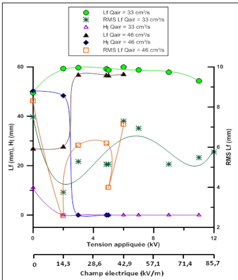
Figure III.3.14a : Evolution de L_f , H_l , \text{RMS } L_f en fonction de l'intensité du champ électrique appliqué pour un débit d'air de 33 \text{ cm}^3/\text{s} et 46 \text{ cm}^3/\text{s} , le débit de méthane étant fixé à 6 \text{ cm}^3/\text{s}
