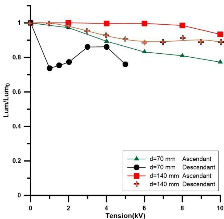
Figure III.1.12 : Comparaison entre les luminosités de flammes normalisées, dans les cas champs ascendant et descendant, en fonction de la tension électrique pour deux distances inter-électrodes. Q CH 4 =4,5 cm 3 /s
