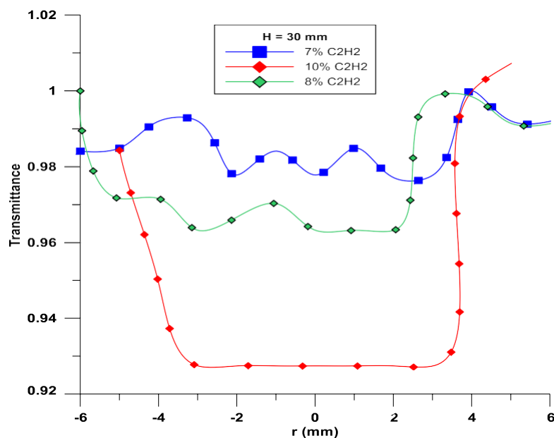
Figure IV.8 : Evolution de la transmittance à H=30 \text{ mm} suivant r(\text{mm}) pour différents pourcentages d'acétylène. Le mélange méthane/acétylène a un débit fixe de 4,5 \text{ cm}^3 \cdot \text{s}^{-1}
