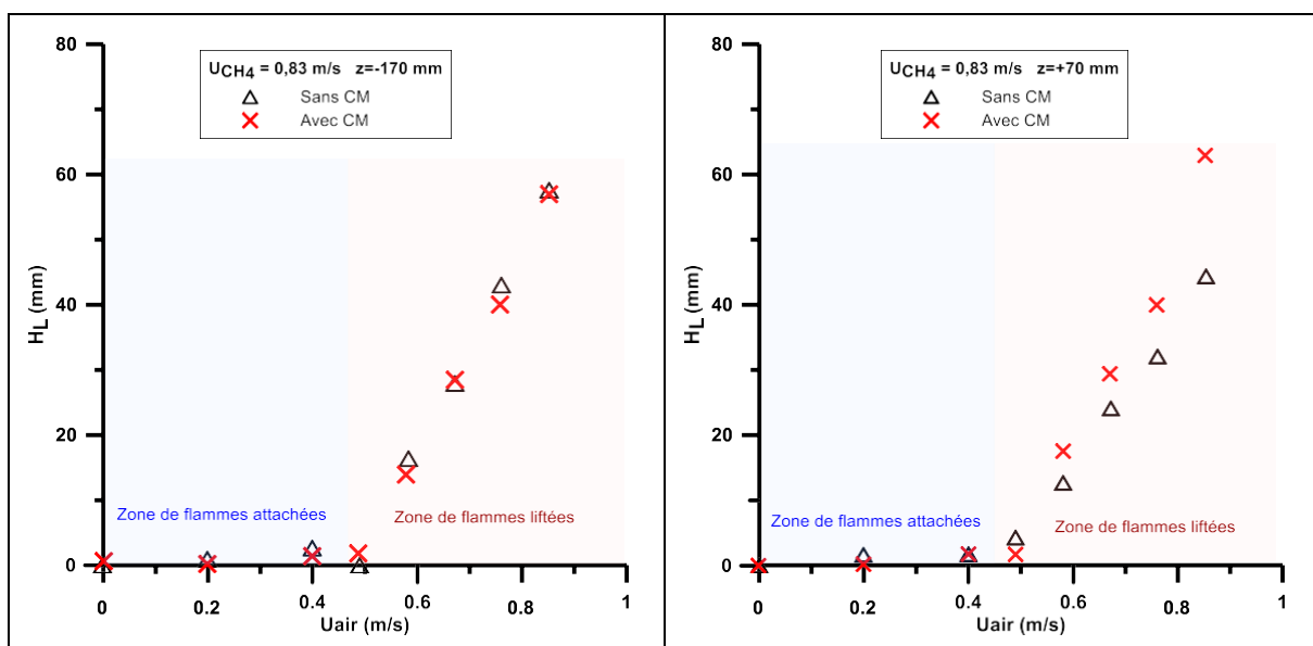
Figure II.10 : Hauteur de décrochage pour les deux positions du brûleur z=70 mm et z= -170 mm
