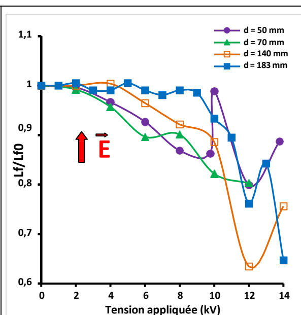
Figure III.1.3 : Evolution de la longueur de flamme normalisée en fonction de la tension électrique pour plusieurs distances inter électrodes (Champ Ascendant). Q_{CH_4}=4,5 cm 3 /s
