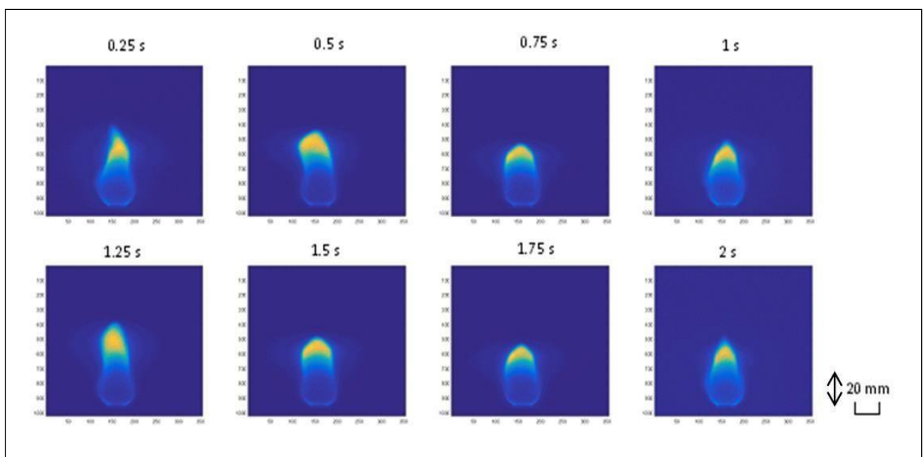
Figure III.3.10 : Images de chimiluminescence du CH* d'une flamme de méthane décrochée du brûleur avec une instabilité de flickering pour un débit de méthane de 6 \text{ cm}^3/\text{s} , un débit d'air de 33 \text{ cm}^3/\text{s} à 0 \text{ kV/m}
