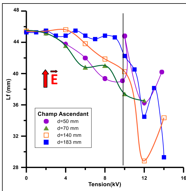
Figure III.1.2 : Evolution de la longueur de flamme en fonction de la tension électrique pour plusieurs distances inter électrodes (Champ Ascendant). Q_{CH_4}=4,5 cm 3 /s
