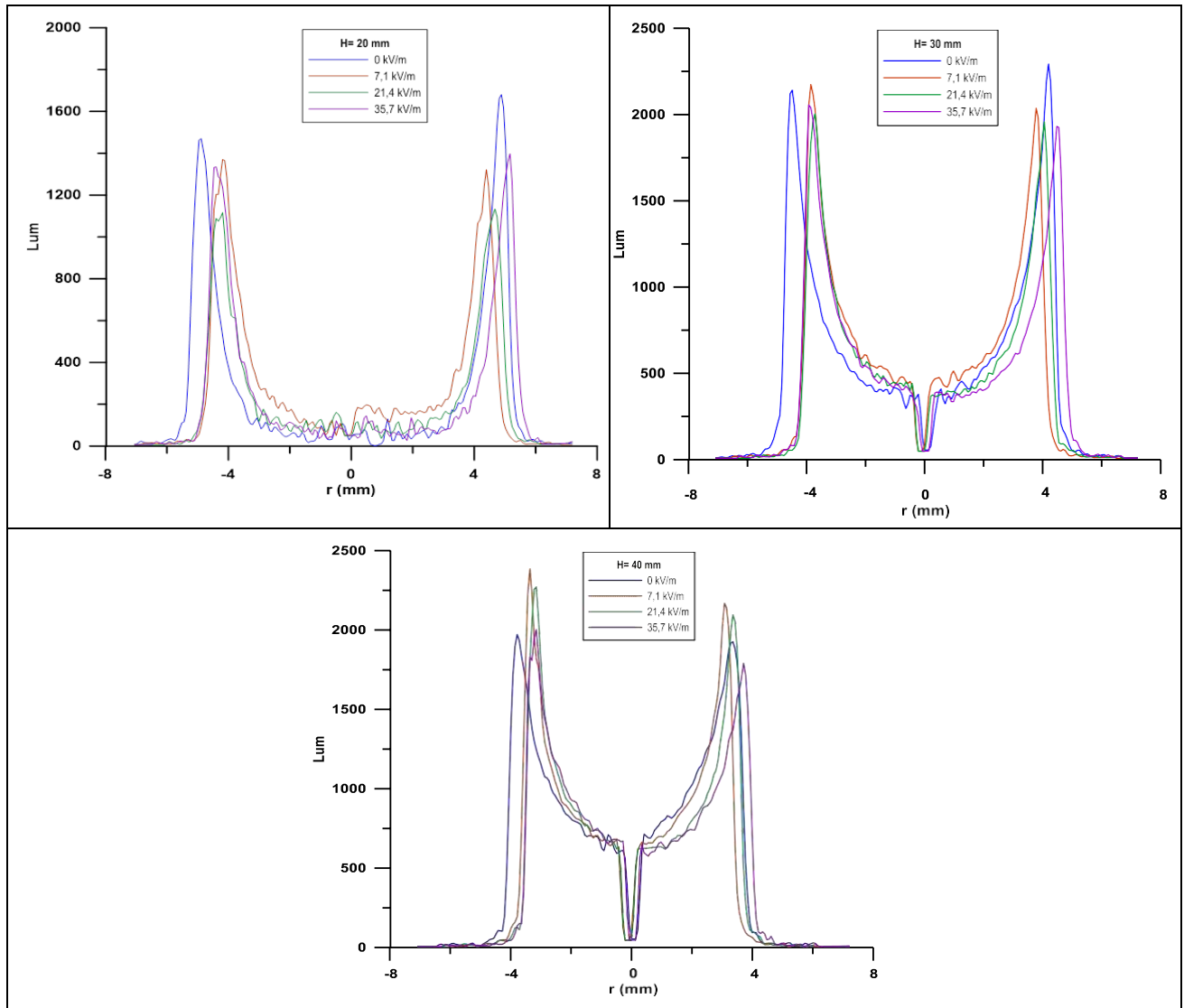
Figure IV.14 : Distribution de la luminosité en fonction du rayon de la flamme à différentes intensités de champs électriques pour trois hauteurs H=20, 30 et 40 mm.
