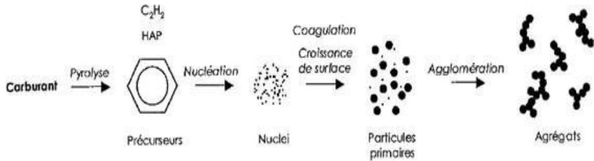
Figure I.14 : Processus chimique amenant aux agrégats de suies
