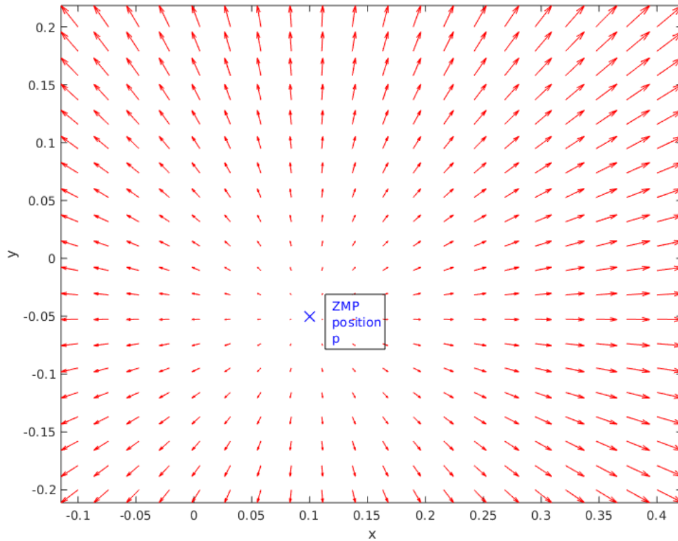
FIGURE 1.6 – Cette figure illustre la valeur de l'accélération horizontale du COM ( \ddot{x}, \ddot{y} ) pour chaque position de COM, relativement à la position du ZMP. L'effet répulseur du ZMP est ici mis en évidence. Attention, le champ de vecteurs représenté est un champ de force et non un portrait de phase, la trajectoire du COM ne sera pas parallèle aux vecteurs si elle a une vitesse initiale non nulle.
