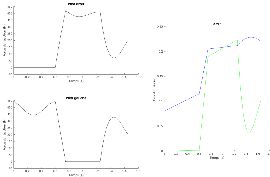
FIGURE 5.12 – Répartition de la force de réaction verticale entre le pied gauche et le pied droit pendant la phase d'arrêt, et lien avec la trajectoire du ZMP (coordonnée X en bleu et Y en vert).
