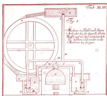
Fig. 163. Machine à vapeur de Papin
