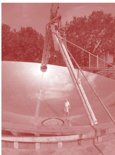
Fig. 221. Le cuisinier solaire de la cantine d'Auroville
