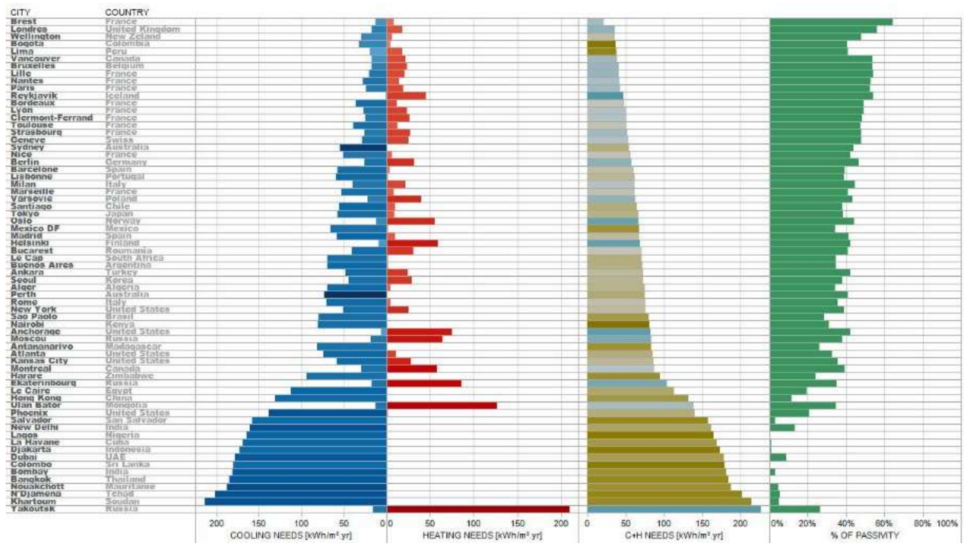
Fig. 405. Histogrammes climatiques. En bleu et en kilowattheures utiles de froid par mètre-carré et par an. En rouge et en kilowattheures utiles de chaleur par mètre-carré et par an. Résultats du ClimElioth, traités sous le logiciel Tableau.
