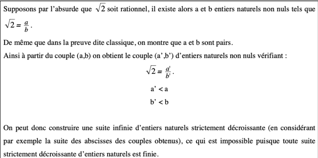
Figure 2-1: Preuve par descente infinie (Battie V. , 2003, p. 233)
