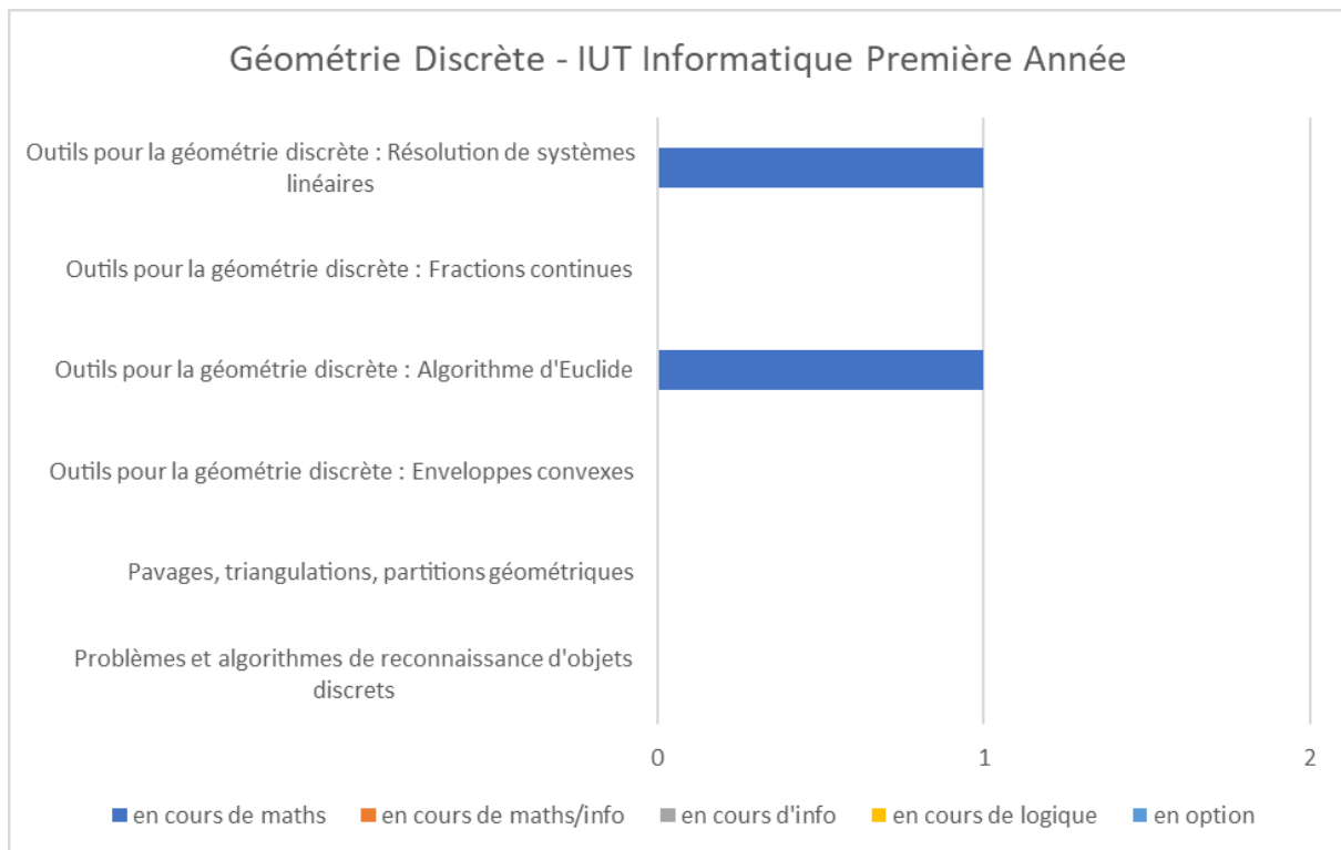
Annexe-Figure 77: Géométrie Discrète - IUT Informatique Première Année – France
