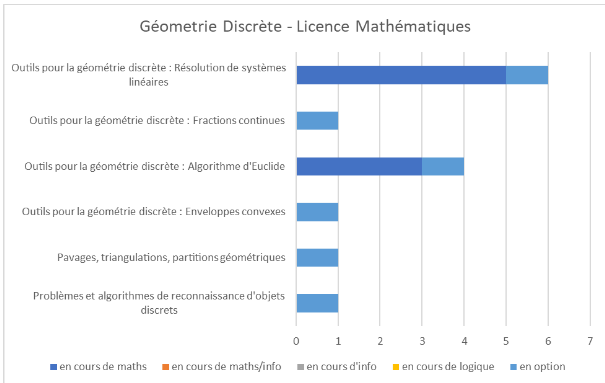
Annexe-Figure 57: Géométrie Discrète - Licence Mathématiques – France
