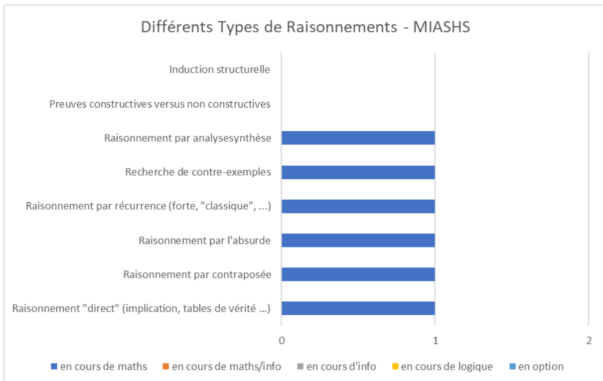
Annexe-Figure 34: Différents Types de Raisonnements - MIASHS – France
