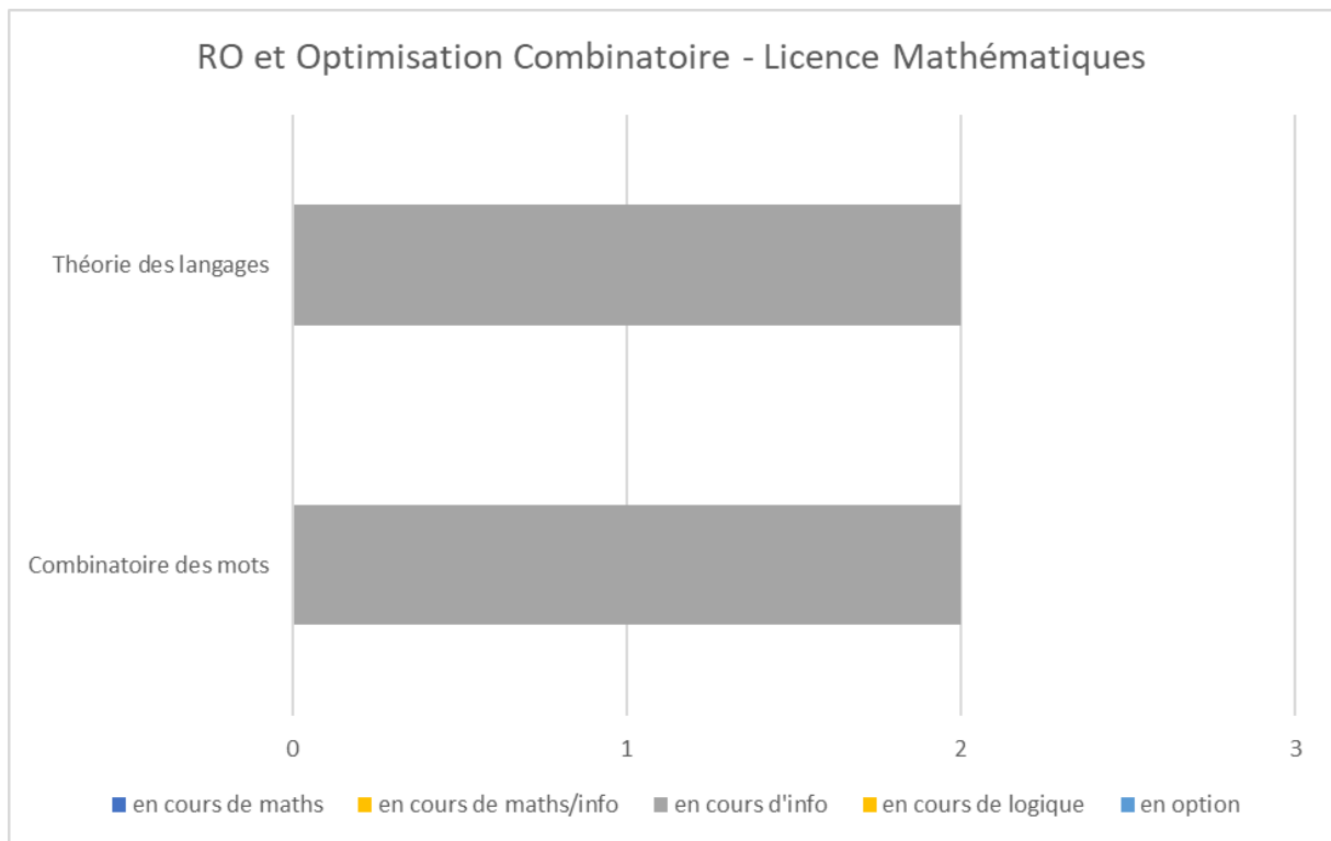
Annexe-Figure 7: RO et Optimisation Combinatoire - Licence Mathématiques – Liban
