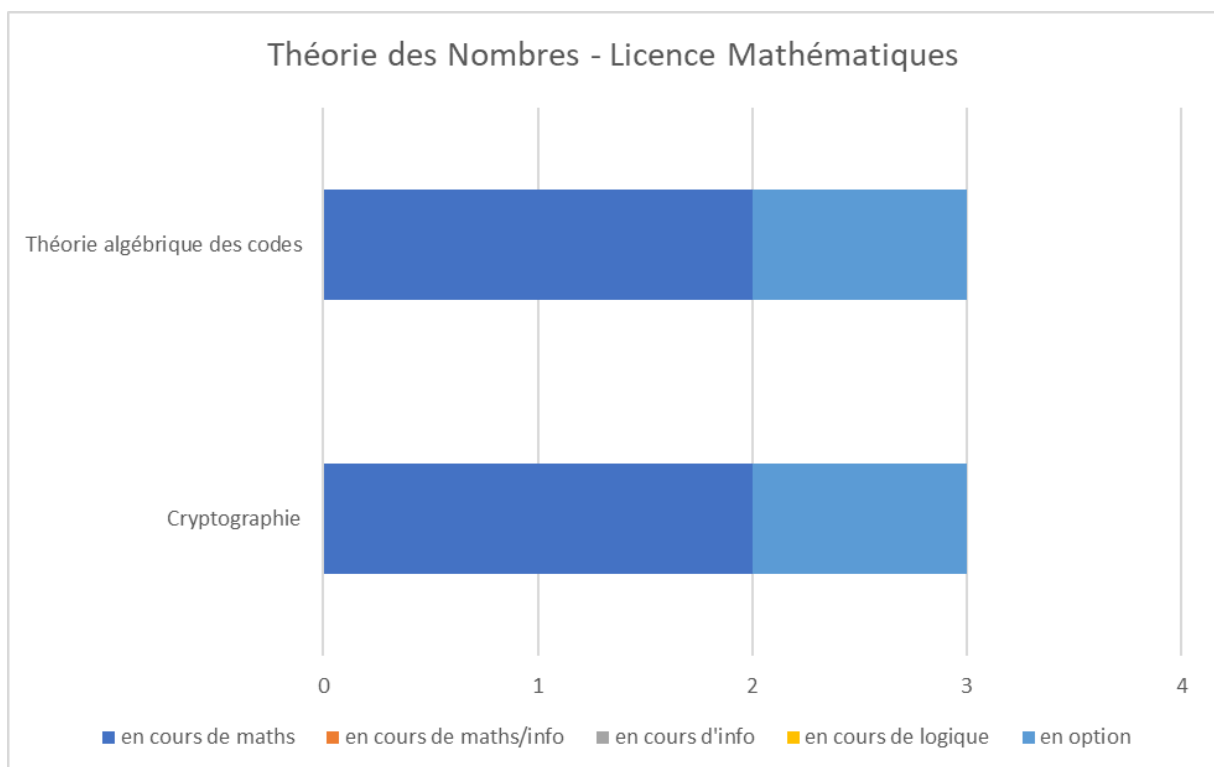
Annexe-Figure 8: Théorie des Nombres - Licence Mathématiques – Liban
