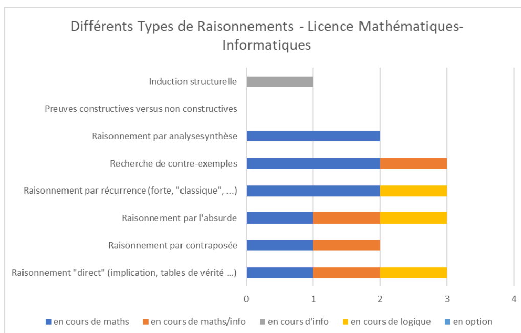
Figure 3-17: Différents Types de Raisonnements - Licence Mathématiques-Informatique – France
