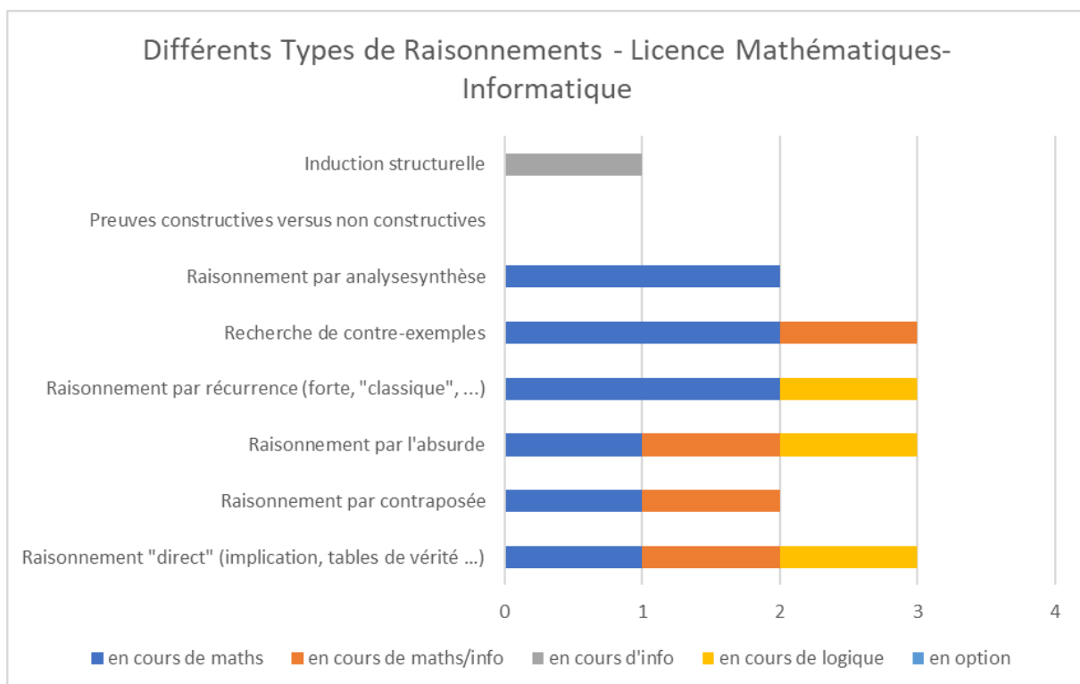
Annexe-Figure 38: Différents Types de Raisonnements - Licence Mathématiques-Informatique – France
