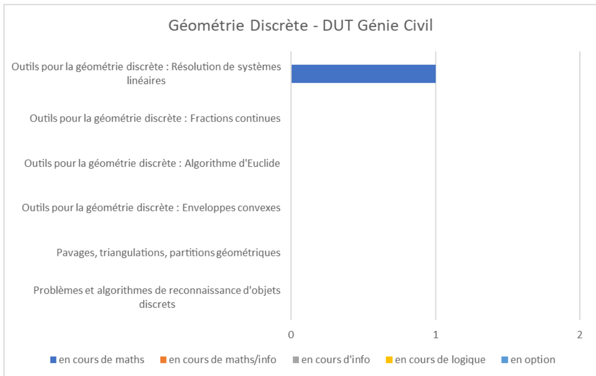
Annexe-Figure 97: Géométrie Discrète - DUT Génie Civil - France
