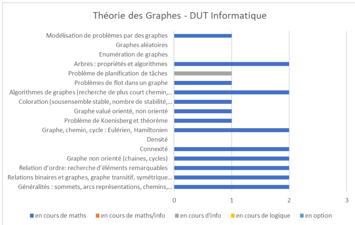
Annexe-Figure 89: Théorie des Graphes - DUT Informatique – France
