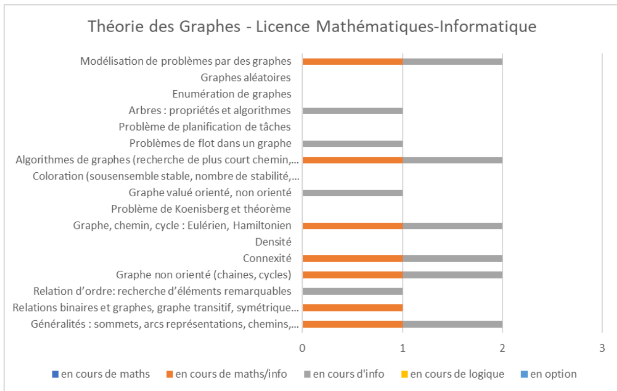
Annexe-Figure 43: Théorie des Graphes - Licence Mathématiques-Informatique – France
