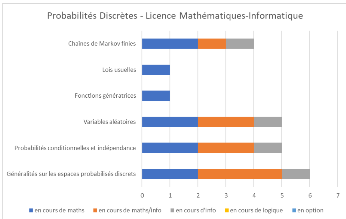
Annexe-Figure 20: Probabilités Discrètes - Licence Mathématiques-Informatique – Liban
