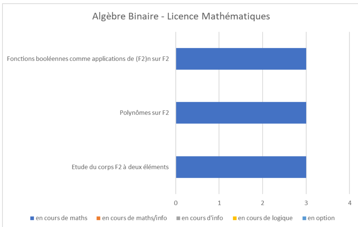
Annexe-Figure 10: Algèbre Binaire - Licence Mathématiques – Liban
