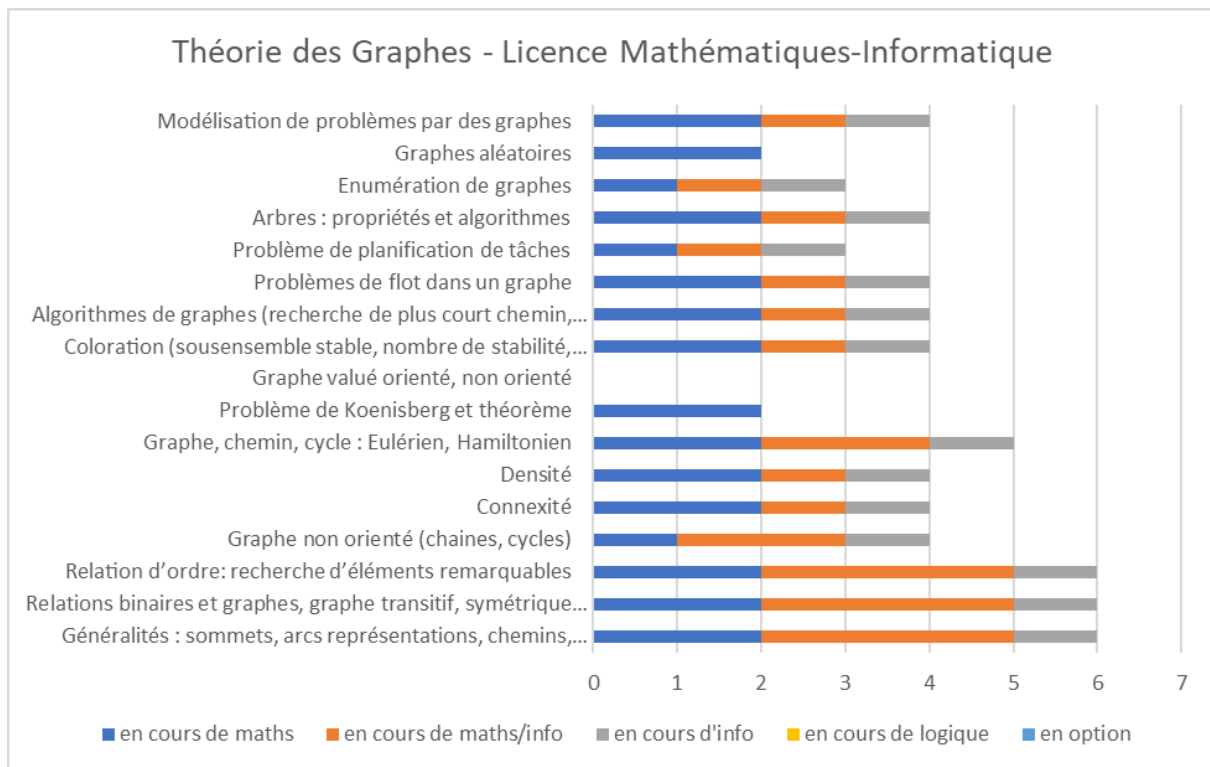
Annexe-Figure 17: Théorie des Graphes - Licence Mathématiques-Informatique – Liban
