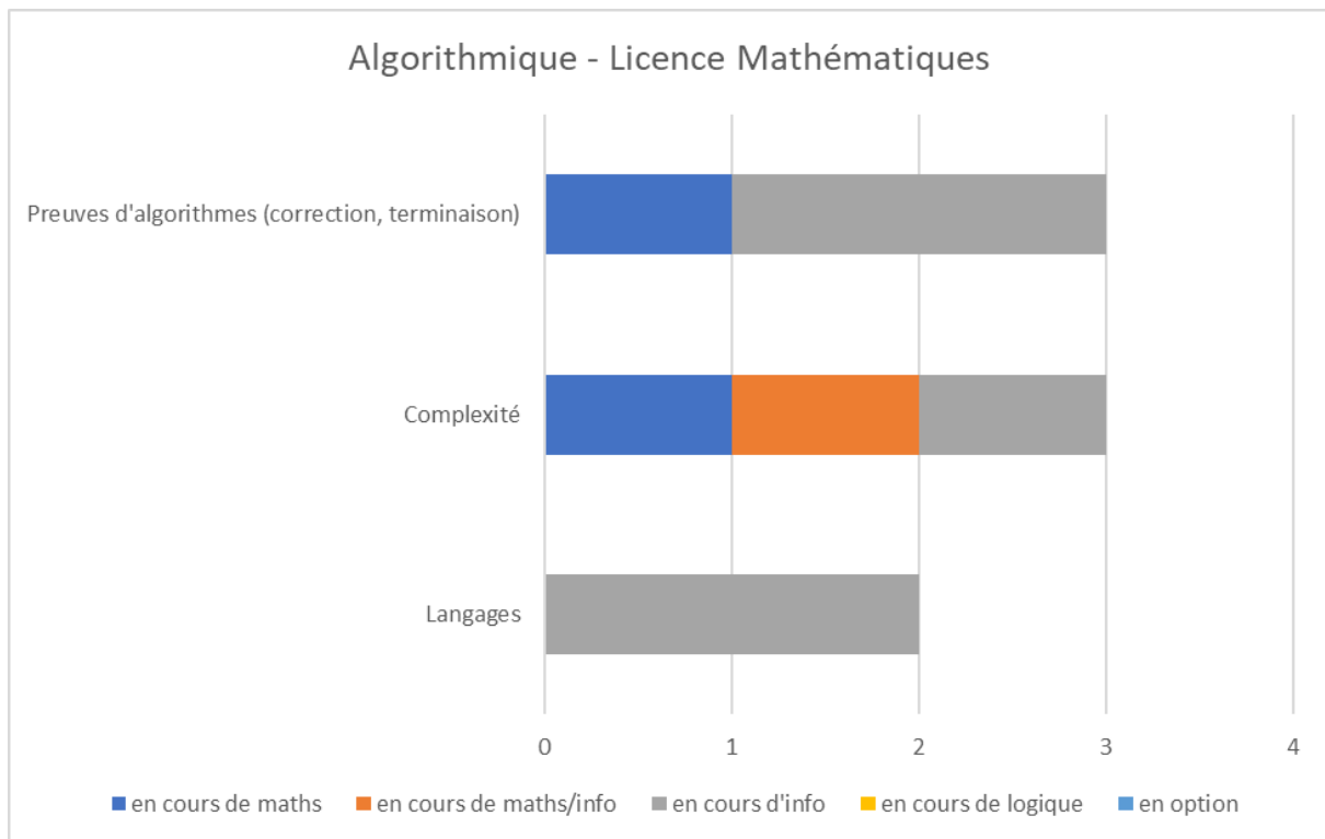
Annexe-Figure 5: Algorithmique - Licence Mathématiques – Liban
