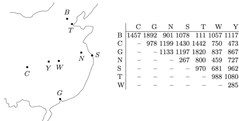
Figure 3-67: Exemple arbres couvrant de poids minimum (Bondy & Murty, 2008)
