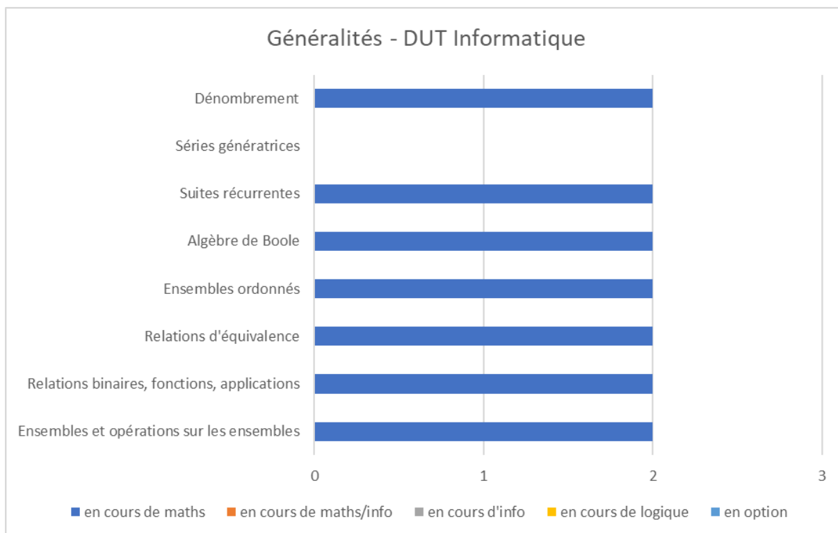
Annexe-Figure 87: Généralités - DUT Informatique – France
