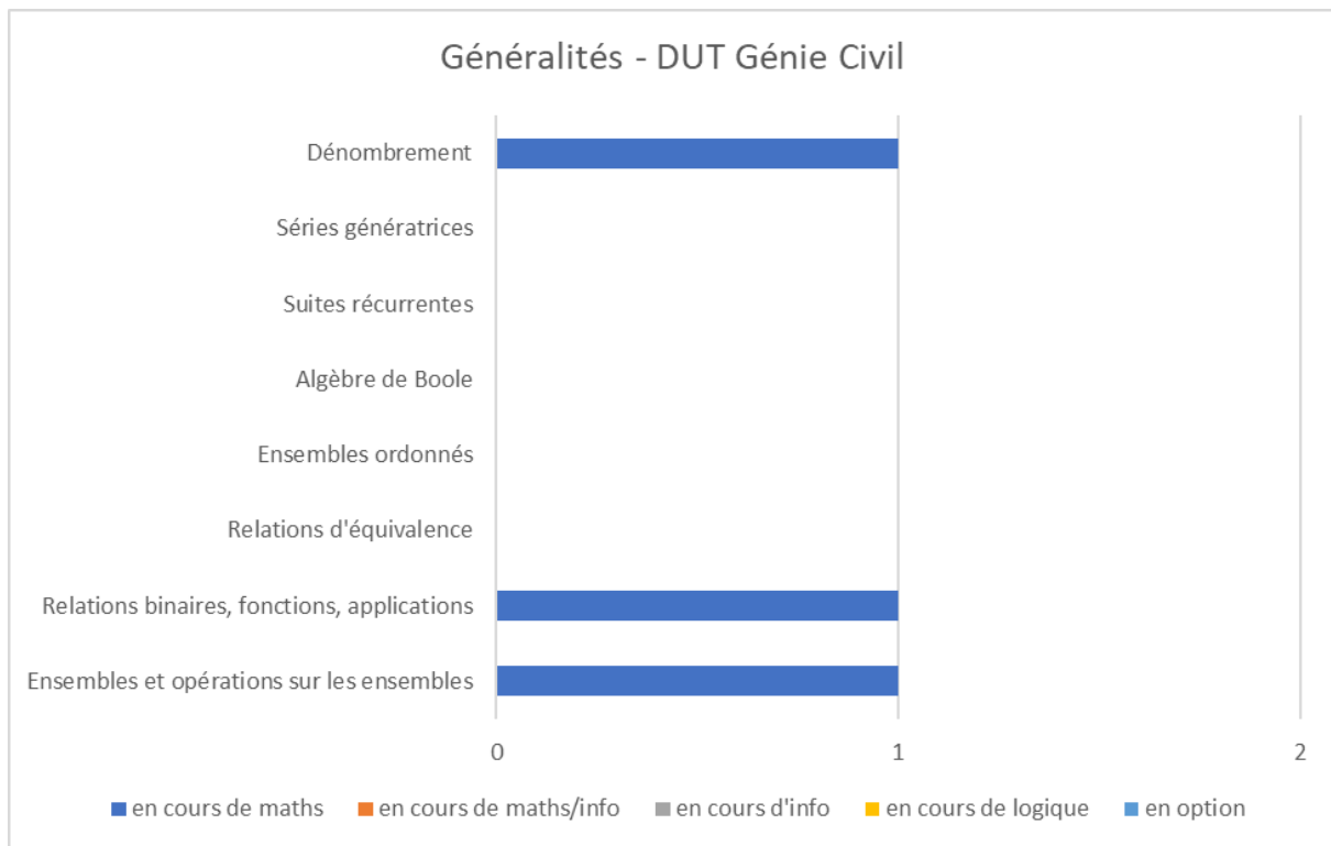
Annexe-Figure 95: Généralités - DUT Génie Civil – France
