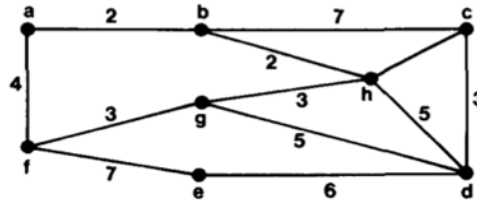
Figure 3-68: Exemple sur arbre couvrant de poids minimum (Hartsfield & Ringel, 1994)
