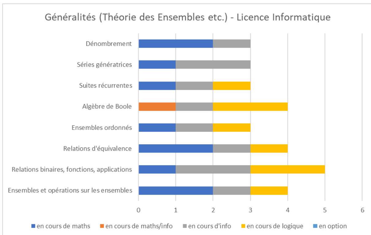
Annexe-Figure 26: Généralités (Théorie des Ensembles etc.) - Licence Informatique – Liban
