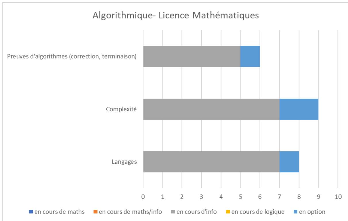
Annexe-Figure 51: Algorithmique- Licence Mathématiques – France
