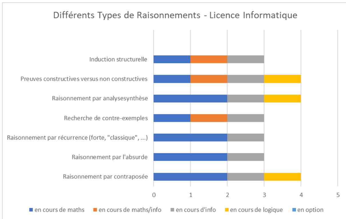
Annexe-Figure 23: Différents Types de Raisonnements - Licence Informatique – Liban
