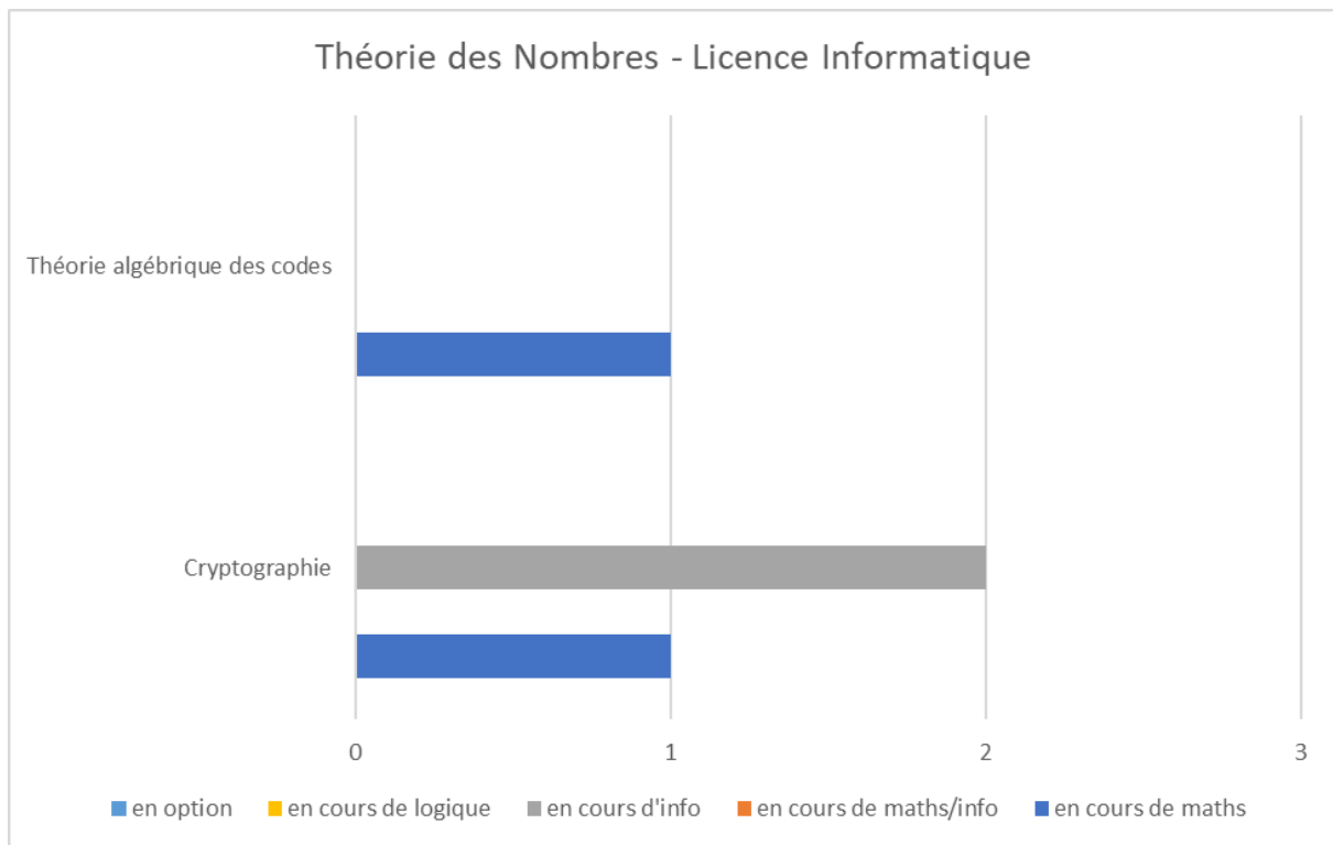
Annexe-Figure 65: Théorie des Nombres - Licence Informatique – France
