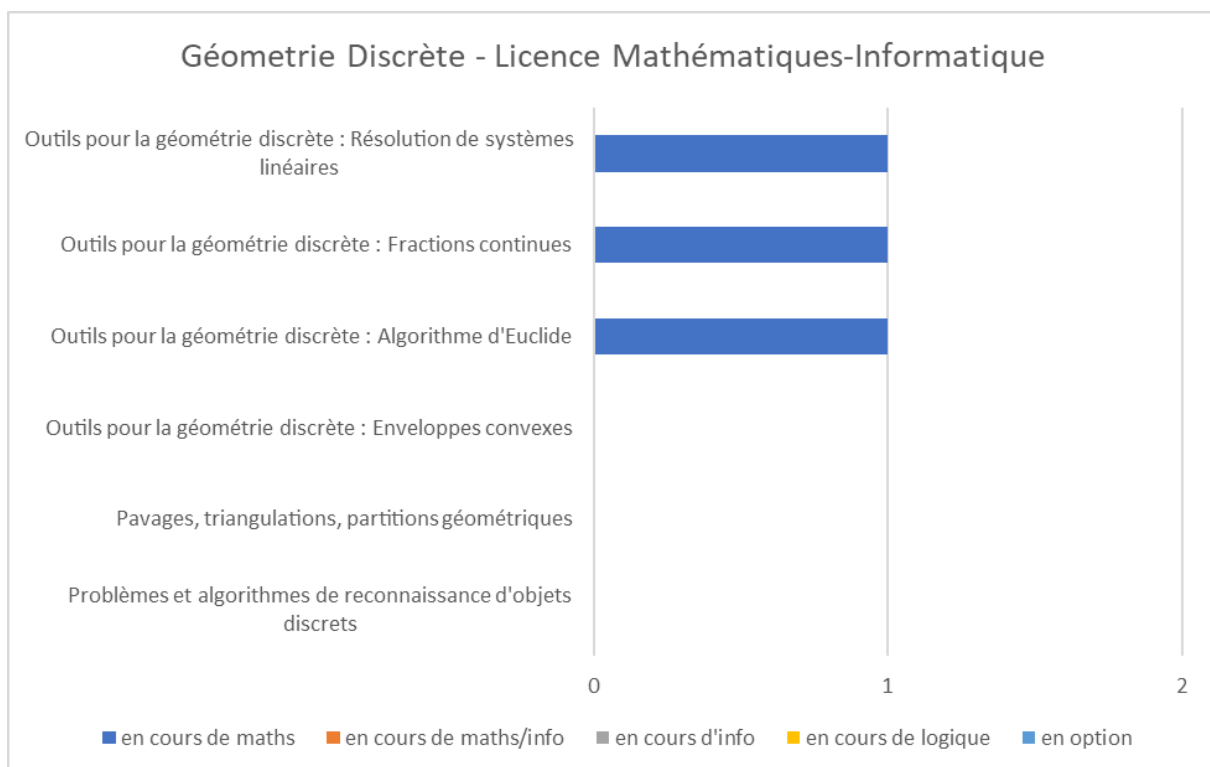
Annexe-Figure 46: Géométrie Discrète - Licence Mathématiques-Informatique - France
