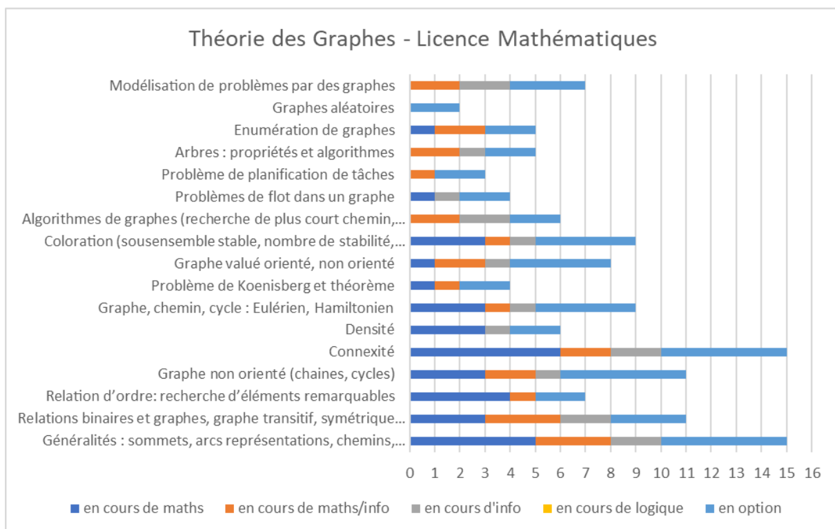
Annexe-Figure 52: Théorie des Graphes - Licence Mathématiques – France
