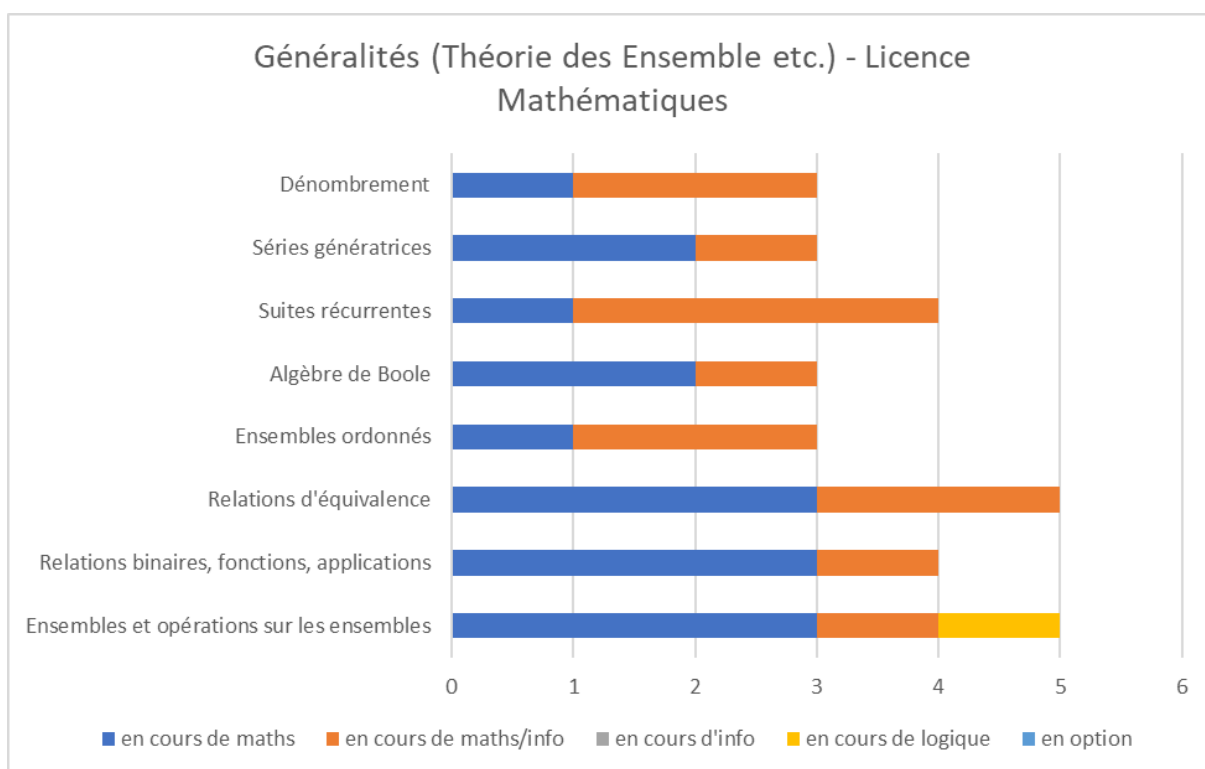
Annexe-Figure 4: Généralités (Théorie des Ensemble etc.) - Licence Mathématiques – Liban
