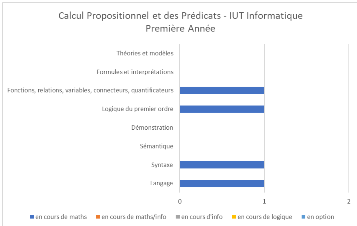
Annexe-Figure 69: Calcul Propositionnel et des Prédicats - IUT Informatique Première Année – France
