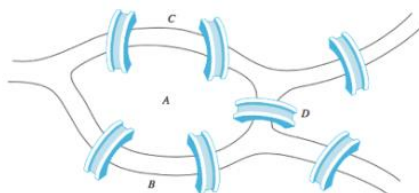
Figure 3-22: Les sept ponts du Königsberg
