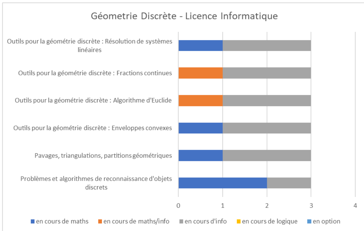
Annexe-Figure 33: Géométrie Discrète - Licence Informatique - Liban
