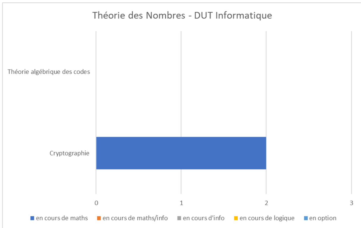
Annexe-Figure 91: Théorie des Nombres - DUT Informatique – France
