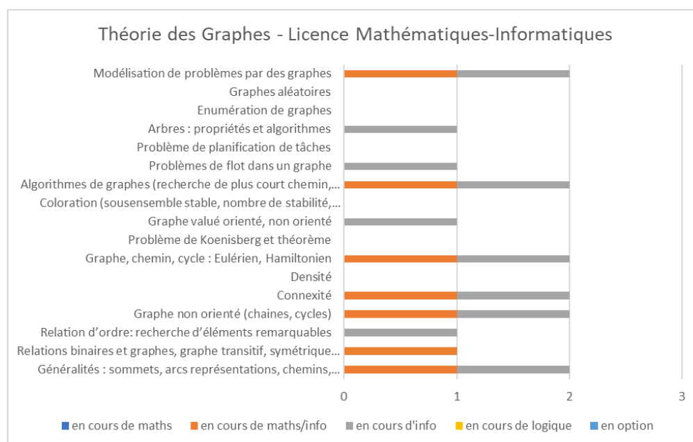
Figure 3-14: Théorie des Graphes - Licence Mathématiques-Informatique – France
