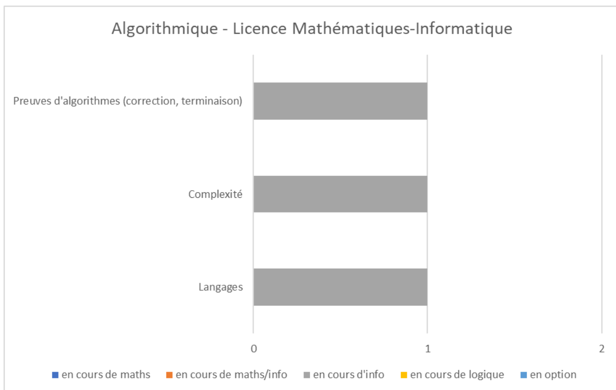
Annexe-Figure 42: Algorithmique - Licence Mathématiques-Informatique – France
