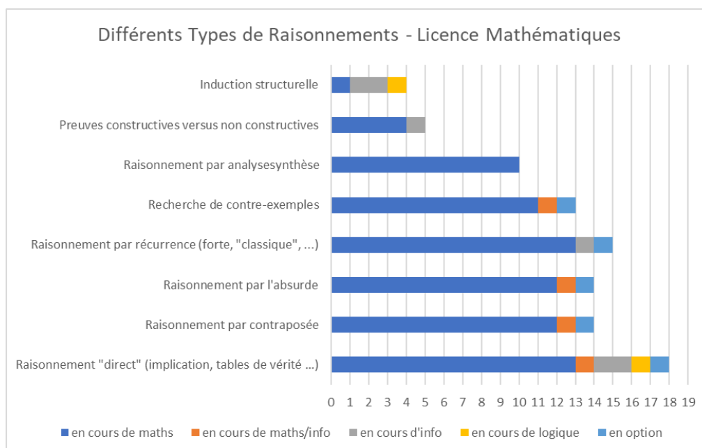
Figure 3-16: Différents Types de Raisonnements - Licence Mathématiques – France
