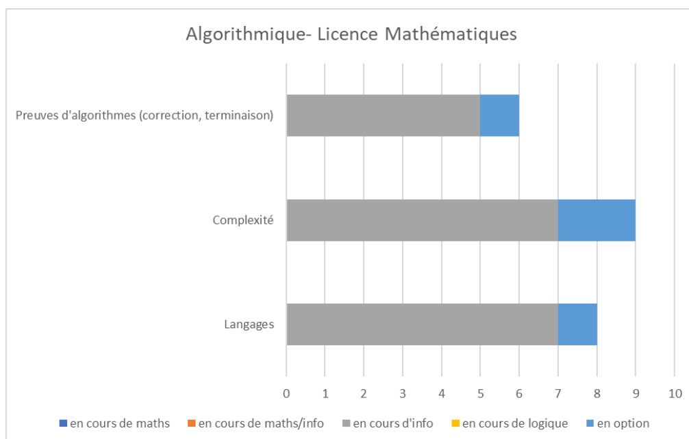
Figure 3-19: Algorithmique- Licence Mathématiques – France
