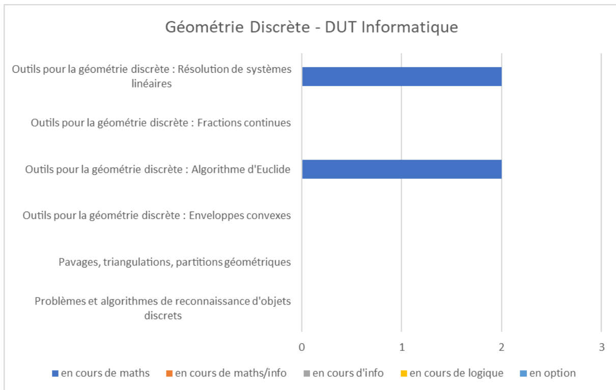
Annexe-Figure 93: Géométrie Discrète - DUT Informatique – France
