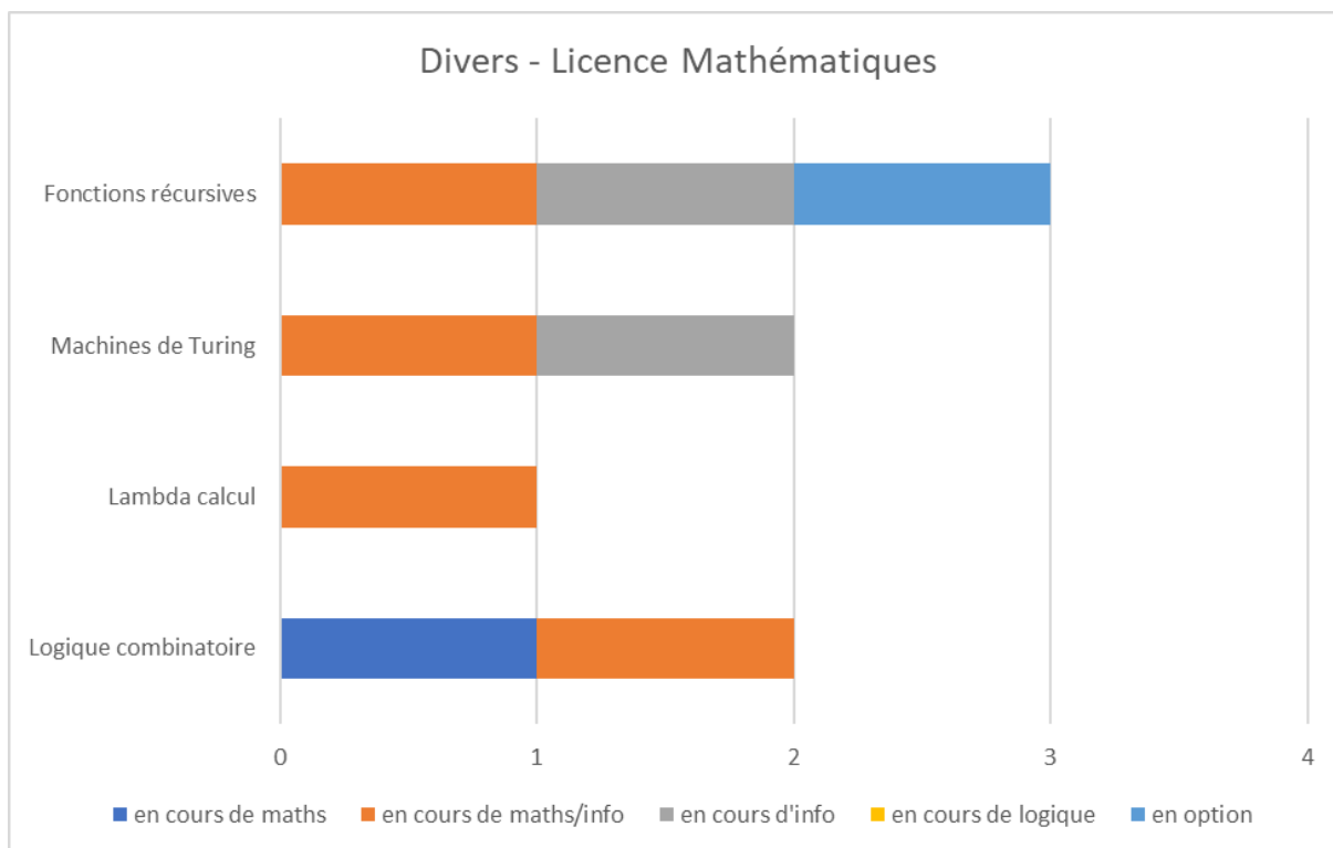
Annexe-Figure 49: Divers - Licence Mathématiques – France
