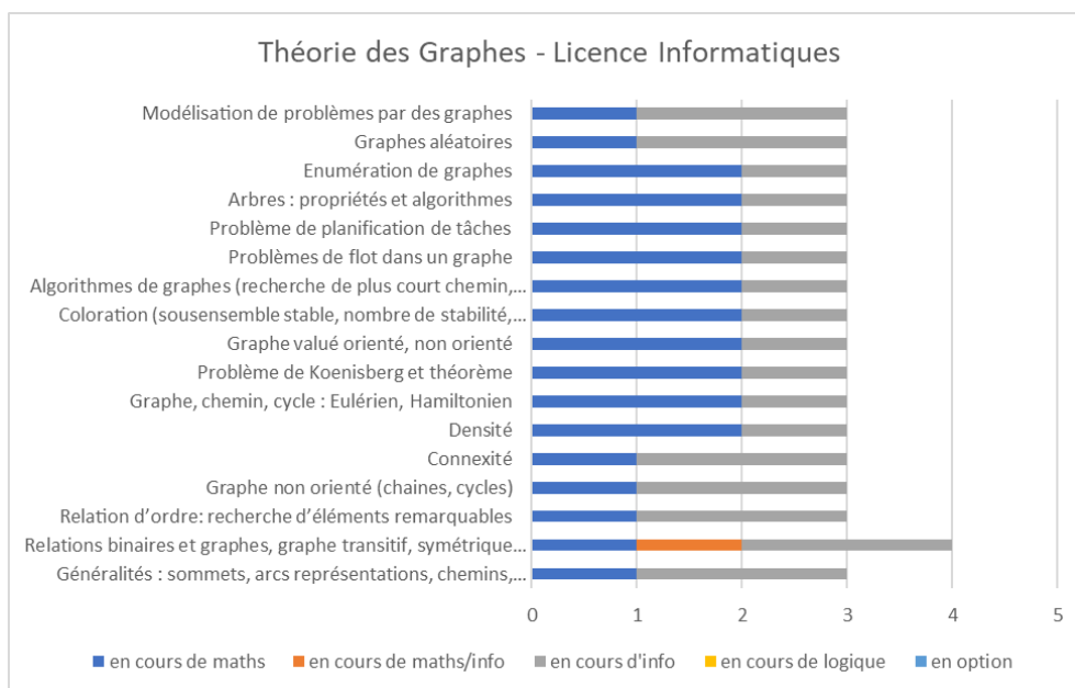
Figure 3-6: Théorie des Graphes - Licence Informatique – Liban
