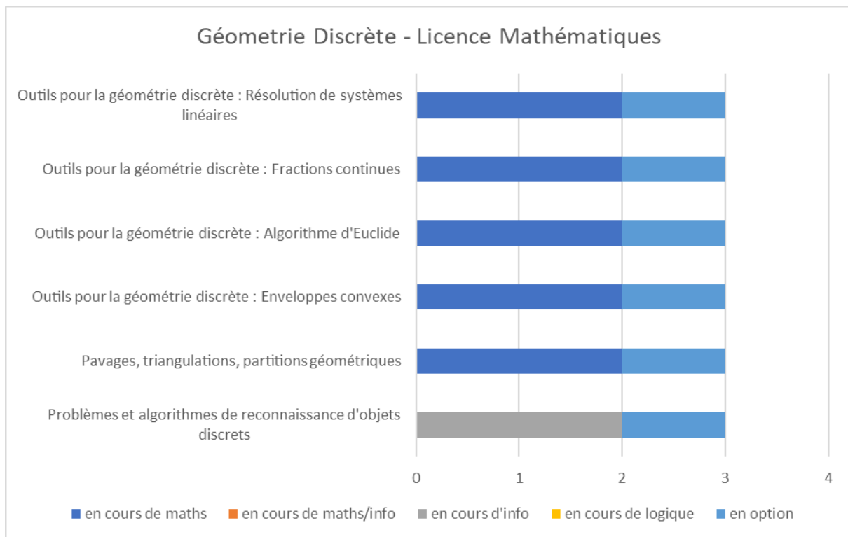
Annexe-Figure 11: Géométrie Discrète - Licence Mathématiques – Liban
