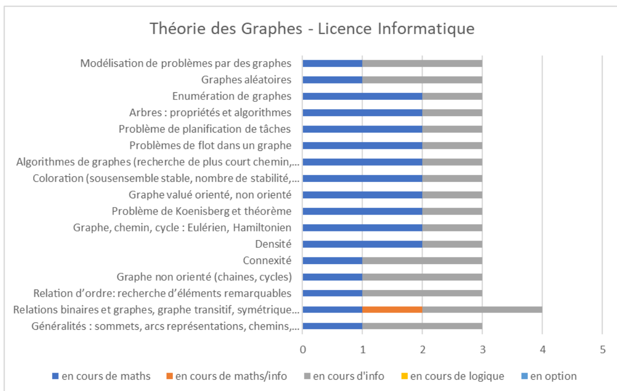
Annexe-Figure 28: Théorie des Graphes - Licence Informatique – Liban
