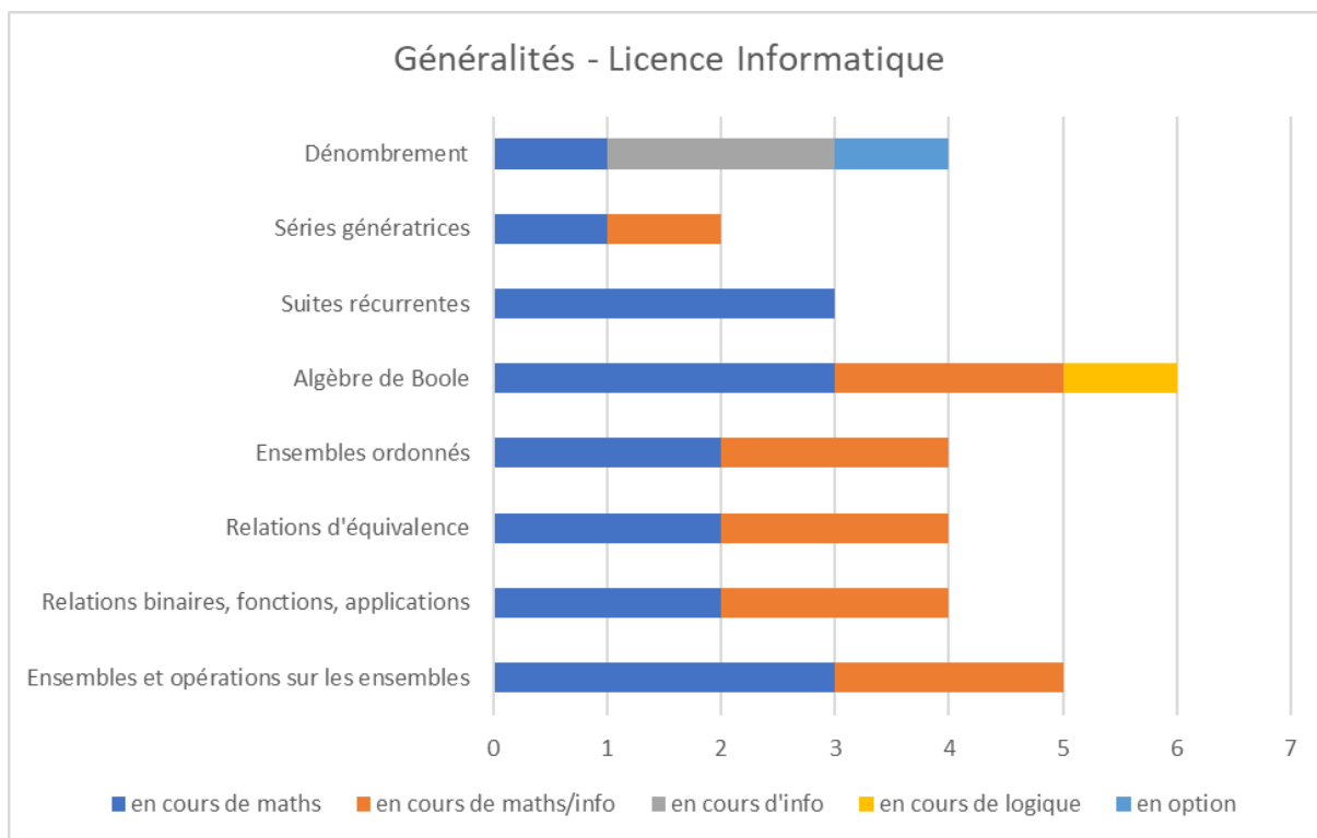
Annexe-Figure 61: Généralités - Licence Informatique – France
