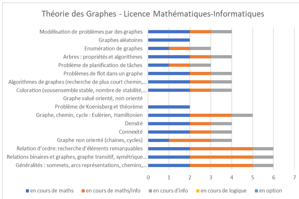
Figure 3-5: Théorie des Graphes - Licence Mathématiques-Informatique – Liban
