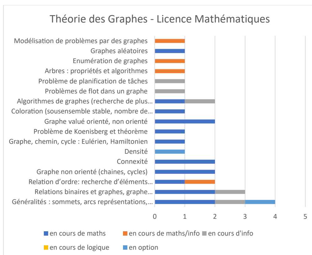
Figure 3-4: Théorie des Graphes - Licence Mathématiques – Liban
