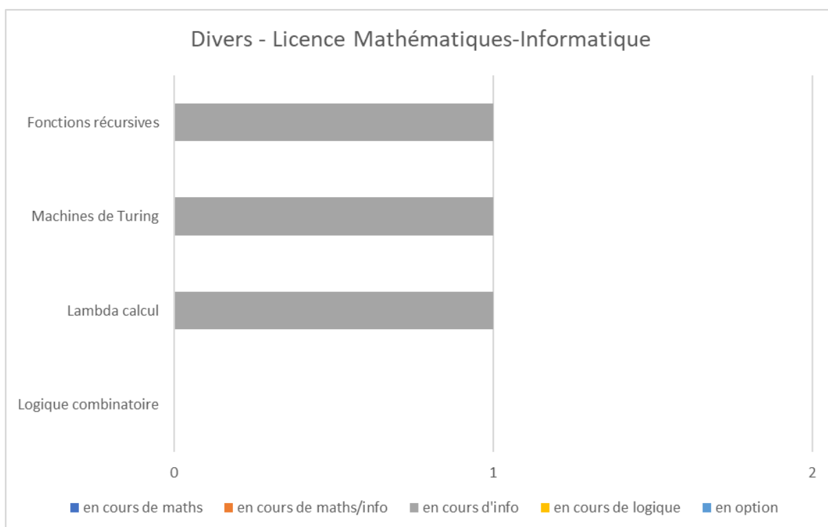
Annexe-Figure 40: Divers - Licence Mathématiques-Informatique – France
