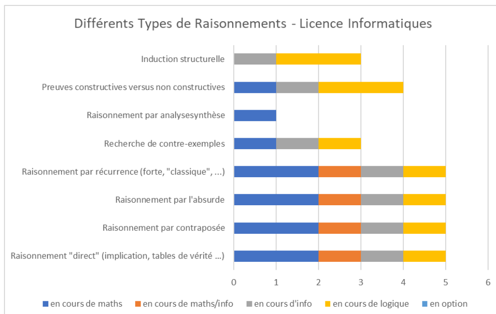
Figure 3-18: Différents Types de Raisonnements - Licence Informatique – France
