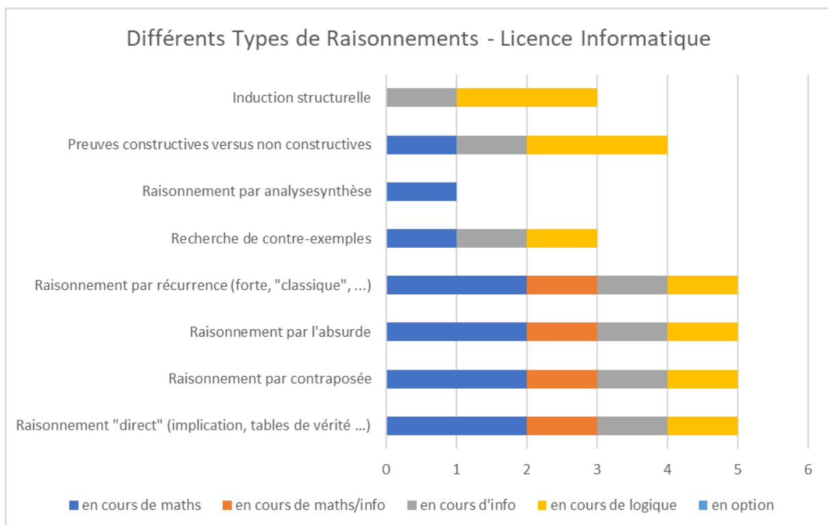
Annexe-Figure 58: Différents Types de Raisonnements - Licence Informatique – France
