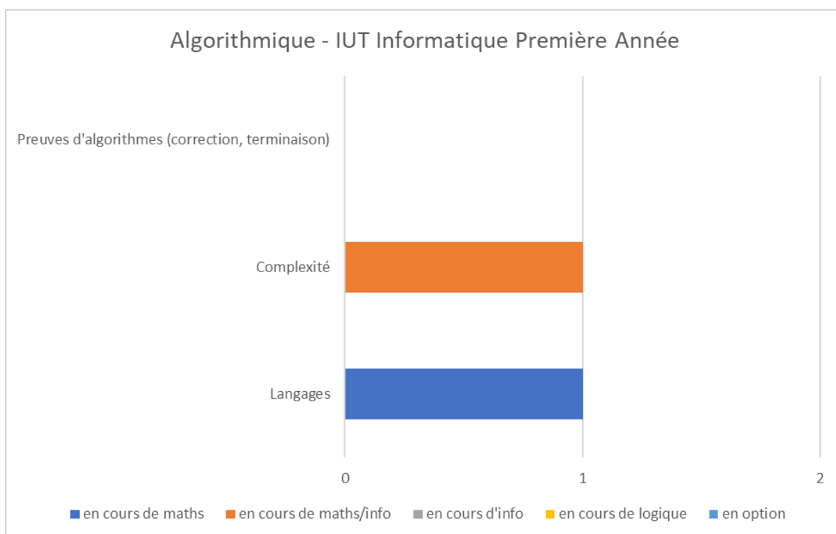
Annexe-Figure 72: Algorithmique - IUT Informatique Première Année – France
