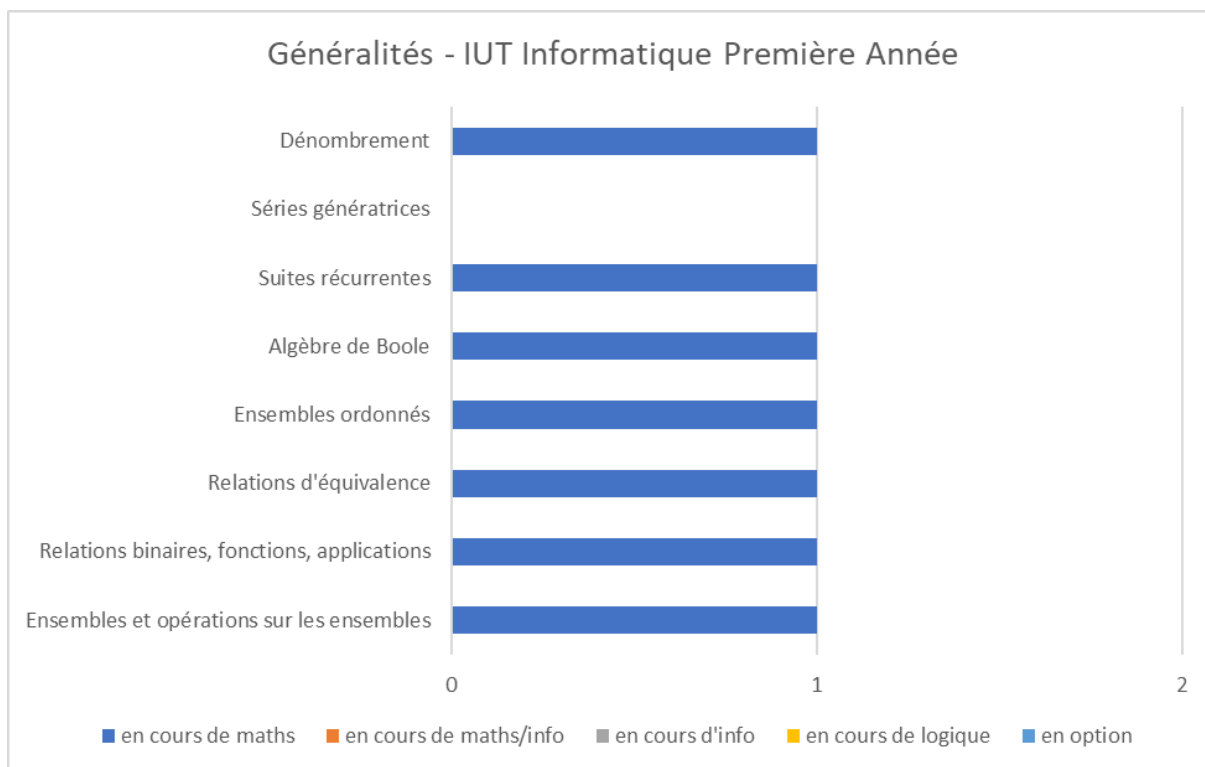
Annexe-Figure 71: Généralités - IUT Informatique Première Année – France
