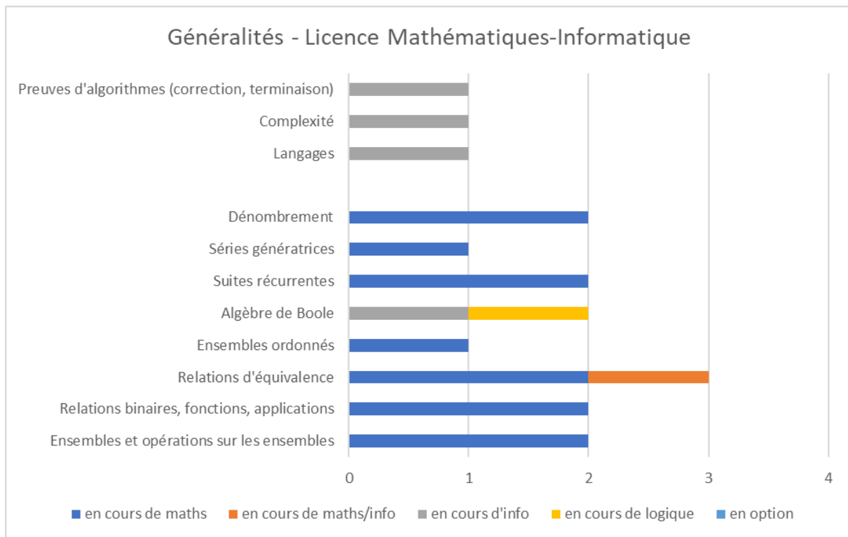
Annexe-Figure 41: Généralités - Licence Mathématiques-Informatique – France
