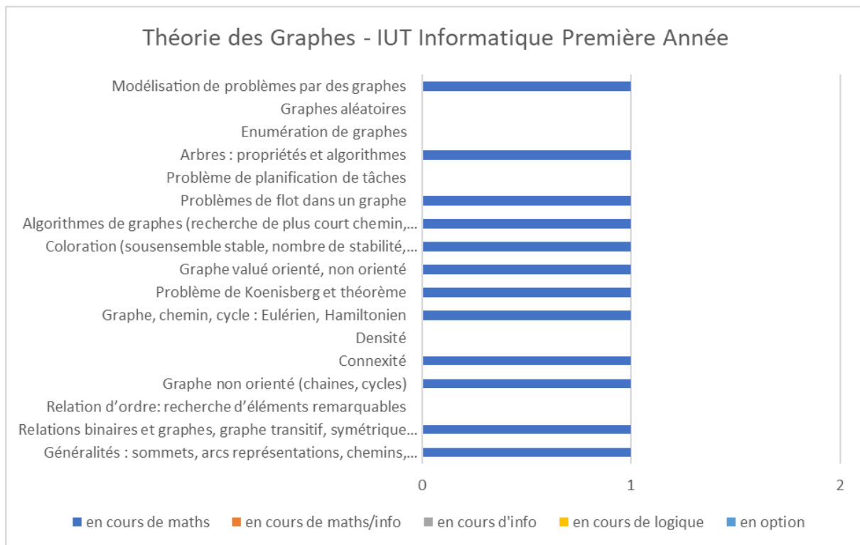
Annexe-Figure 73: Théorie des Graphes - IUT Informatique Première Année – France
