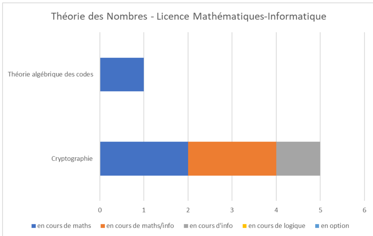
Annexe-Figure 19: Théorie des Nombres - Licence Mathématiques-Informatique – Liban
