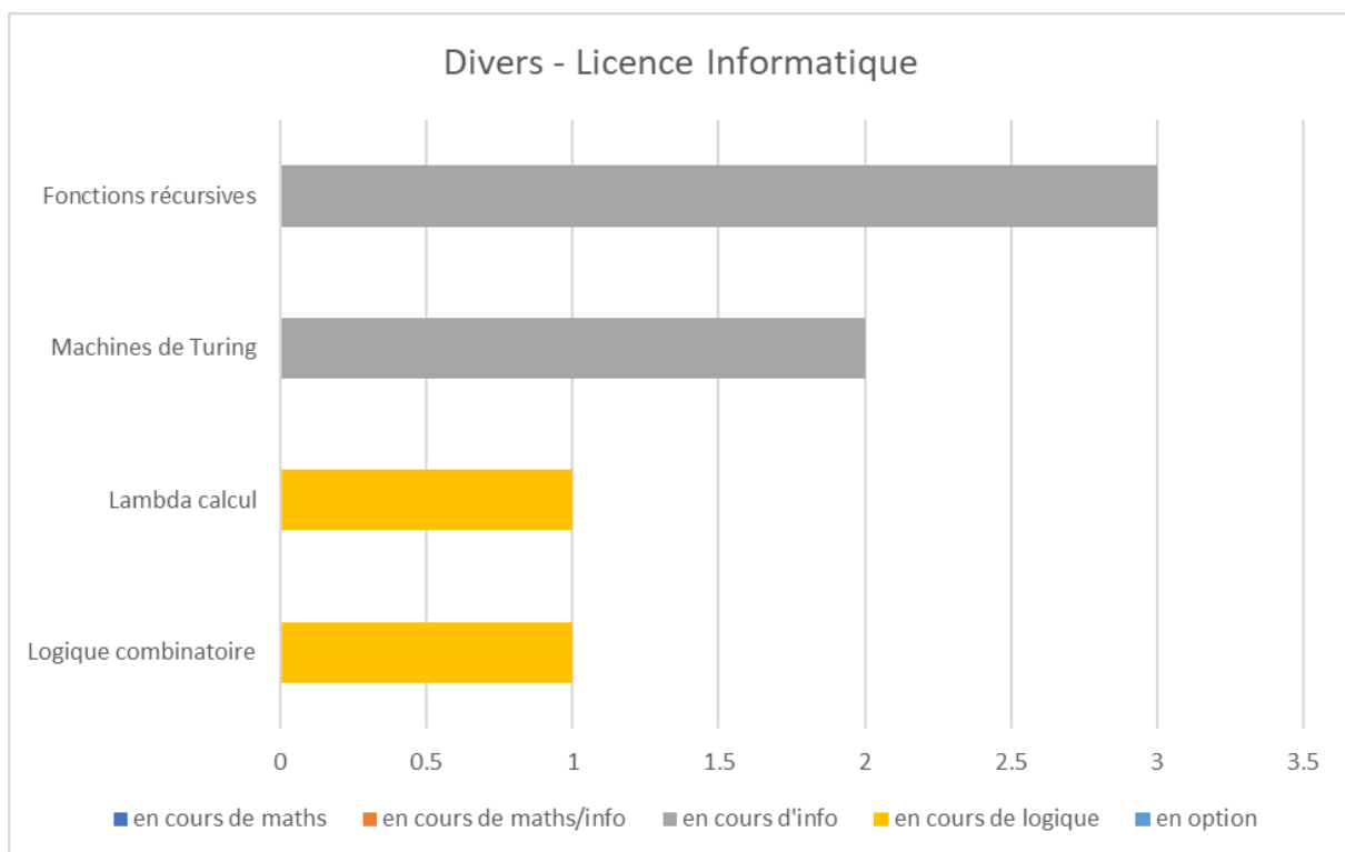
Annexe-Figure 60: Divers - Licence Informatique – France
