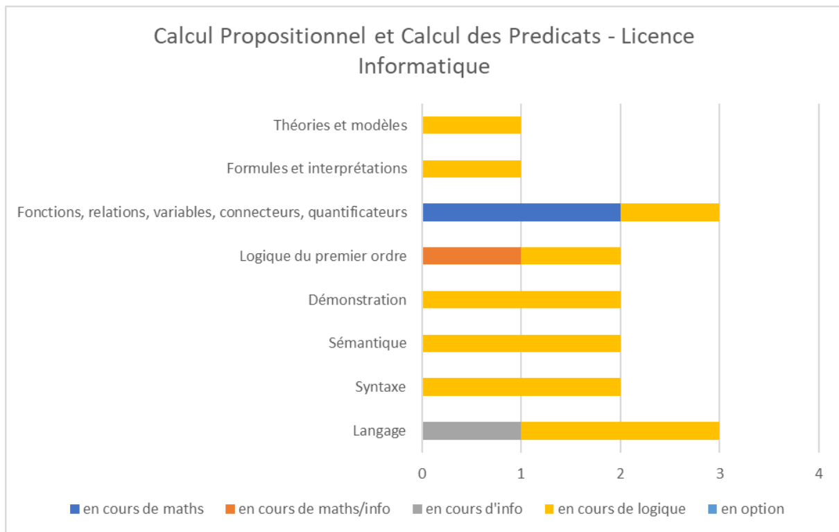
Annexe-Figure 59: Calcul Propositionnel et Calcul des Prédicats - Licence Informatique – France
