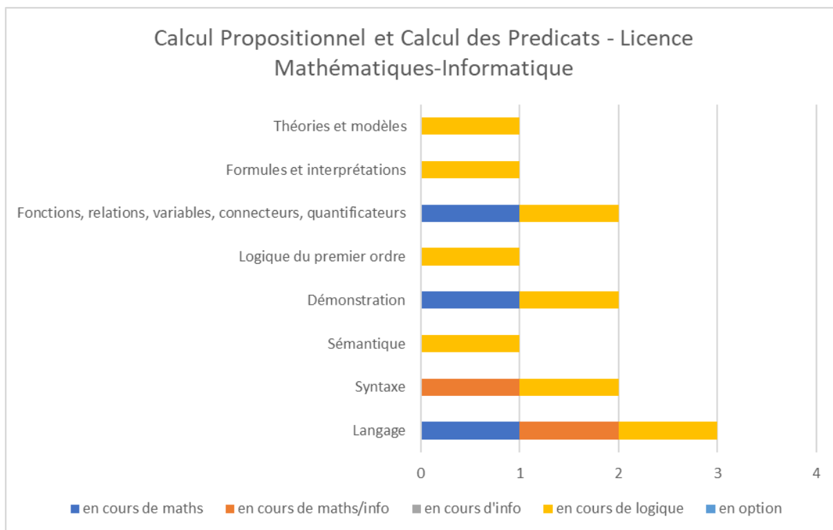
Annexe-Figure 39: Calcul Propositionnel et Calcul des Prédicats - Licence Mathématiques-Informatique – France
