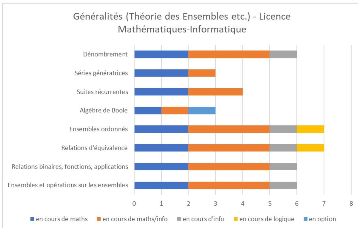
Annexe-Figure 15: Généralités (Théorie des Ensembles etc.) - Licence Mathématiques-Informatique – Liban
