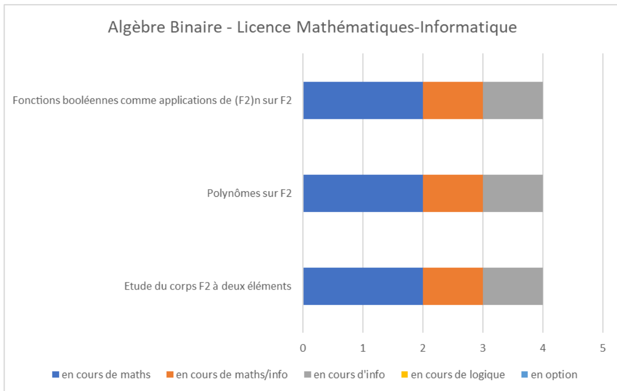
Annexe-Figure 21: Algèbre Binaire - Licence Mathématiques-Informatique – Liban
