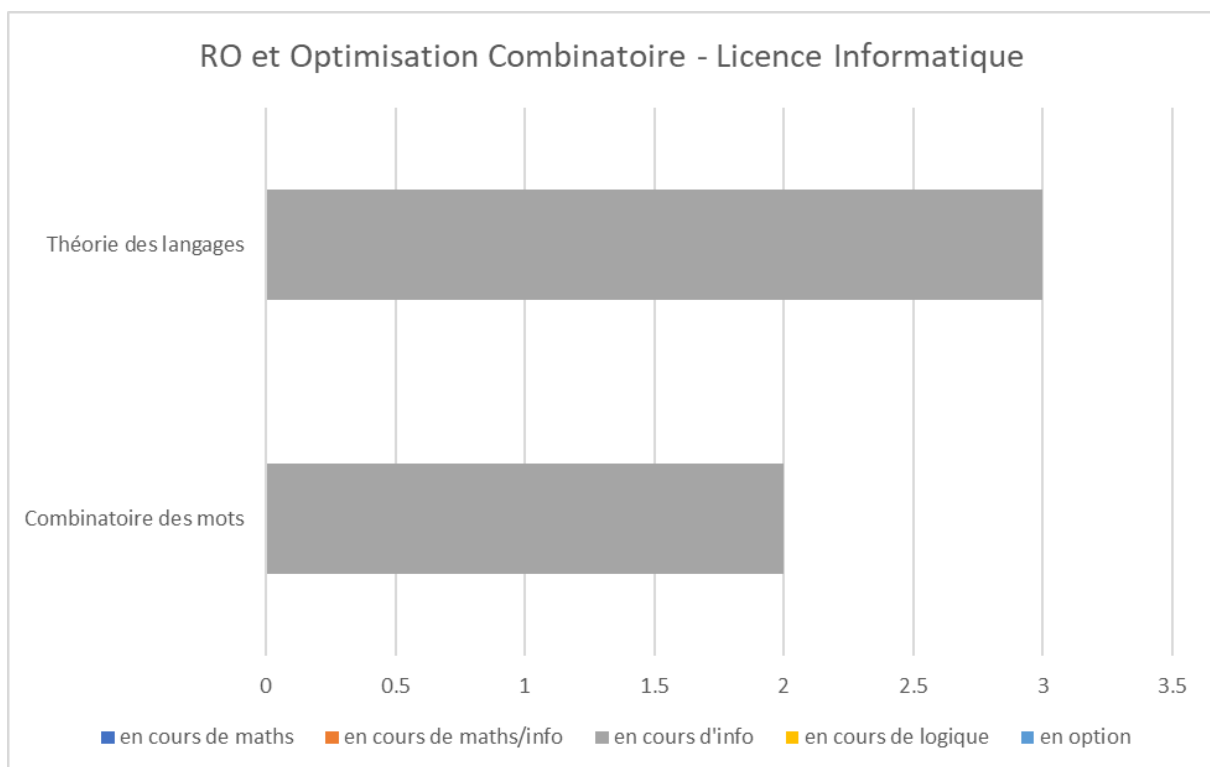
Annexe-Figure 64: RO et Optimisation Combinatoire - Licence Informatique – France
