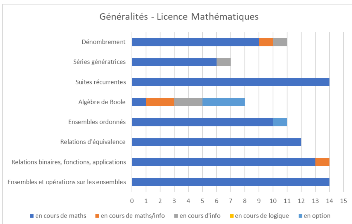
Annexe-Figure 50: Généralités - Licence Mathématiques – France
