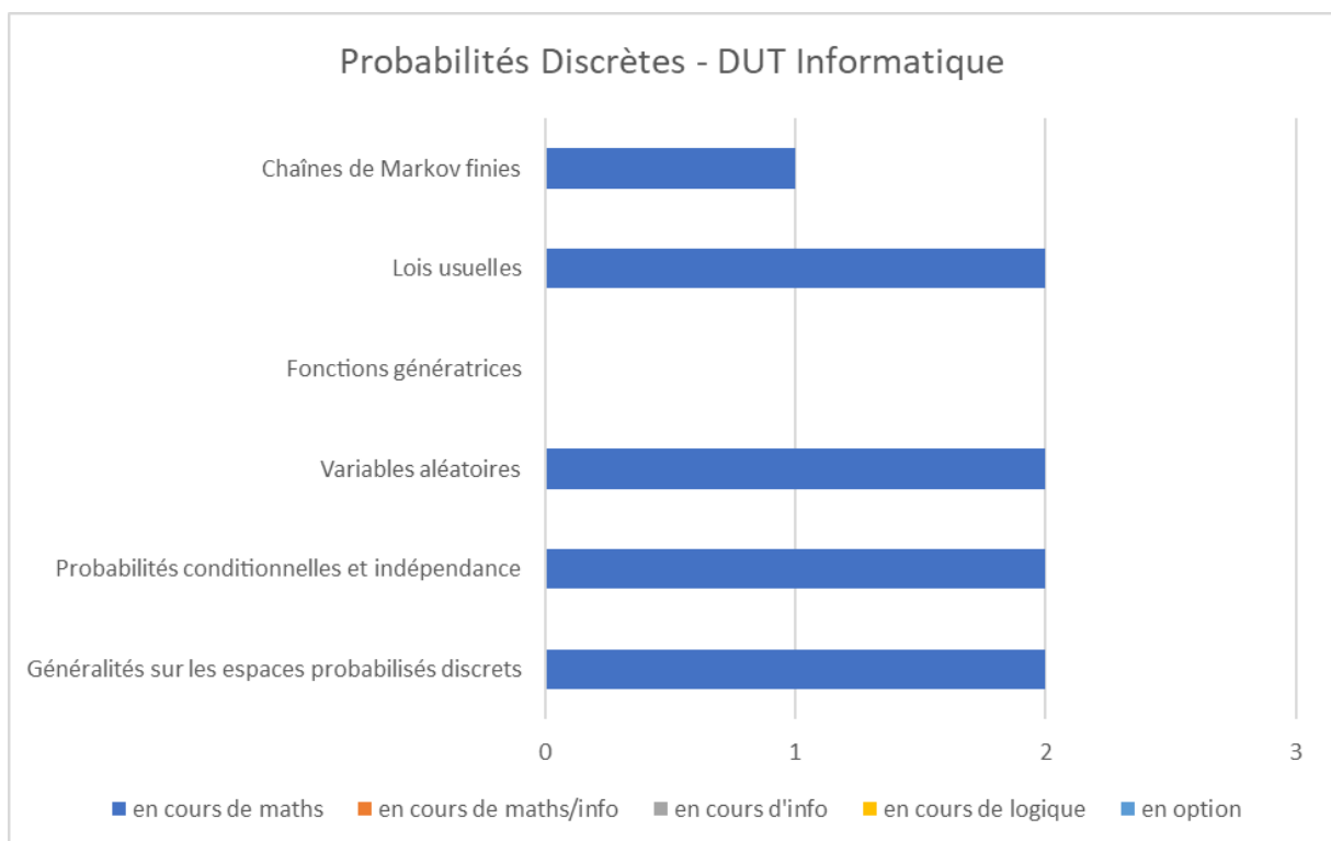
Annexe-Figure 92: Probabilités Discrètes - DUT Informatique – France
