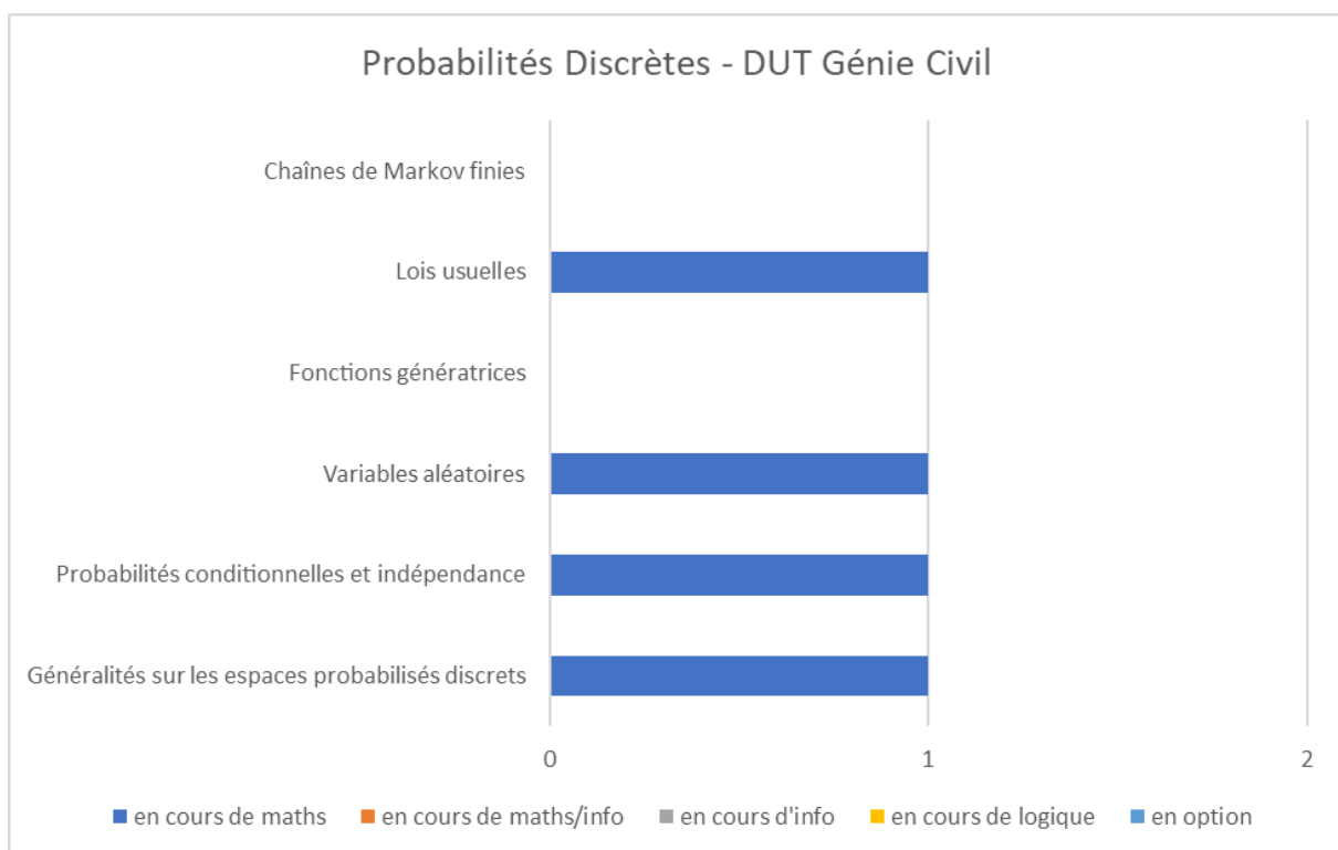
Annexe-Figure 96: Probabilités Discrètes - DUT Génie Civil – France
