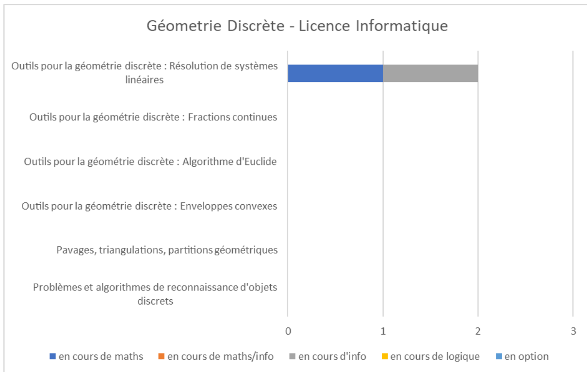
Annexe-Figure 67: Géométrie Discrète - Licence Informatique - France
