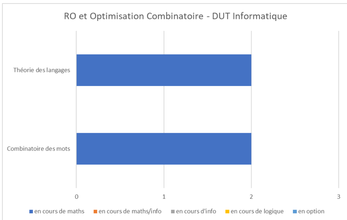
Annexe-Figure 90: RO et Optimisation Combinatoire - DUT Informatique – France
