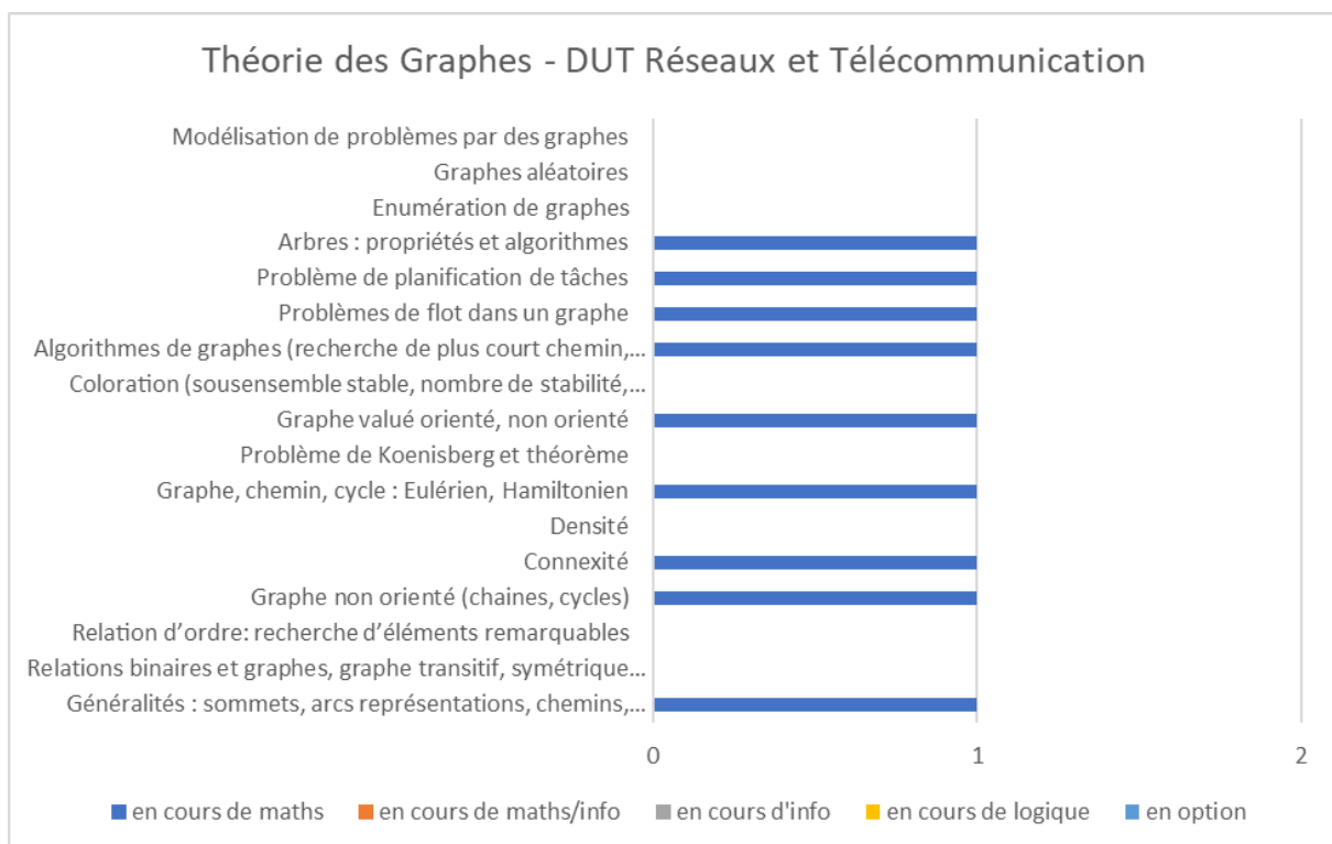
Annexe-Figure 82: Théorie des Graphes - DUT Réseaux et Télécommunication – France
