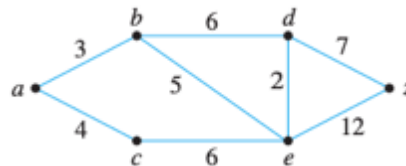
Figure 3-64: Exemple sur le plus court chemin (Epp, 2011)
