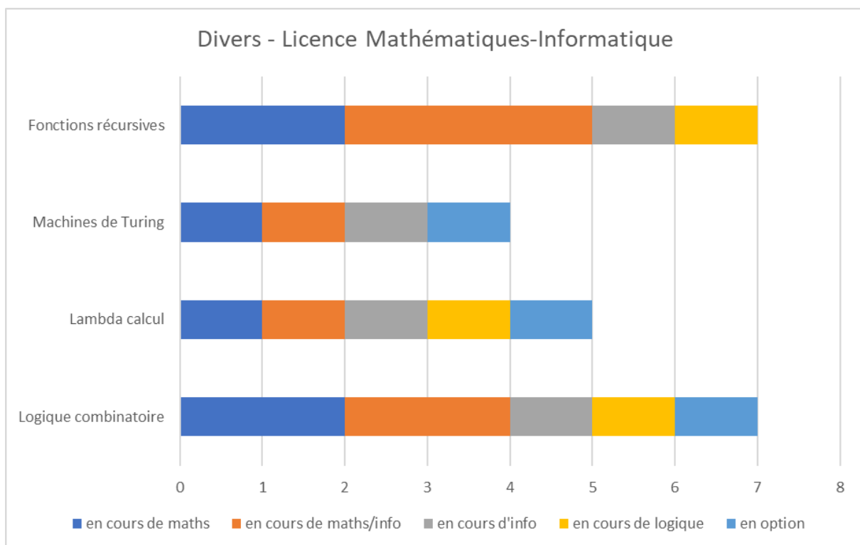
Annexe-Figure 14: Divers - Licence Mathématiques-Informatique – Liban
