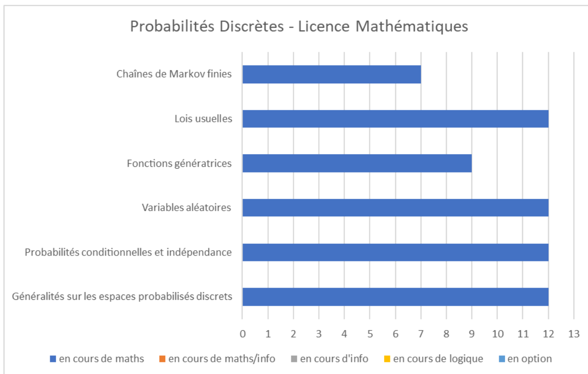
Annexe-Figure 55: Probabilités Discrètes - Licence Mathématiques – France
