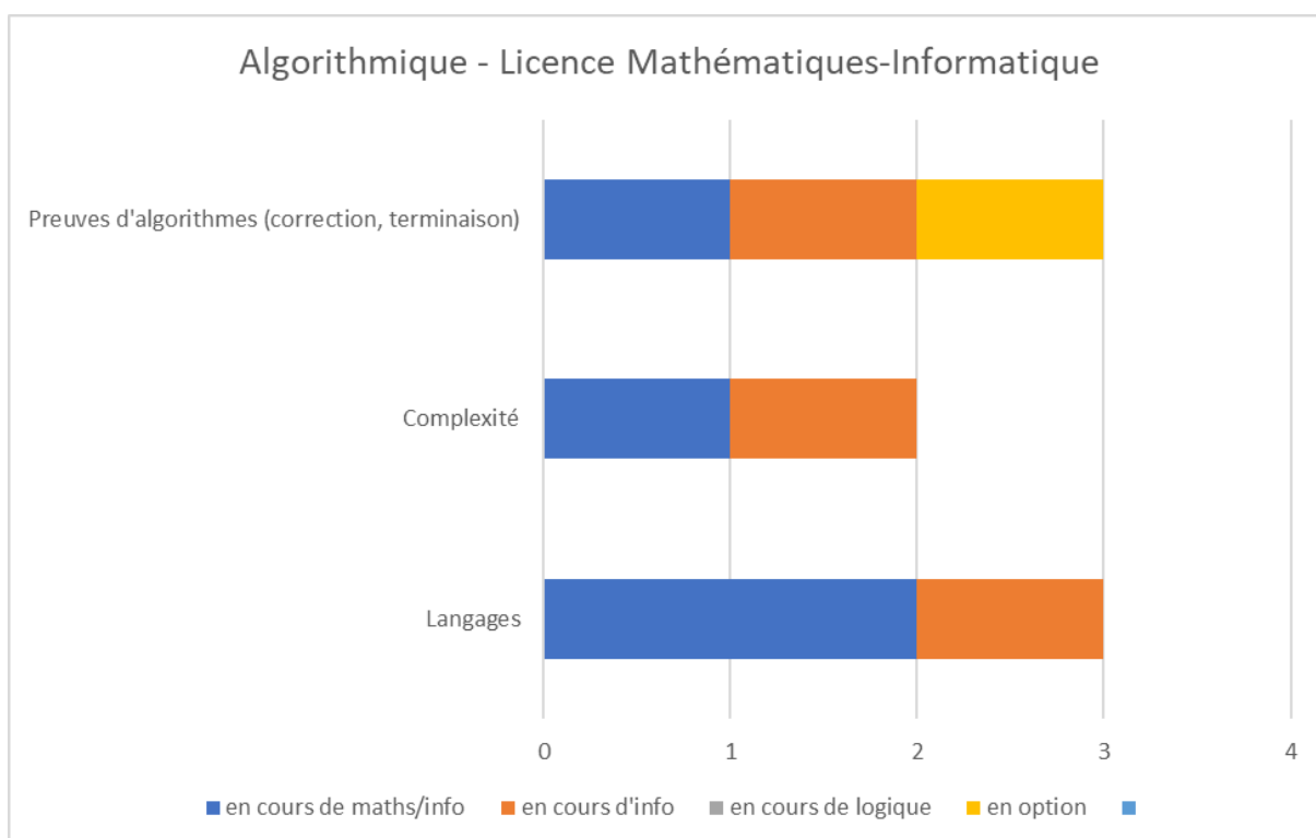
Annexe-Figure 16: Algorithmique - Licence Mathématiques-Informatique – Liban
