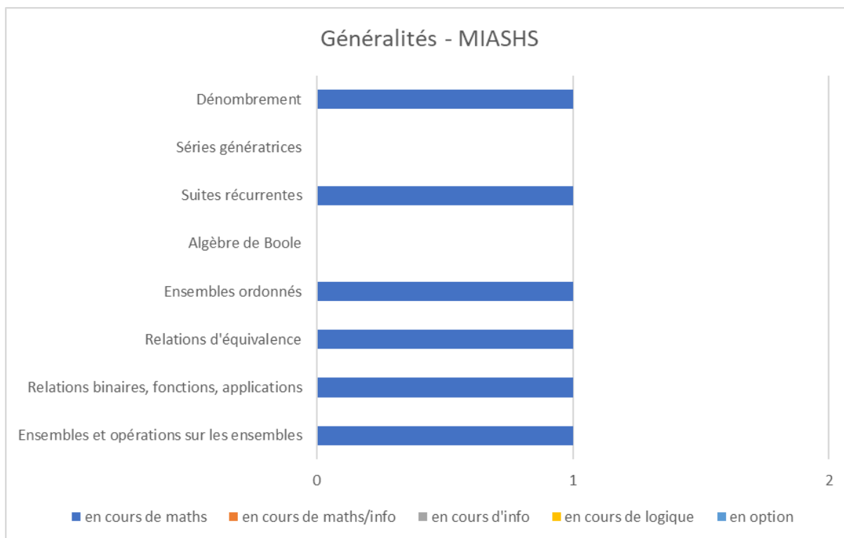
Annexe-Figure 35: Généralités - MIASHS – France
