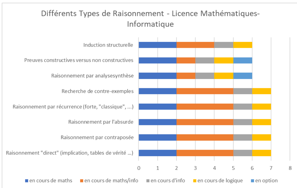
Annexe-Figure 12: Différents Types de Raisonnement - Licence Mathématiques-Informatique – Liban
