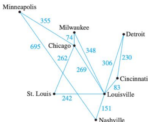
Figure 3-66: Exemple sur l'arbres couvrant de poids minimum (Epp, 2011)
