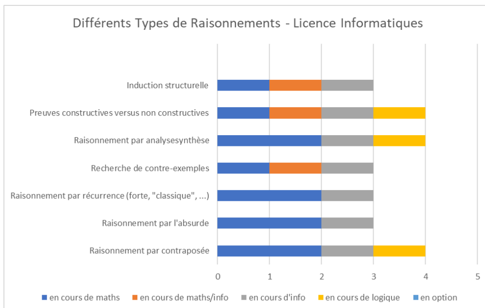
Figure 3-9: Différents Types de Raisonnements - Licence Informatique – Liban
