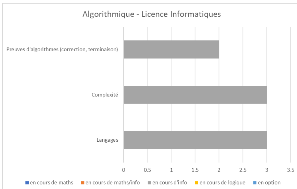
Figure 3-21: Algorithmique - Licence Informatique – France
