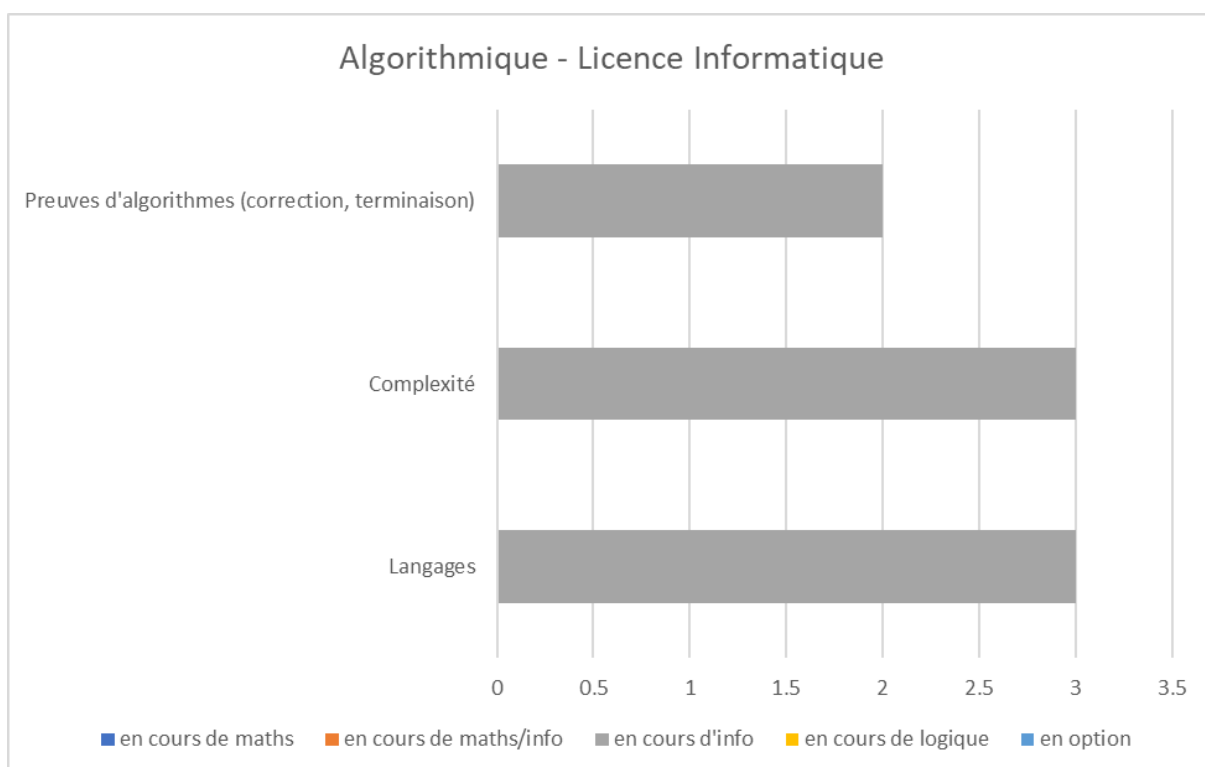
Annexe-Figure 62: Algorithmique - Licence Informatique – France
