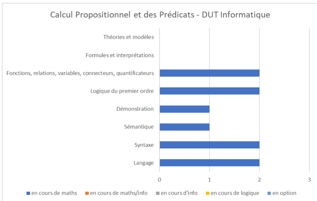
Annexe-Figure 86: Calcul Propositionnel et des Prédicats - DUT Informatique – France
