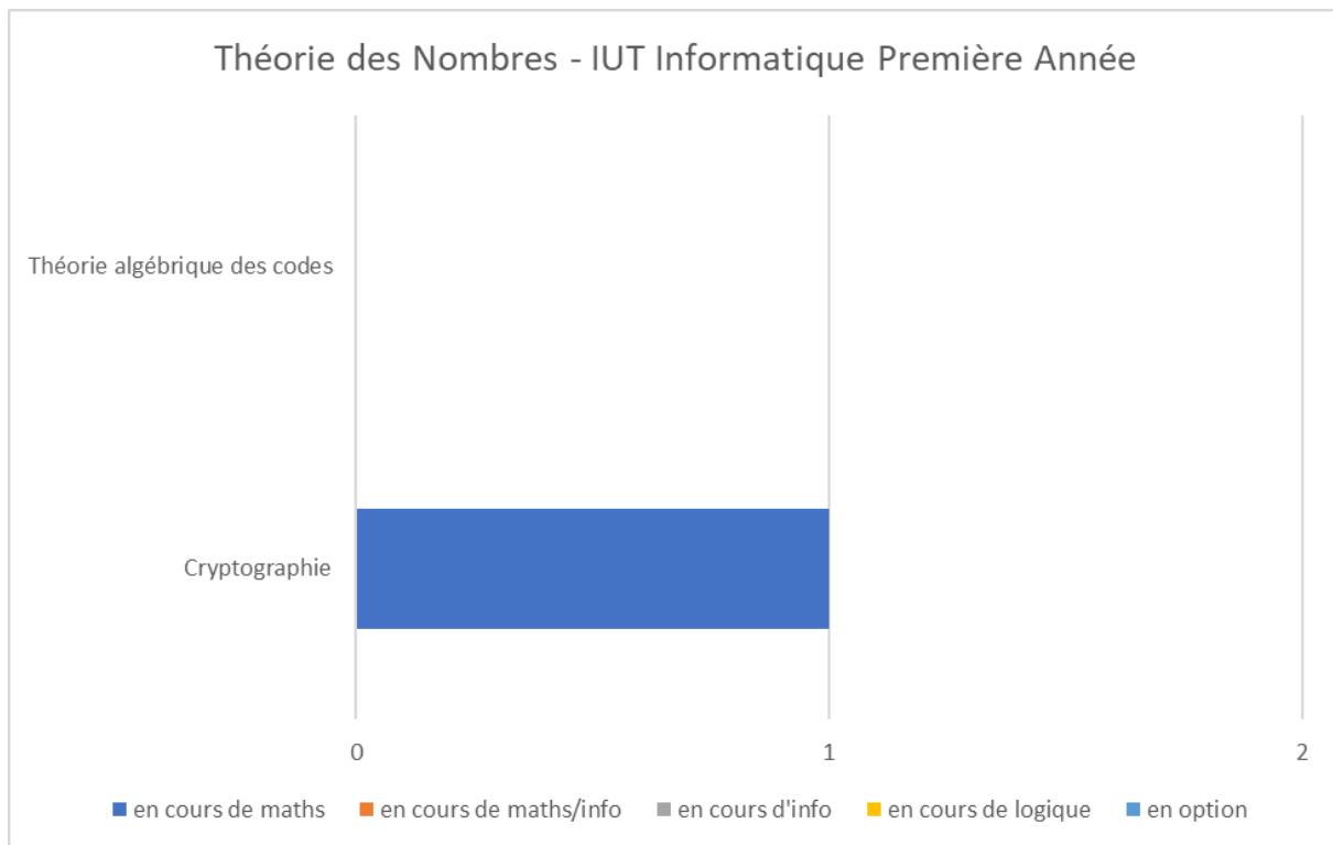
Annexe-Figure 75: Théorie des Nombres - IUT Informatique Première Année – France
