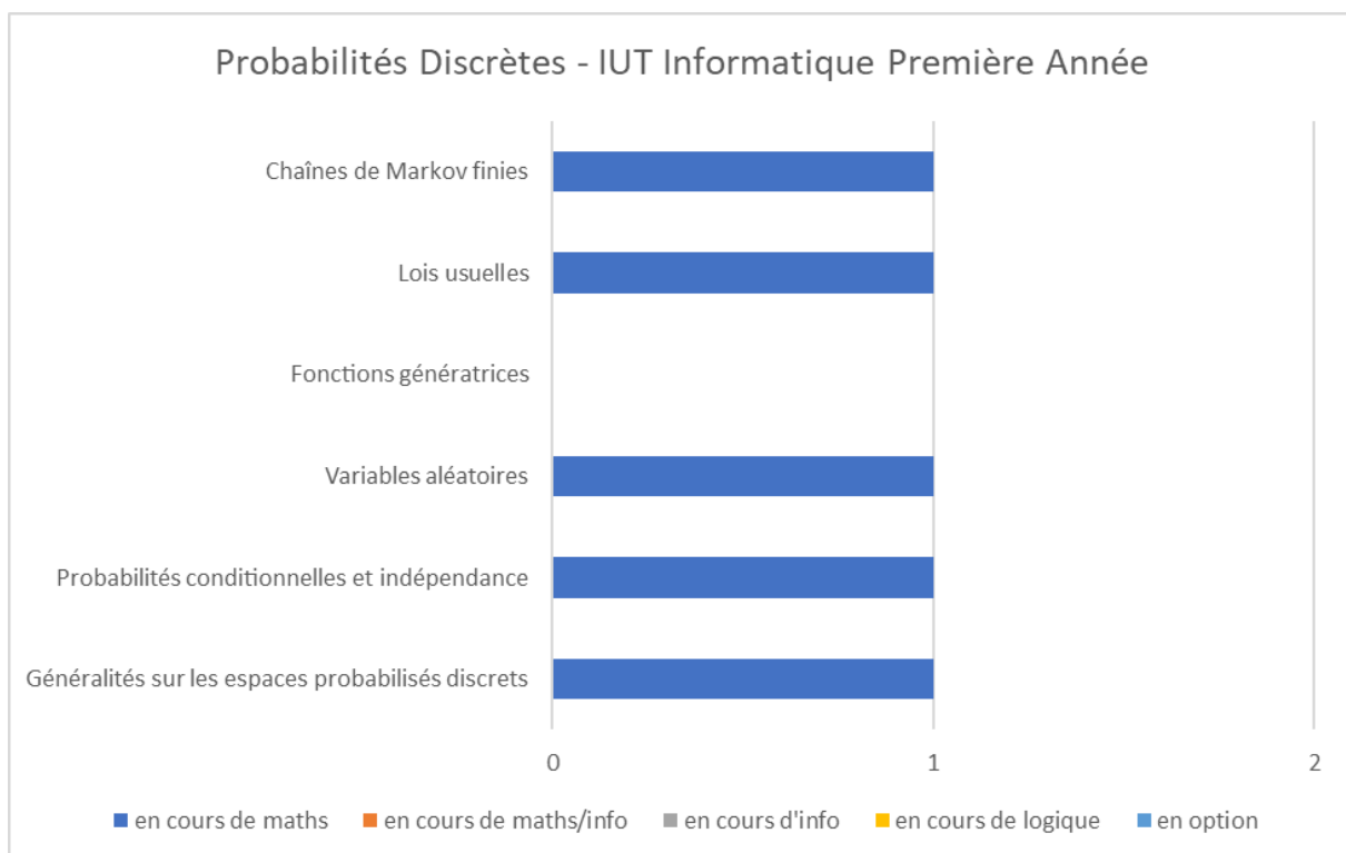
Annexe-Figure 76: Probabilités Discrètes - IUT Informatique Première Année – France
