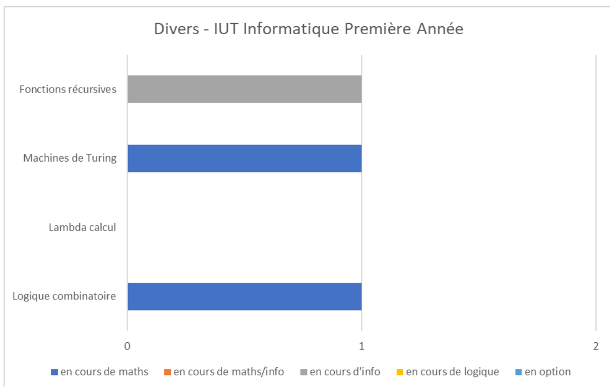
Annexe-Figure 70: Divers - IUT Informatique Première Année - France
