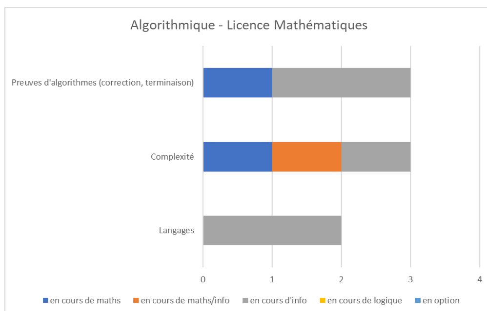
Figure 3-10: Algorithmique - Licence Mathématiques – Liban
