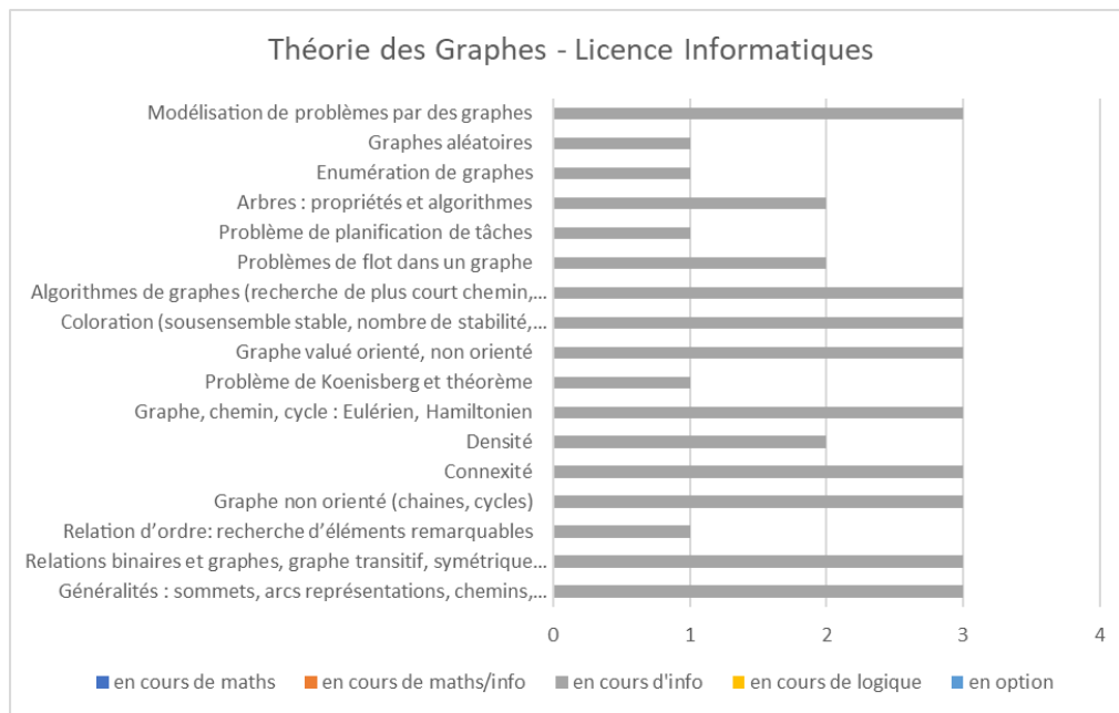
Figure 3-15: Théorie des Graphes - Licence Informatique – France
