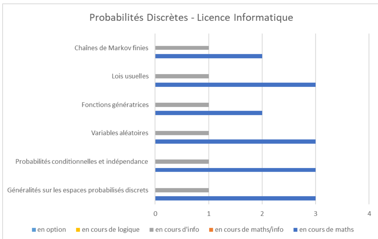
Annexe-Figure 66: Probabilités Discrètes - Licence Informatique – France
