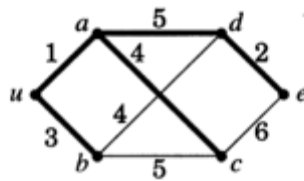
Figure 3-65: Exemple sur le plus court chemin (West, 2002)
