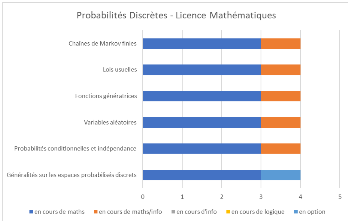
Annexe-Figure 9: Probabilités Discrètes - Licence Mathématiques - Liban
