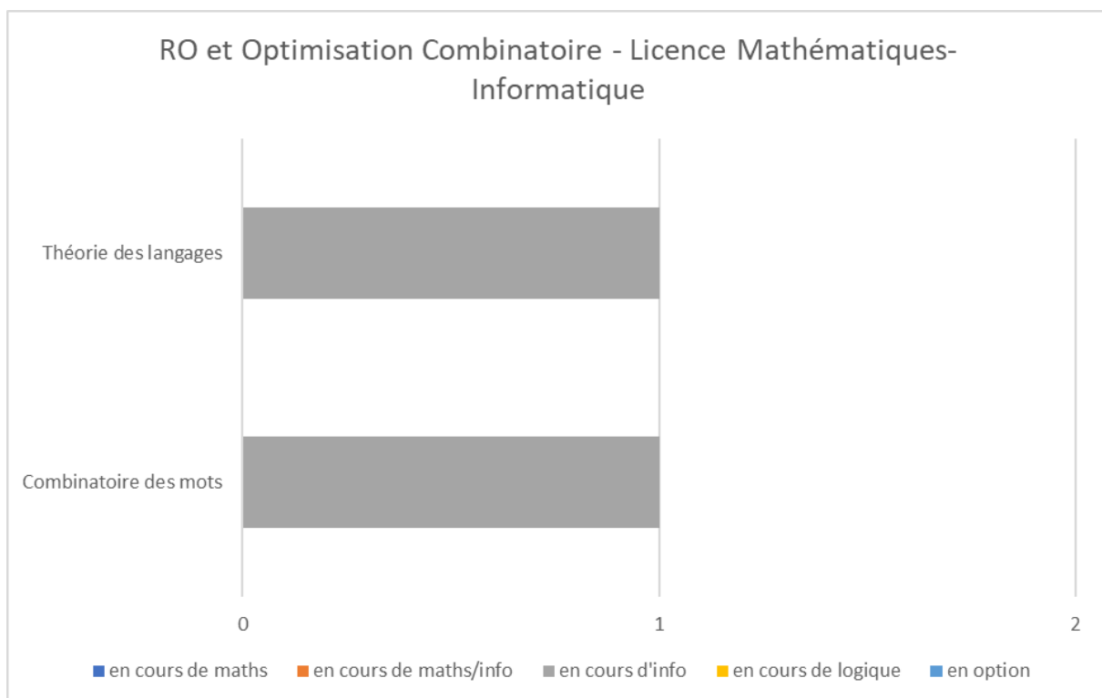
Annexe-Figure 44: RO et Optimisation Combinatoire - Licence Mathématiques-Informatique – France
