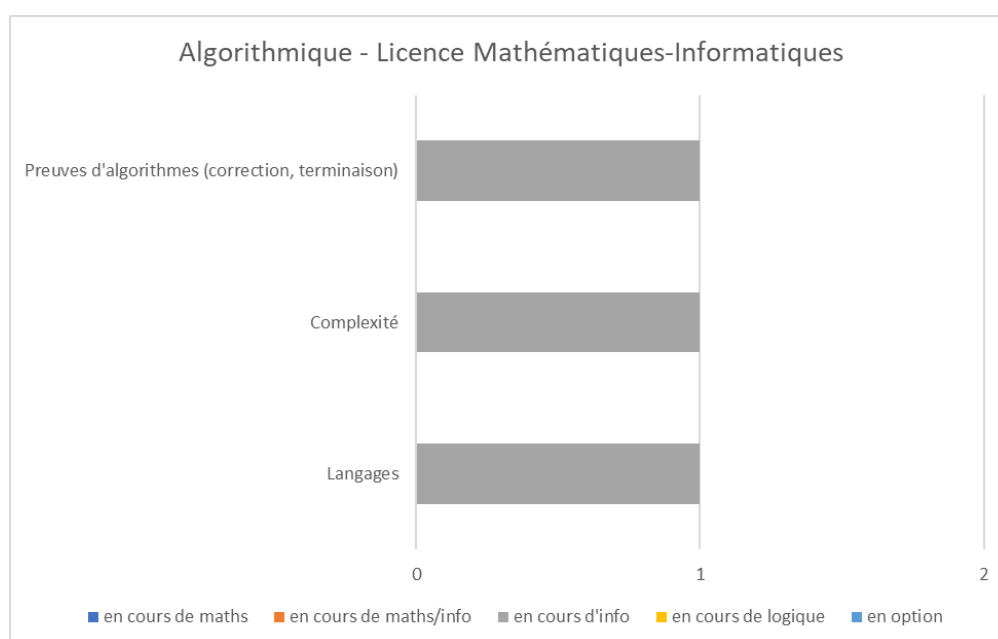
Figure 3-20: Algorithmique - Licence Mathématiques-Informatique – France
