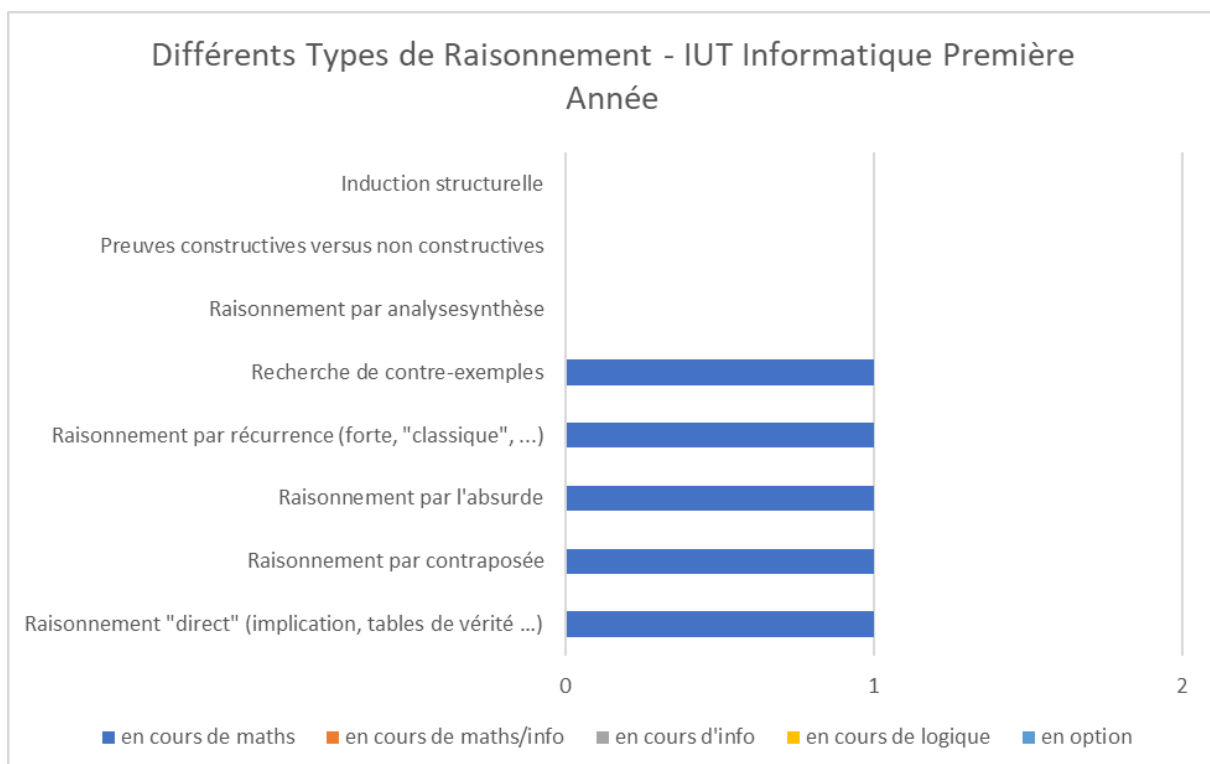
Annexe-Figure 68: Différents Types de Raisonnement - IUT Informatique Première Année – France
