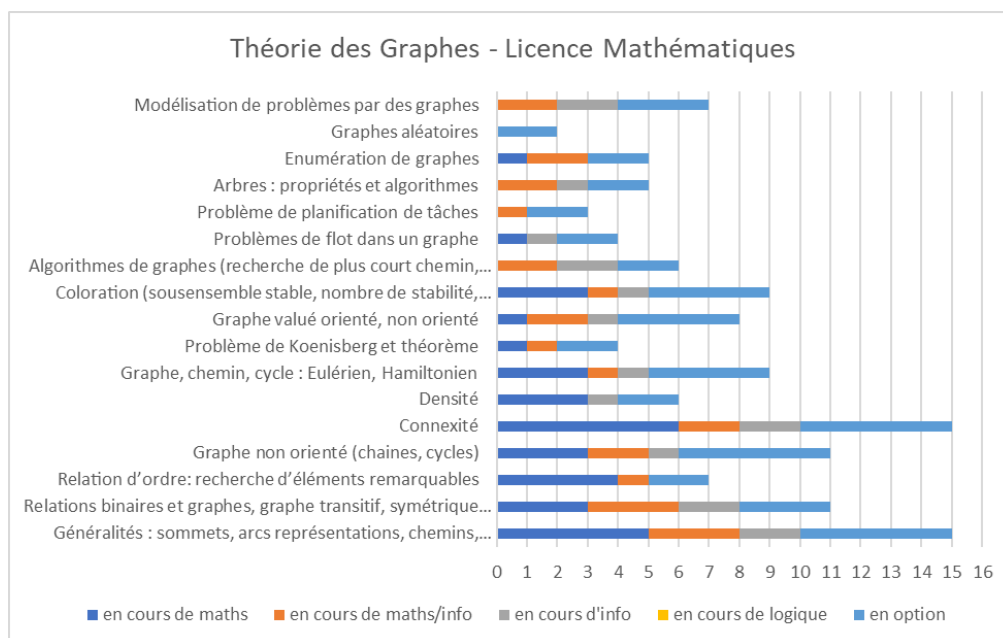
Figure 3-13: Théorie des Graphes - Licence Mathématiques – France
