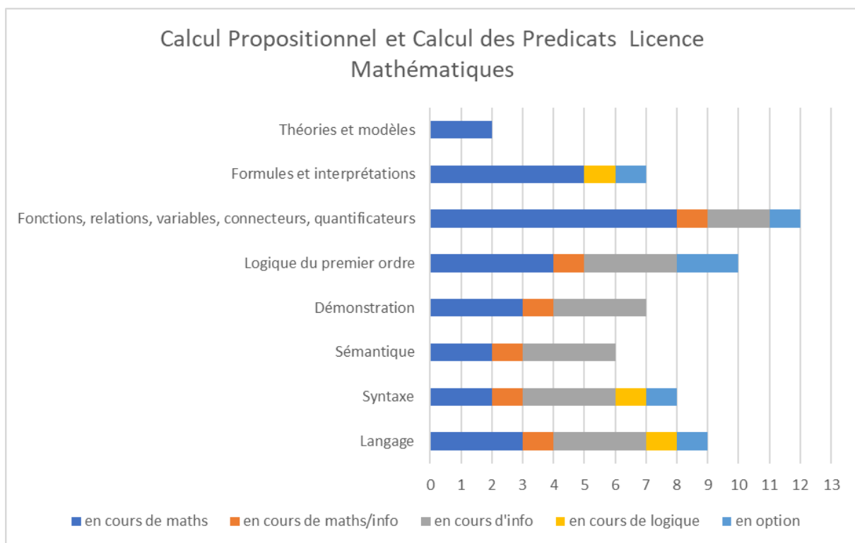
Annexe-Figure 48: Calcul Propositionnel et Calcul des Prédicats Licence Mathématiques – France
