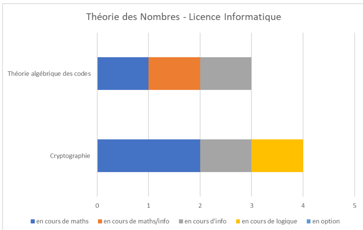
Annexe-Figure 30: Théorie des Nombres - Licence Informatique – Liban
