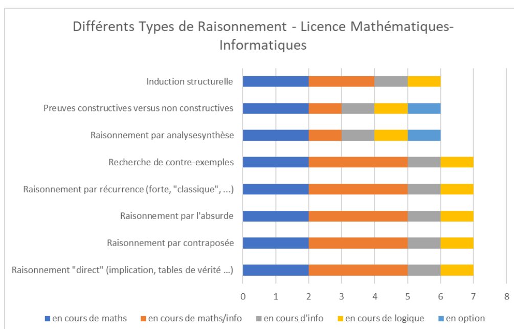
Figure 3-8: Différents Types de Raisonnement - Licence Mathématiques-Informatique – Liban
