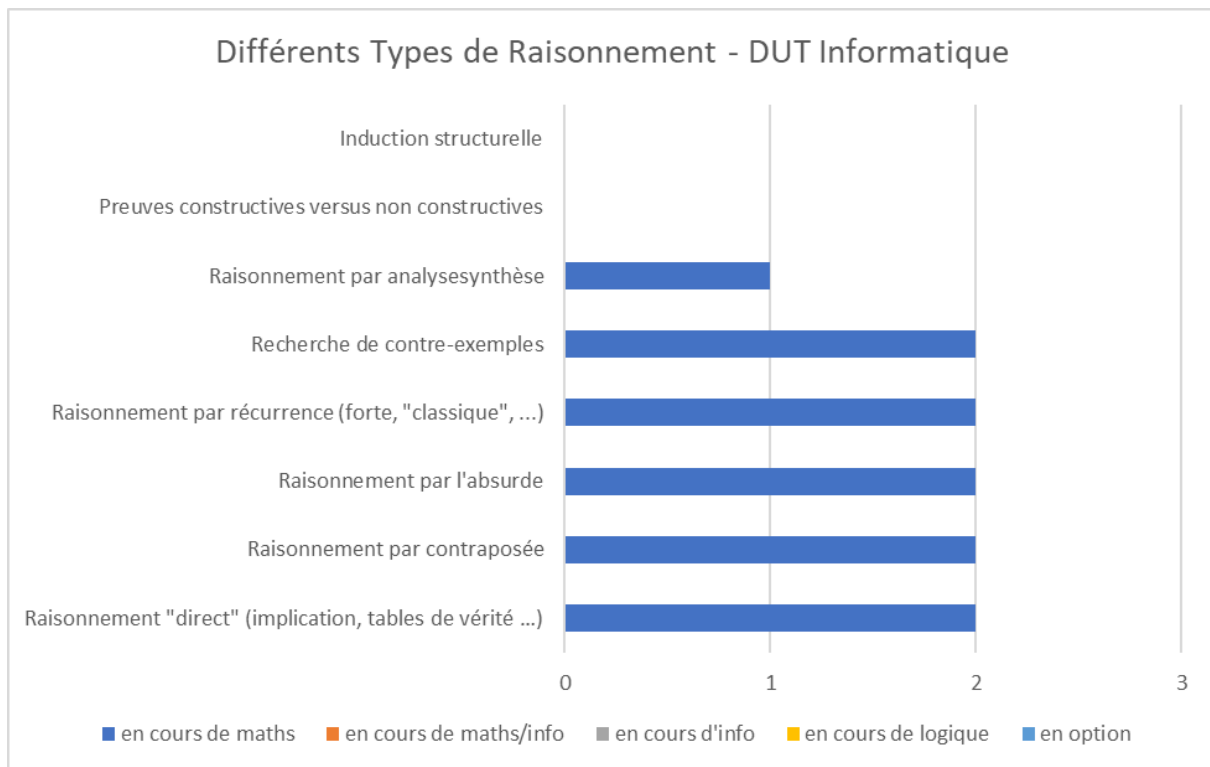
Annexe-Figure 85: Différents Types de Raisonnement - DUT Informatique – France
