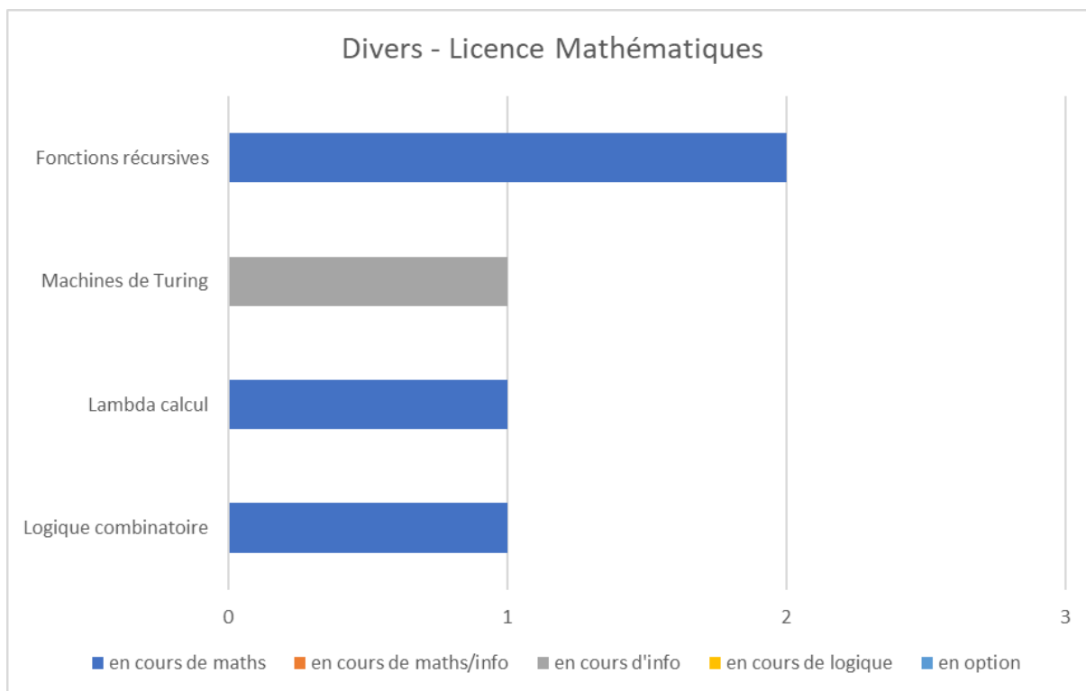
Annexe-Figure 3: Divers - Licence Mathématiques – Liban
