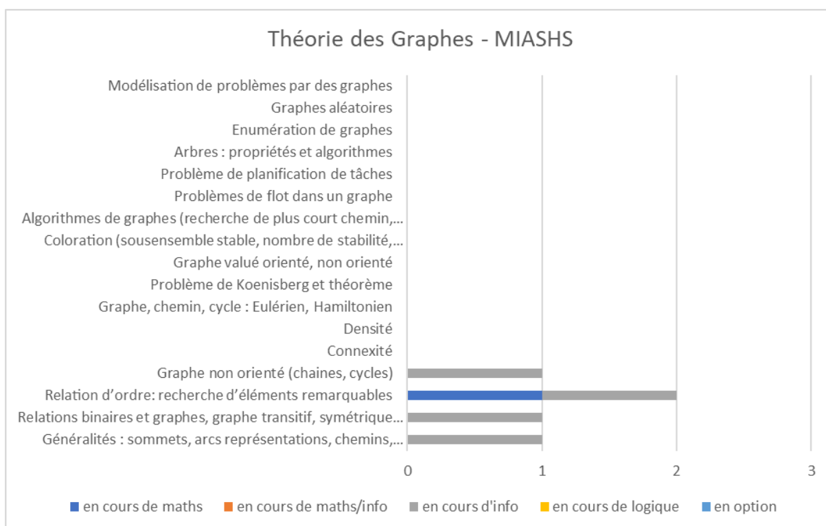
Annexe-Figure 36: Théorie des Graphes - MIASHS – France
