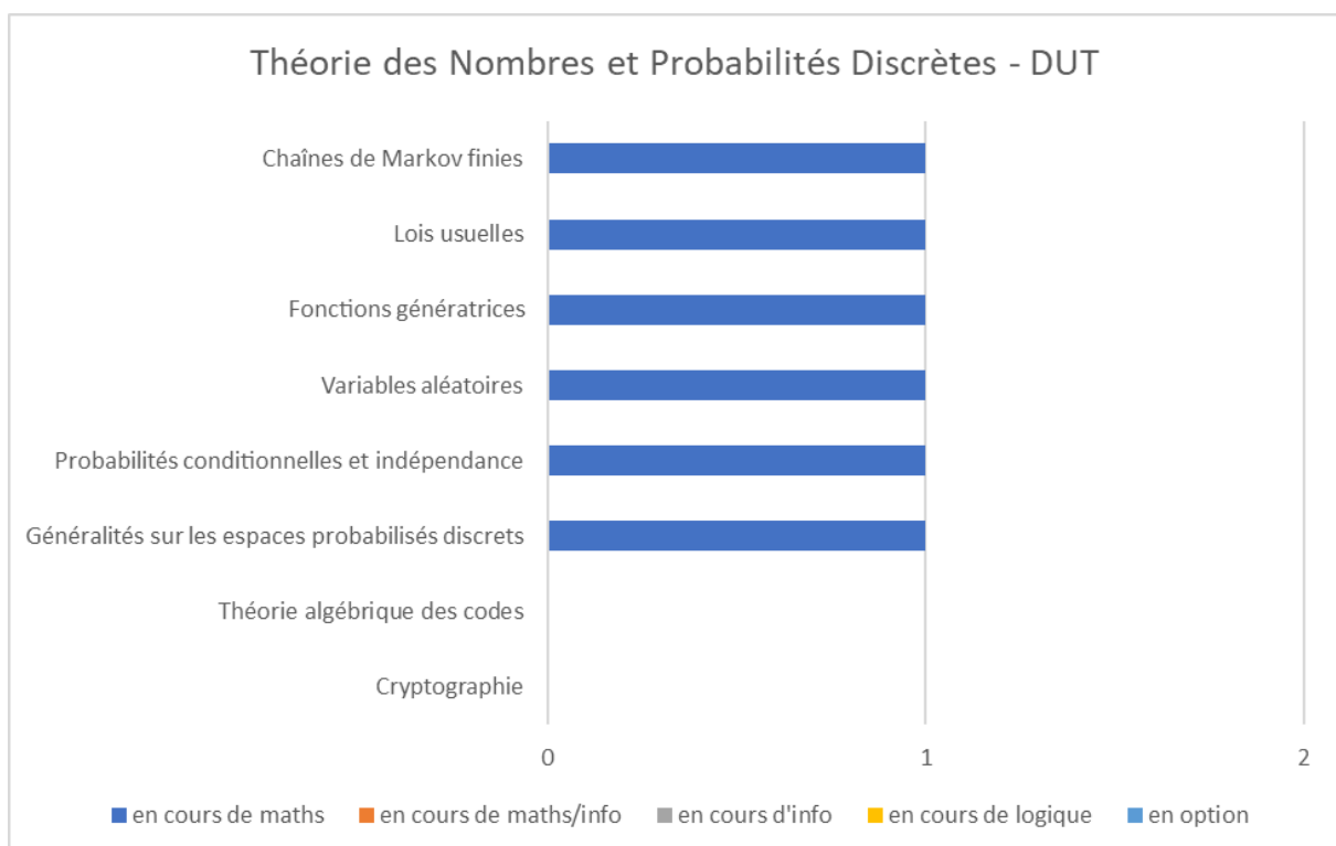
Annexe-Figure 78: Théorie des Nombres et Probabilités Discrètes - DUT – France
