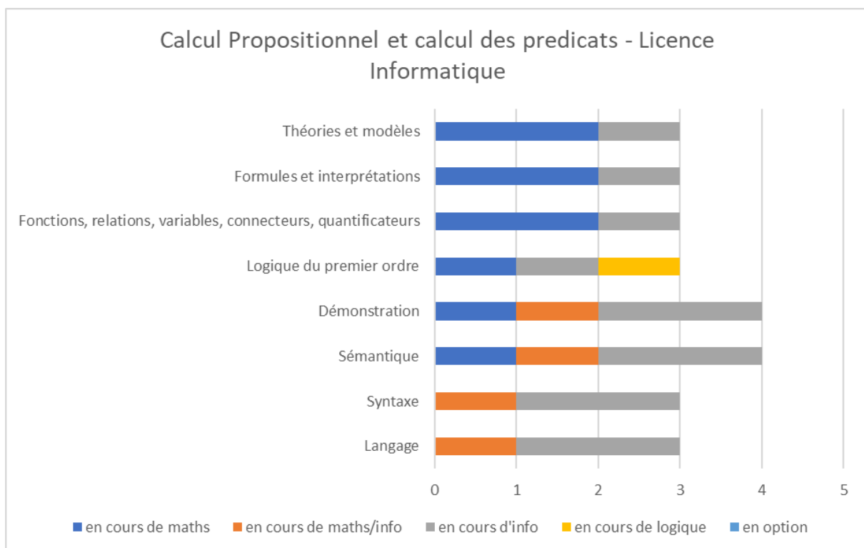
Annexe-Figure 24: Calcul Propositionnel et calcul des Prédicats - Licence Informatique – Liban
