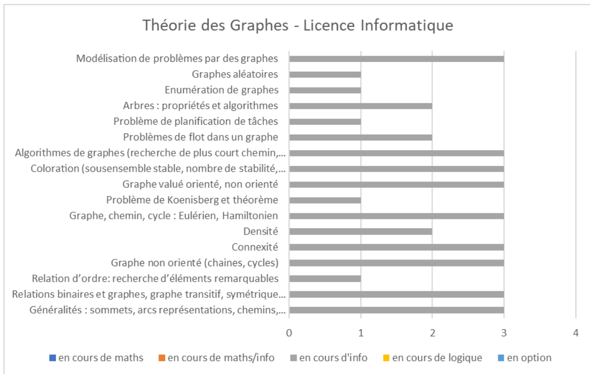
Annexe-Figure 63: Théorie des Graphes - Licence Informatique – France
