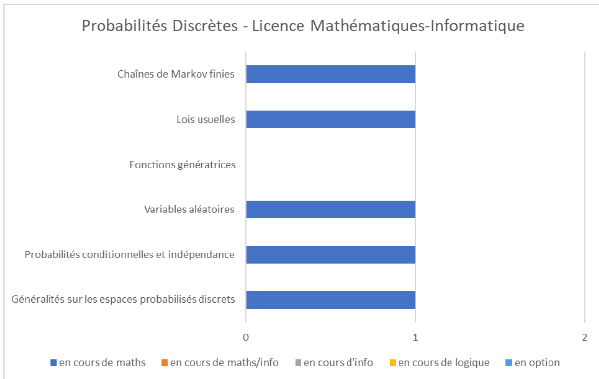
Annexe-Figure 45: Probabilités Discrètes - Licence Mathématiques-Informatique – France
