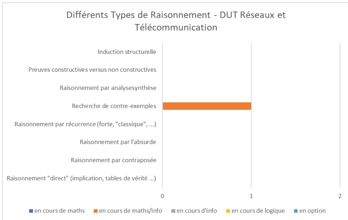
Annexe-Figure 79: Différents Types de Raisonnement - DUT Réseaux et Télécommunication – France
