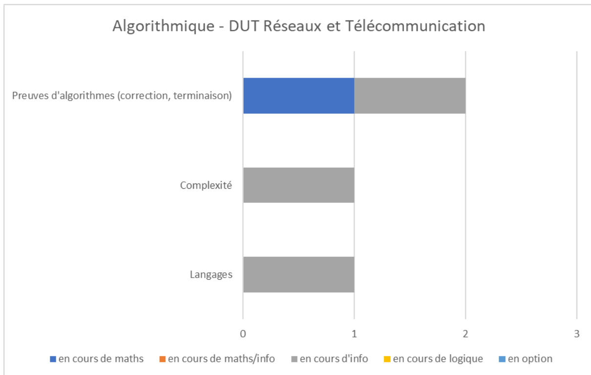
Annexe-Figure 81: Algorithmique - DUT Réseaux et Télécommunication – France
