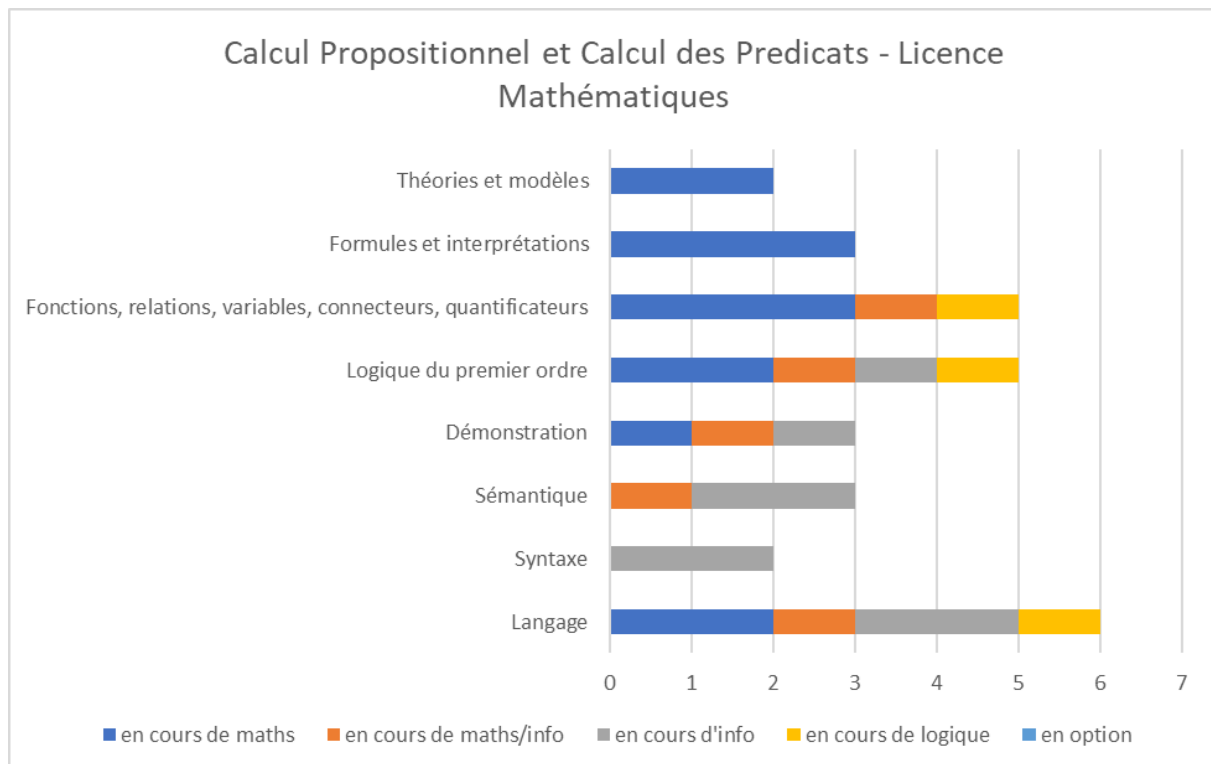
Annexe-Figure 2: Calcul Propositionnel et Calcul des Prédicats - Licence Mathématiques – Liban
