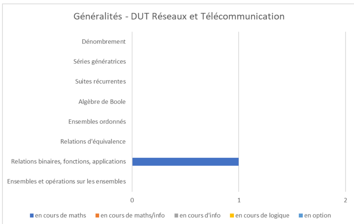
Annexe-Figure 80: Généralités - DUT Réseaux et Télécommunication – France
