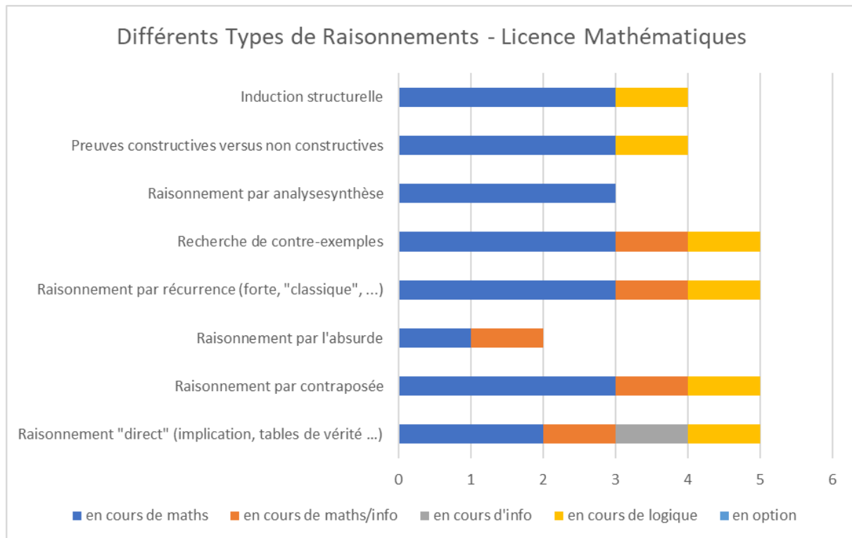
Annexe-Figure 1: Différents Types de Raisonnements - Licence Mathématiques – Liban
