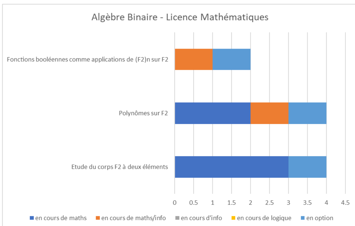
Annexe-Figure 56: Algèbre Binaire - Licence Mathématiques – France
