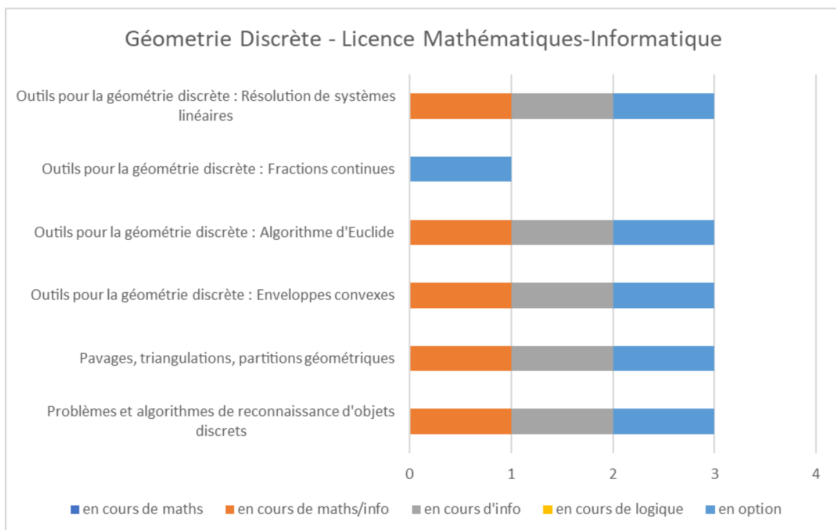
Annexe-Figure 22: Géométrie Discrète - Licence Mathématiques-Informatique – Liban
