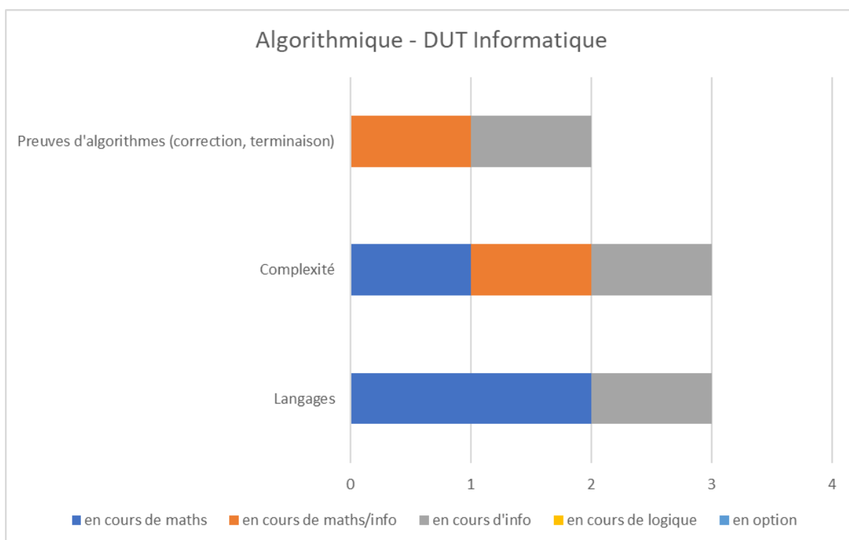
Annexe-Figure 88: Algorithmique - DUT Informatique – France
