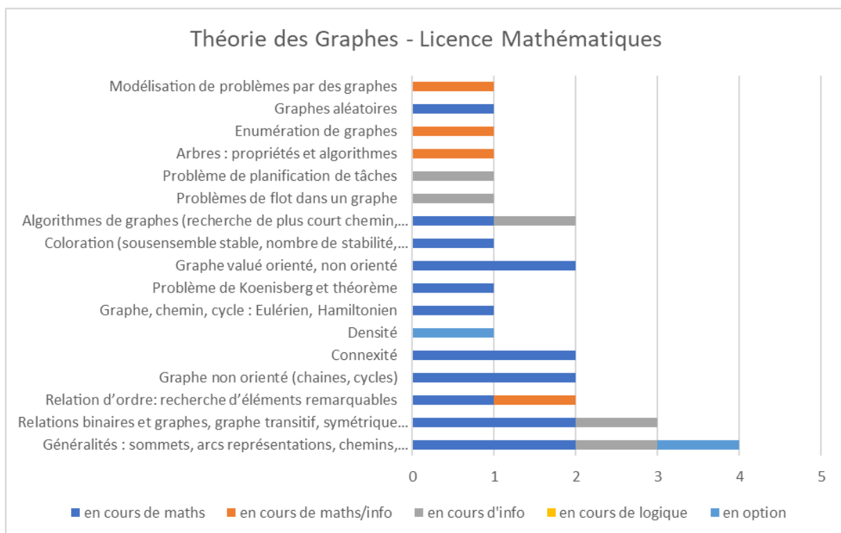
Annexe-Figure 6: Théorie des Graphes - Licence Mathématiques – Liban
