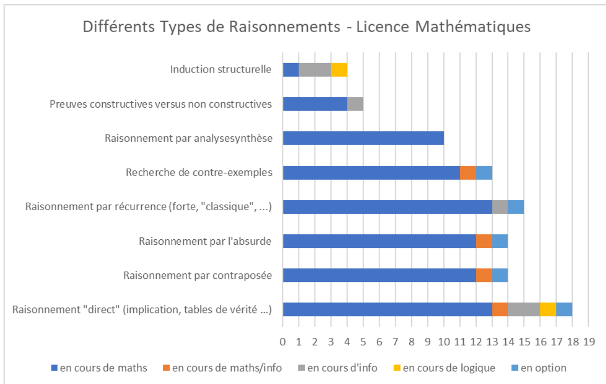
Annexe-Figure 47: Différents Types de Raisonnements - Licence Mathématiques – France
