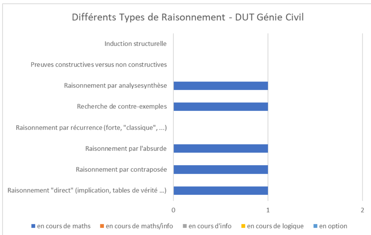
Annexe-Figure 94: Différents Types de Raisonnement - DUT Génie Civil – France
