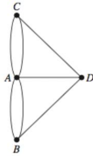
Figure 3-23: Un multigraphe de la ville de Königsberg
