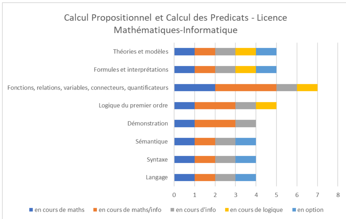
Annexe-Figure 13: Calcul Propositionnel et Calcul des Prédicats - Licence Mathématiques-Informatique – Liban
