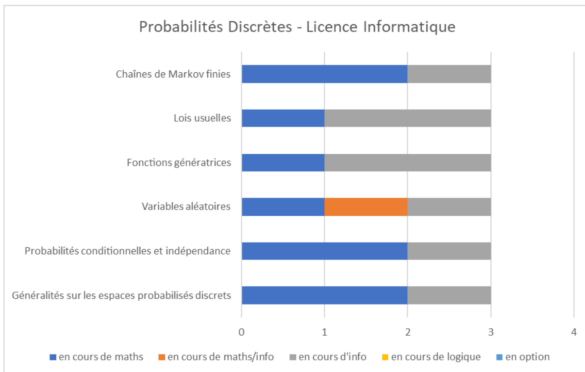
Annexe-Figure 31: Probabilités Discrètes - Licence Informatique – Liban
