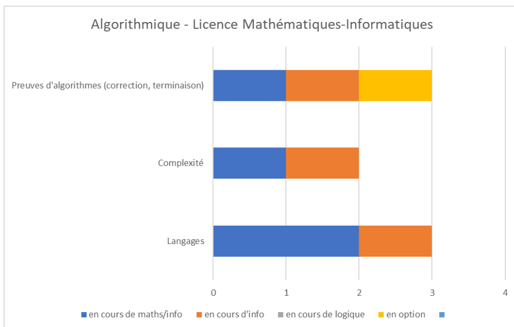
Figure 3-11: Algorithmique - Licence Mathématiques-Informatique – Liban
