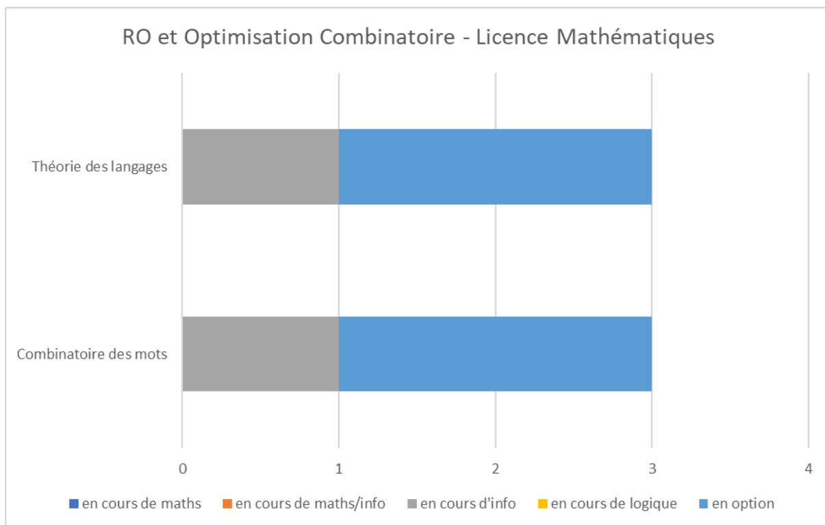
Annexe-Figure 53: RO et Optimisation Combinatoire - Licence Mathématiques – France
