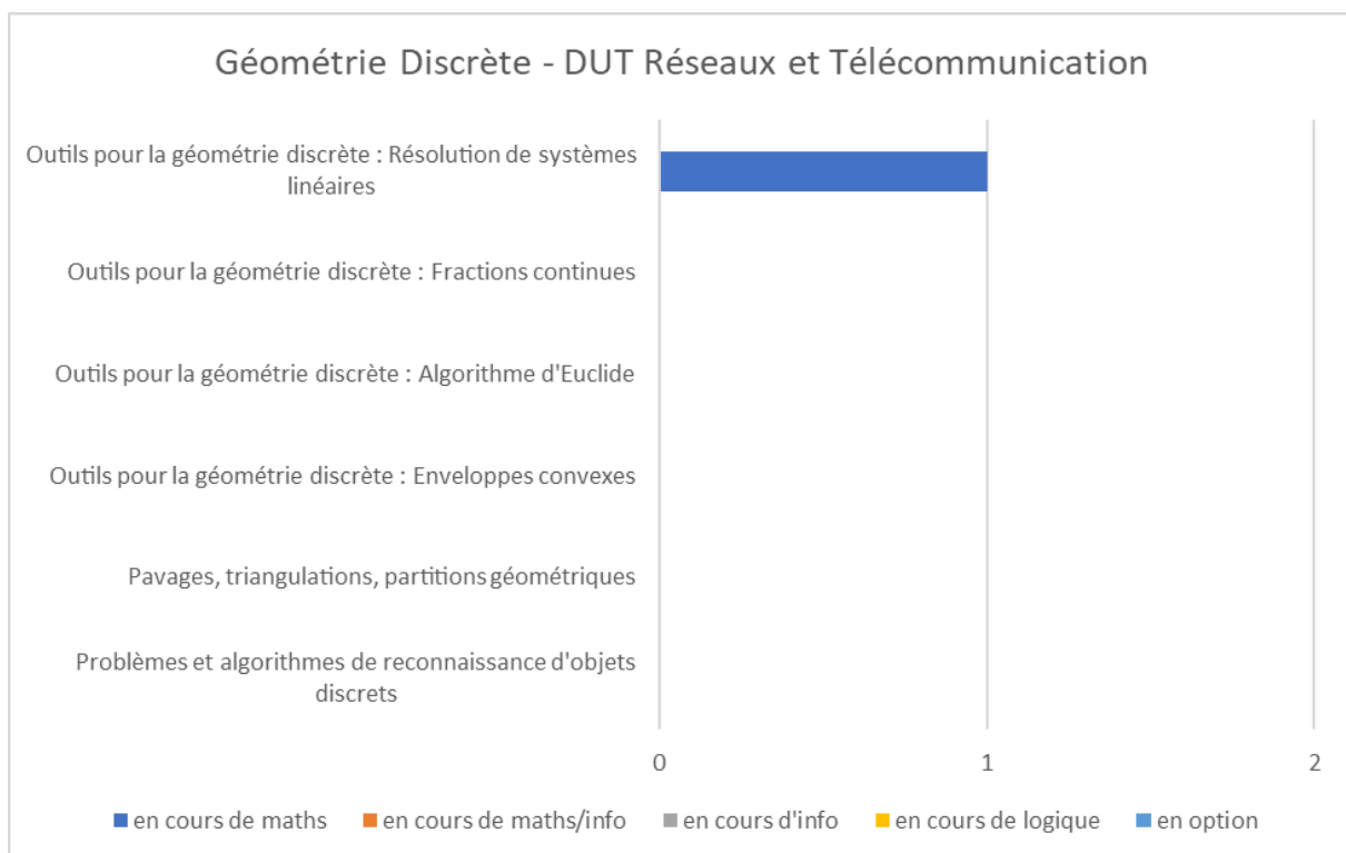
Annexe-Figure 84: Géométrie Discrète - DUT Réseaux et Télécommunication – France
