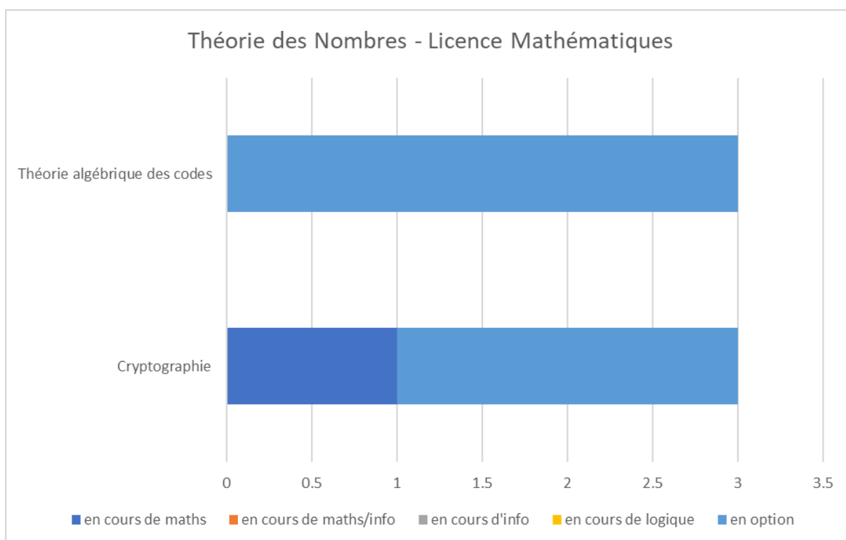
Annexe-Figure 54: Théorie des Nombres - Licence Mathématiques – France
