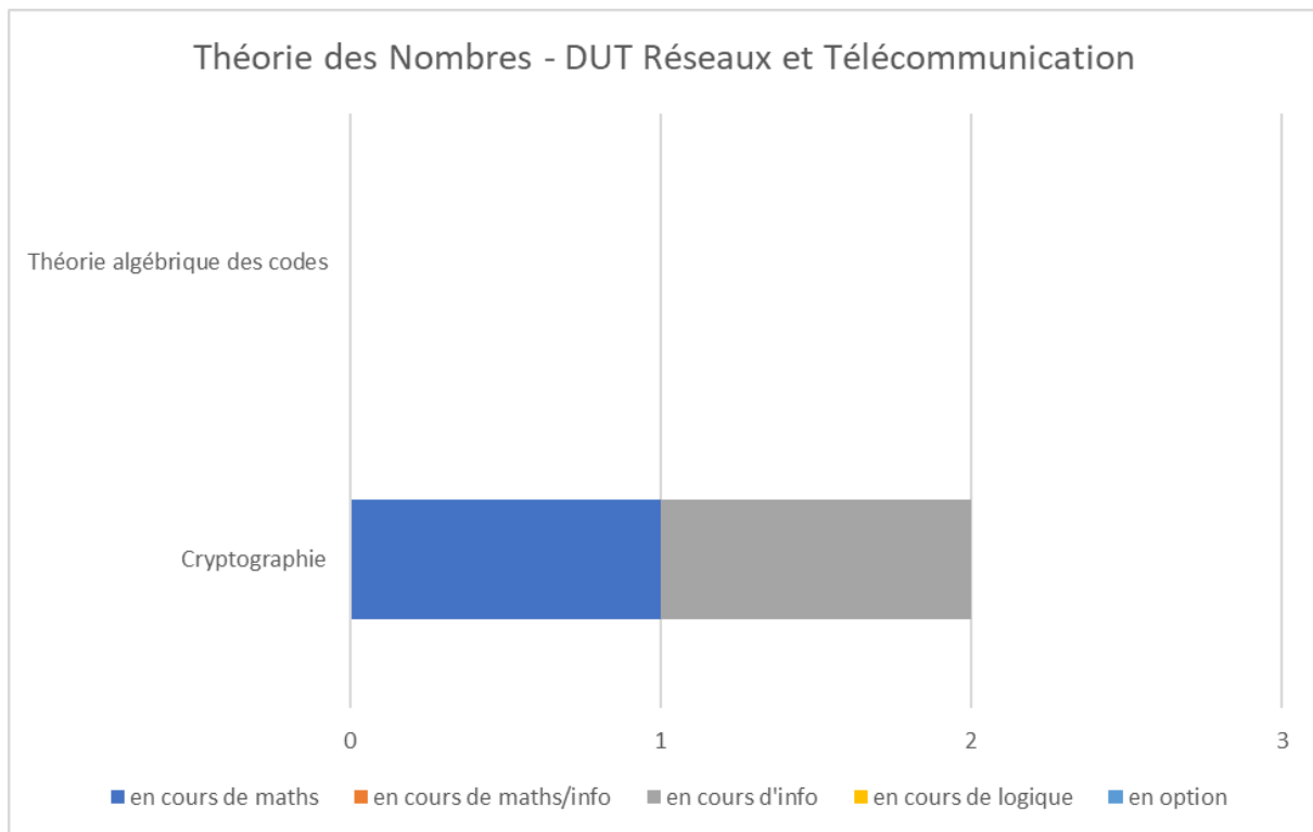
Annexe-Figure 83: Théorie des Nombres - DUT Réseaux et Télécommunication – France
