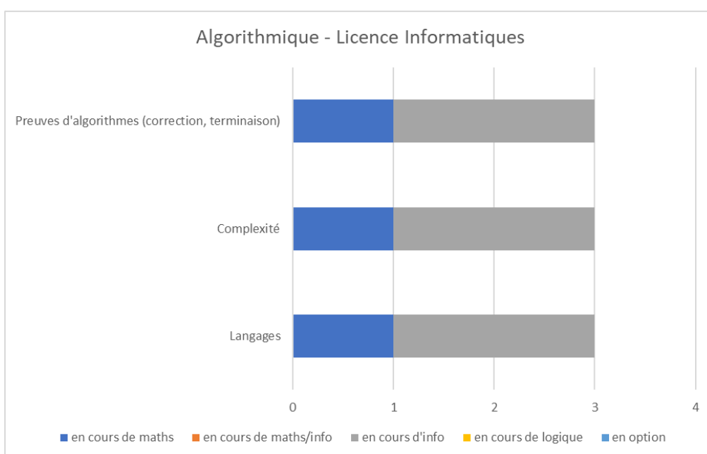
Figure 3-12: Algorithmique - Licence Informatique – Liban
