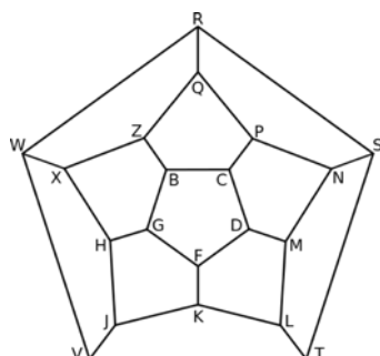
Figure 3-24: Voyage autour du monde (Hamilton)
