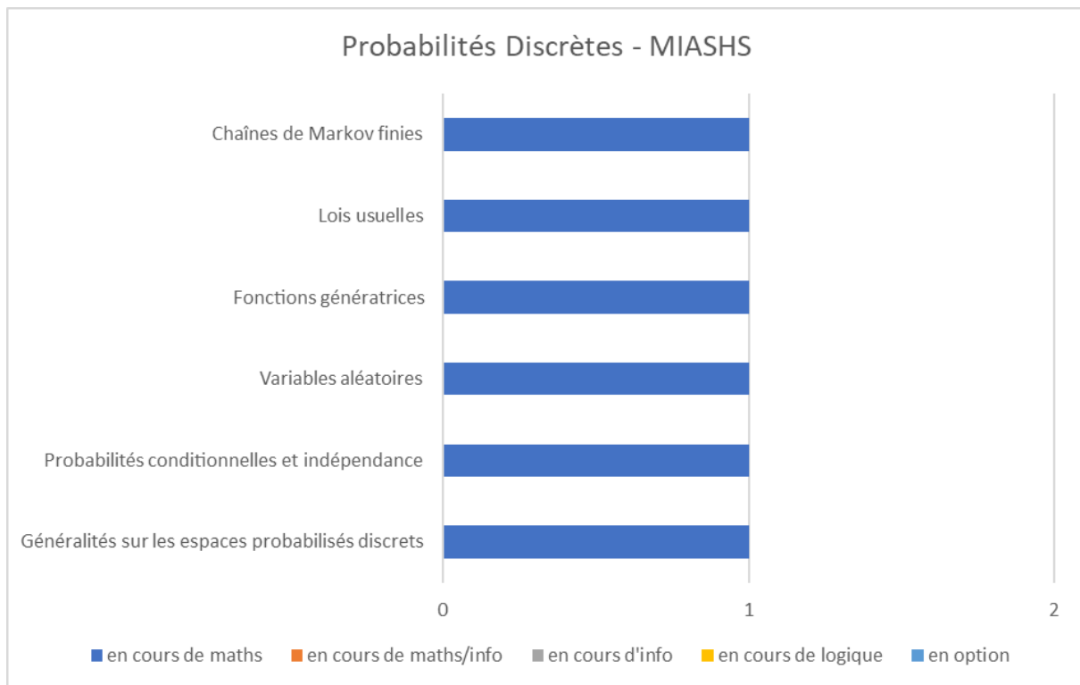
Annexe-Figure 37: Probabilités Discrètes - MIASHS – France
