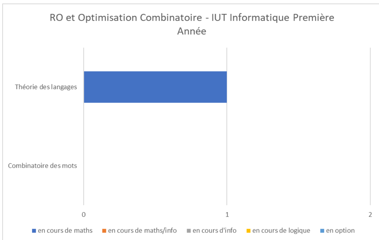
Annexe-Figure 74: RO et Optimisation Combinatoire - IUT Informatique Première Année – France
