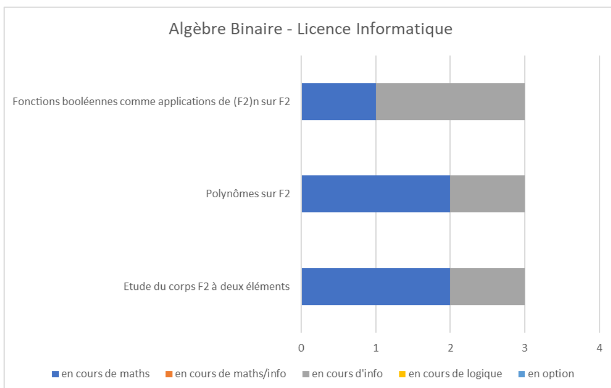
Annexe-Figure 32: Algèbre Binaire - Licence Informatique – Liban
