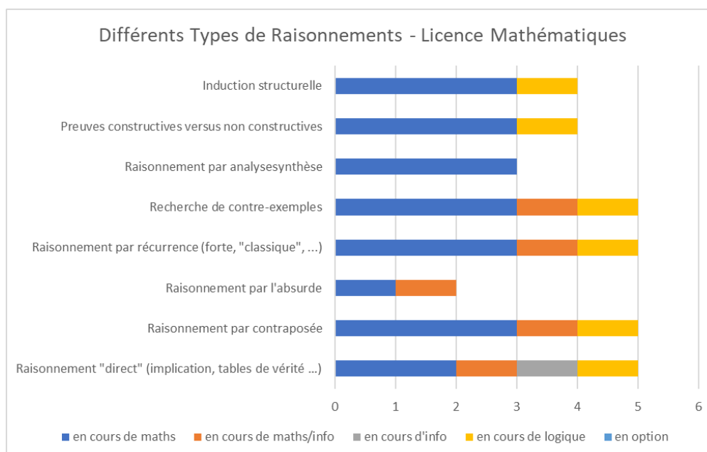
Figure 3-7: Différents Types de Raisonnements - Licence Mathématiques – Liban
