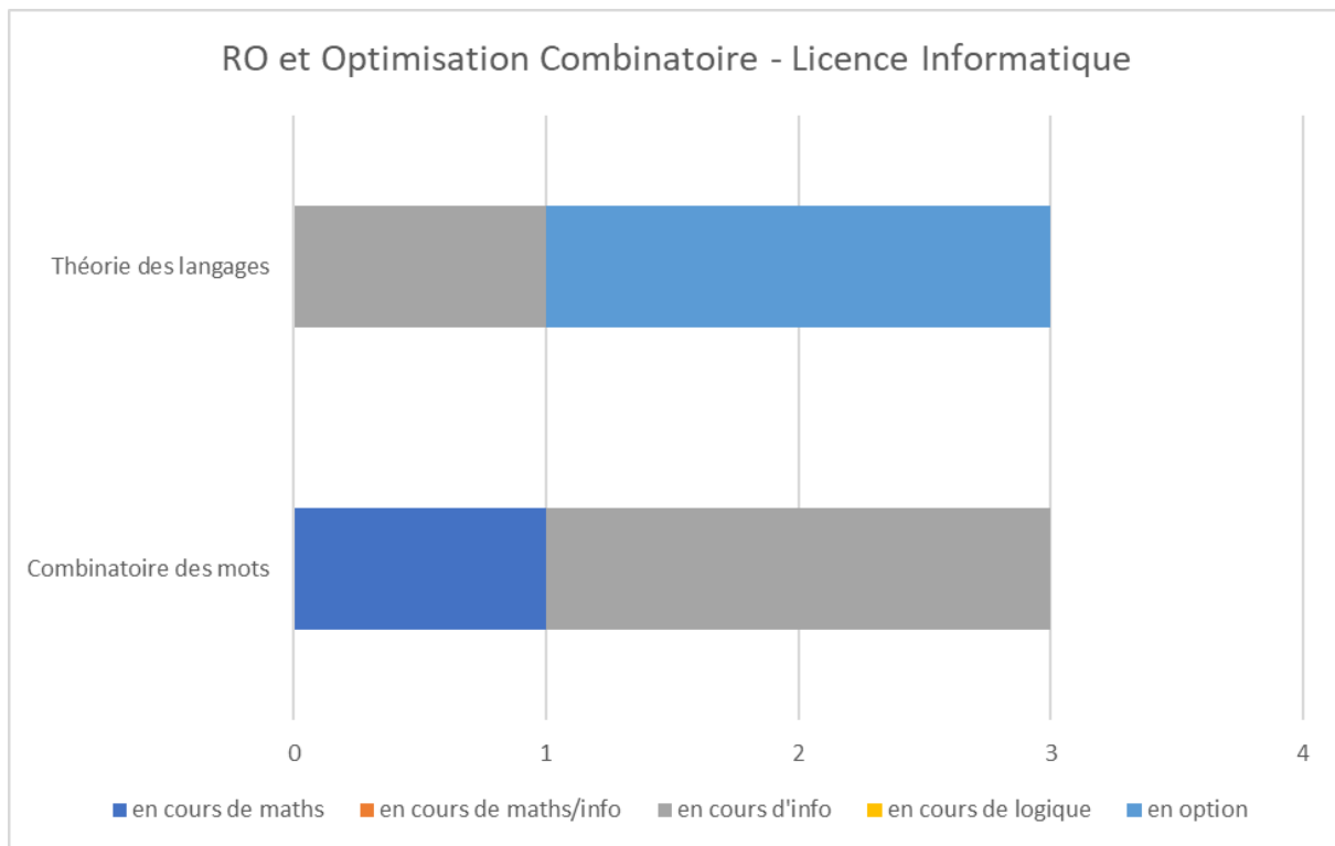
Annexe-Figure 29: RO et Optimisation Combinatoire - Licence Informatique – Liban
