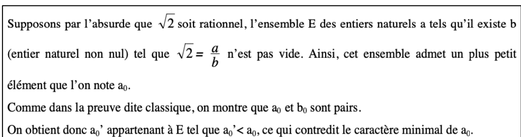
Figure 2-2: Preuve par l'absurde et minimalité (Battie V. , 2003, p. 233)
