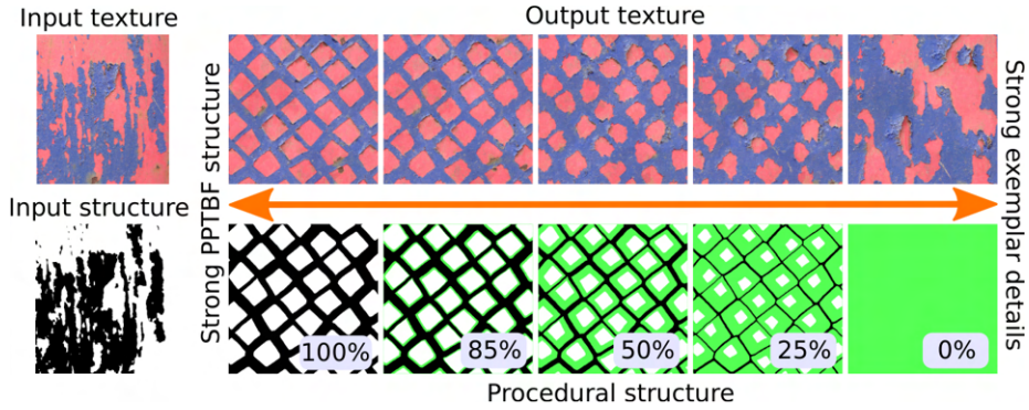
FIGURE 2.18 – Algorithme de synthèse semi-procédurale présentée par Guehl et al. [GAD + 20]. Un masque est synthétisé au travers d'un processus de génération de points très général. Le contenu du masque est rempli avec une synthèse par l'exemple.
