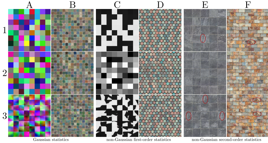
FIGURE 4.12 – Des exemples (ligne 1) synthétisés avec un CS-spot noise sans transfert d'histogramme (ligne 2), et avec un high performance noise CS + transfert d'histogramme CS (ligne 3). La nature Gaussienne de notre CS-spot noise le rend particulièrement efficace avec des exemples ayant des statistiques Gaussiennes cyclostationnaires ou proches (A, B). Notre high performance noise préserve à la place des structures non-Gaussiennes complexes (E, F), mais peut produire des répétitions visibles (entourées en rouge) et de nouvelles tuiles aberrantes (A, B, C, D).
