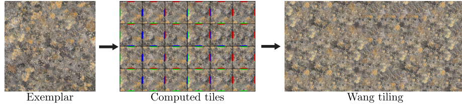
FIGURE 2.6 – Pavage de Wang tel que conçu par Cohen et al. [CSHD03]. Les tuiles sont synthétisées par quilting [EF01].
