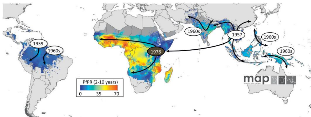
Figure 3. Emergence et dispersion de la résistance à la chloroquine chez Plasmodium falciparum .
