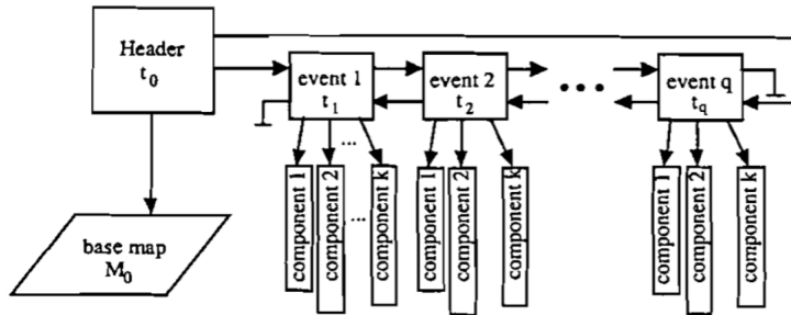
FIGURE 2.5 – La structure du modèle ESTDM est constituée d'un en-tête (header), d'une carte initiale (base map) et d'une liste d'événements (event list), l'événement étant lui-même formé de composants (components)
