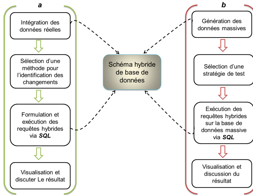
FIGURE 5.1 – Méthodologie d’expérimentation du modèle hybride
