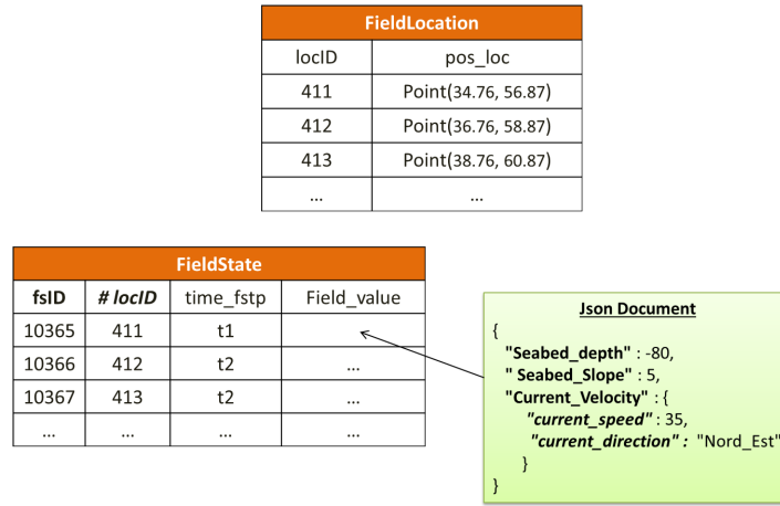
FIGURE 4.8 – Instantiation du modèle champ
