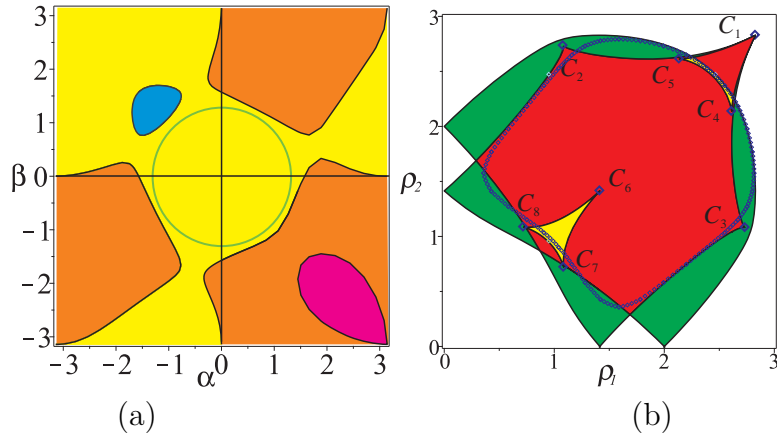
FIGURE 5.11 – Espace de travail (a) et espace articulaire (b) avec 8 points cusps à la limite de l'espace de travail souhaité et son image dans l'espace articulaire pour h = r = f = 1
