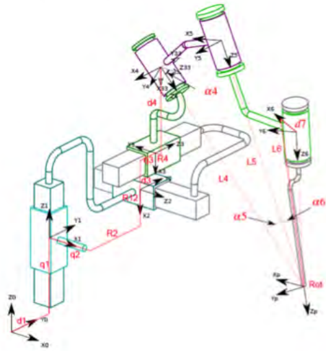
(a) Schéma de l'architecture en série du Robotol.
