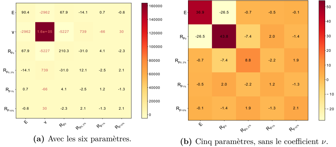
Figure 8.4 – Matrice de covariance des paramètres adimensionnés après identification, dans la configuration bilatérale.
