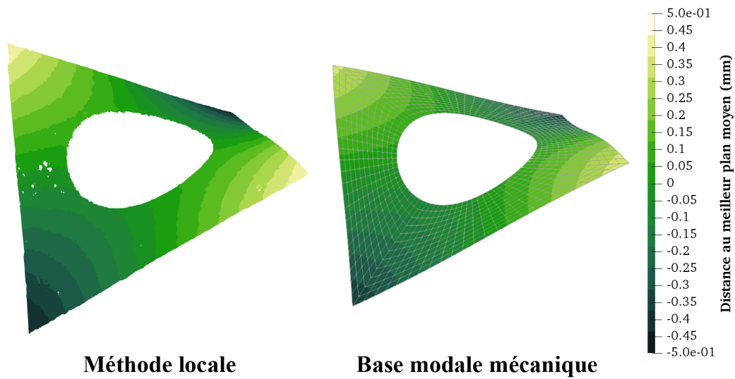
Figure 8.8 – Correction de forme à appliquer à l'éprouvette plate, mesurée par deux méthodes.
