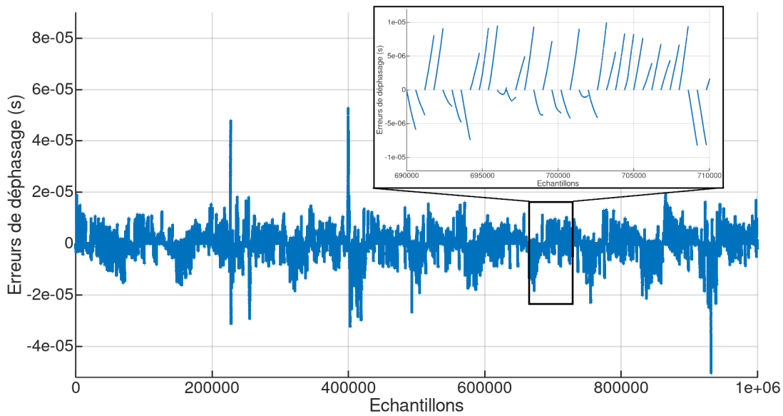
FIGURE 4.3 – Erreurs de prédiction du déphasages pour k=600 s
