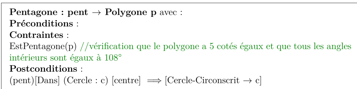
FIGURE 5.4 – Règle de production d'un pentagone en GMC-PC
