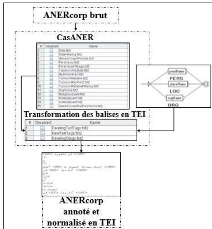
Figure 74. Architecture de la REN effectuée par CasANER sur ANERcorp brut
