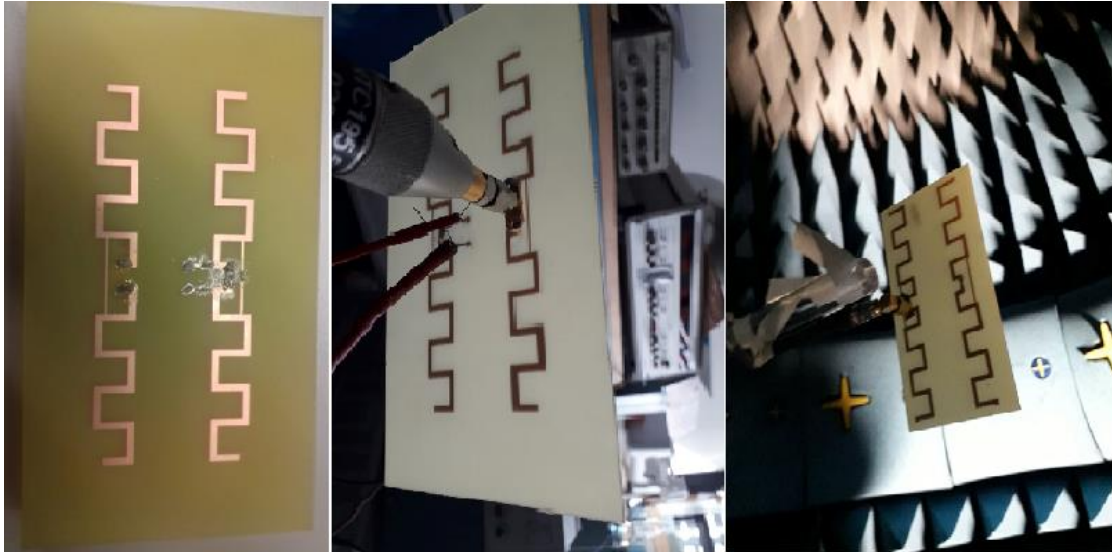
Figure 48 : Photo du prototype de l'antenne proposée
