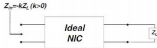
Figure 74 : Illustration du montage NIC
