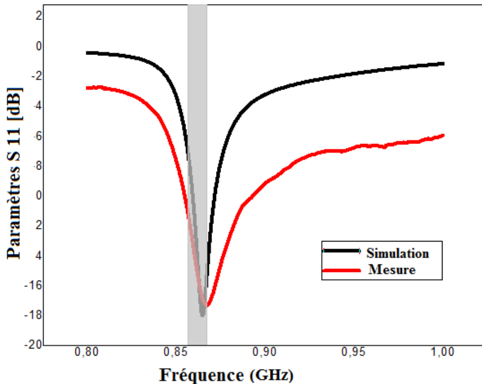
Figure 49 : Coefficient de réflexion mesuré pour Z_L = 5,6pF
