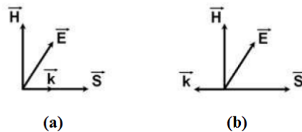
Figure I.9 . Principe des antennes composites. a) Propagation main droite, b) Propagation main gauche
