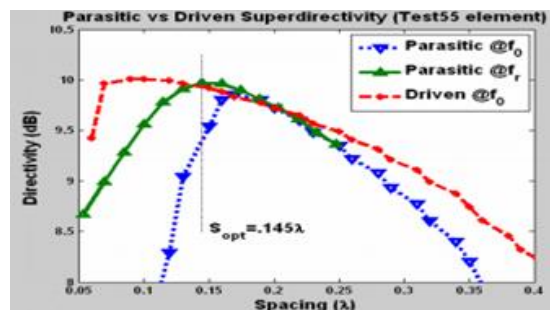
Figure I.18 : Comparaison de la directivité de deux réseaux d'antennes électriquement petites lorsque tous les éléments sont excités et dans le mode parasite (un élément excité et un élément court-circuité).
