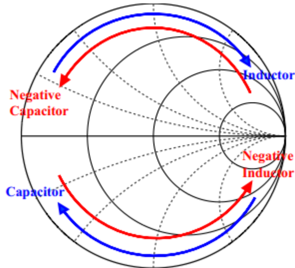
Figure 72 : Principe des composants Foster et non-Foster
