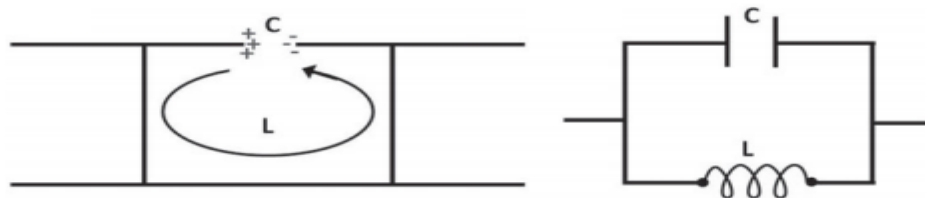
Figure I.8 : modèle de circuit LC équivalent
