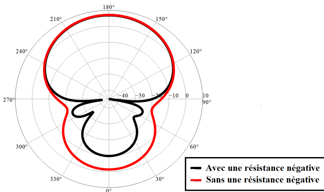
Figure 45 : Diagramme de rayonnement 2D simulé dans le plan d'azimut à 868 MHz lorsque l'antenne parasite est chargée par C = 5,6\text{pF} en série avec et sans résistance négative -5 \Omega .
