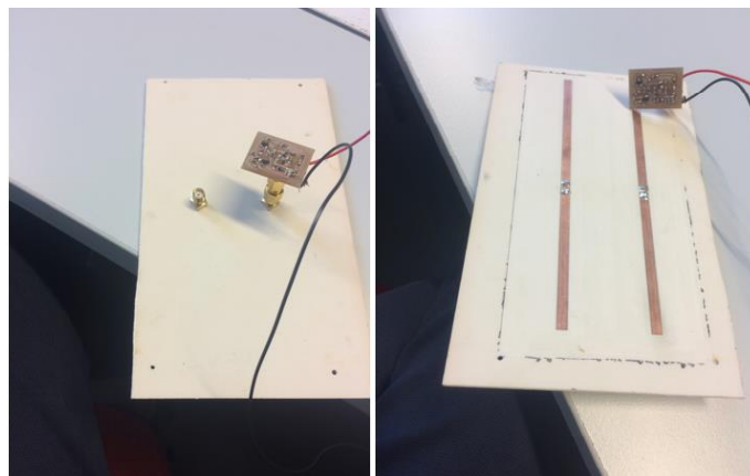
Figure 92 : Photo du prototype réalisé de l'antenne proposée
