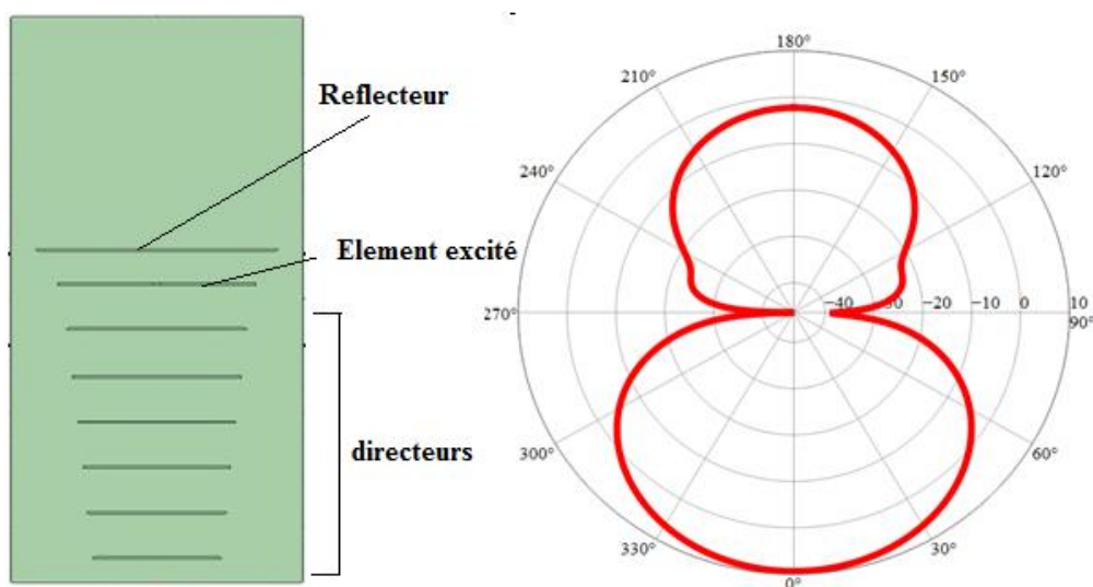
Figure 61 : Structure d'une antenne Yagi simple et le diagramme de rayonnement obtenu en simulation
