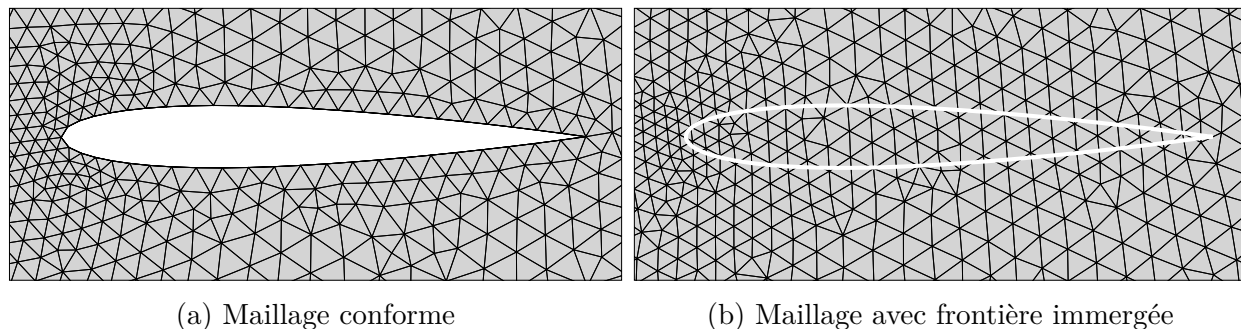
Figure B.3 Exemple de maillages non structurés conformes et frontière immergée pour un profil NACA0012 (maillage grossier pour illustration)
