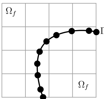
Figure B.5 Représentation des marqueurs de surface ( \Gamma ) entourés de fluide ( \Omega_f ) et immergés dans une grille cartésienne.
