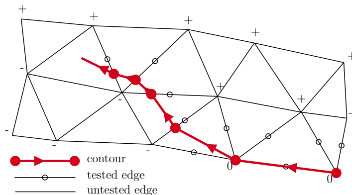
Figure B.28 Illustration du processus d'extraction de contour
