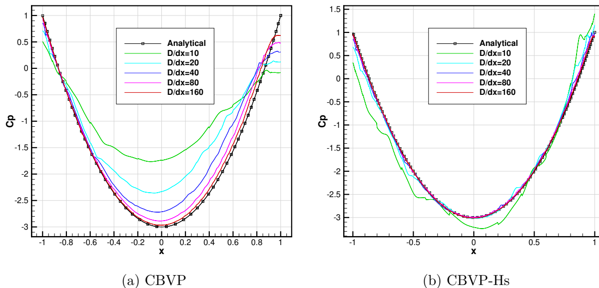
Figure B.14 Distribution de C_p sur différents raffinements de maillage pour le cas cylindre.
