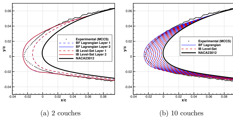
Figure B.31 Simulation multicouche pour le cas 241, givre blanc
