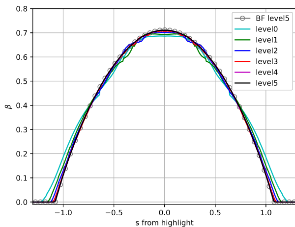
(a) Pénalisation volumique (VPSSO)
