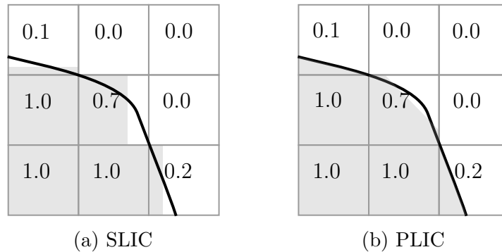
Figure B.11 Reconstruction de l'interface pour une méthode VoF
