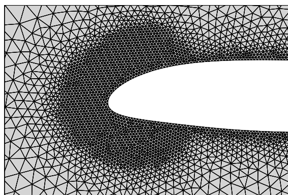
Figure B.30 Exemple de maillage pour un NACA23012 avec un raffinement de maillage étendu près du bord d'attaque.
