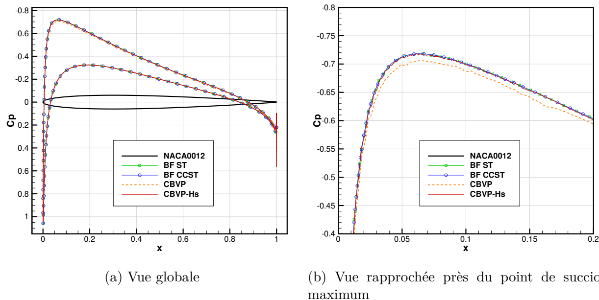
Figure B.16 Coefficients de pression pour le profil NACA0012 à Mach=0.5 et AoA=1.25deg. Comparaison entre les méthodes body-fitted et immergée.
