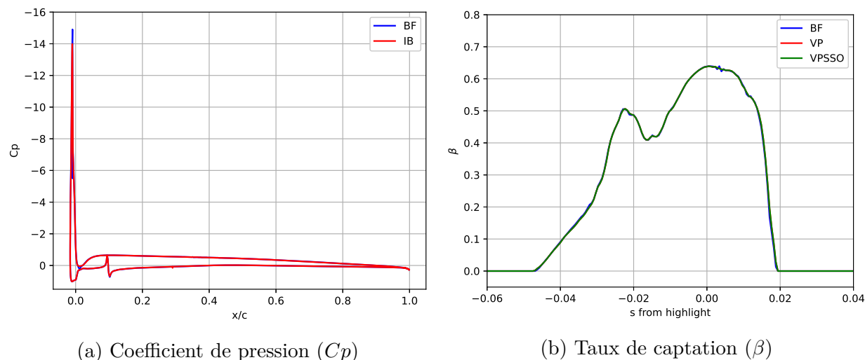
Figure B.25 Comparaison des solutions à la paroi pour la corne de glace
