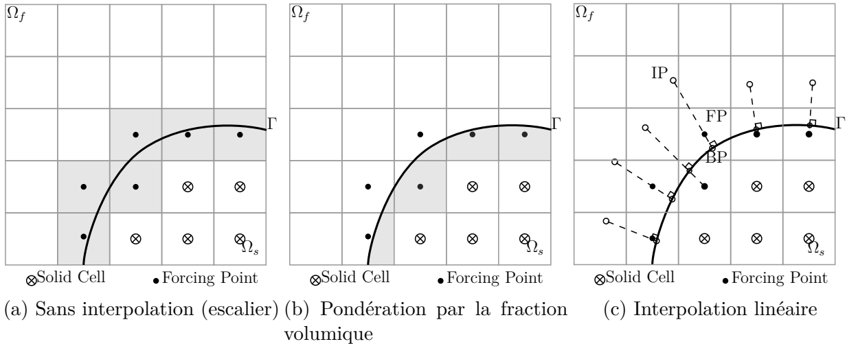
Figure B.7 Trois techniques d'interpolation pour la méthode de forçage direct
