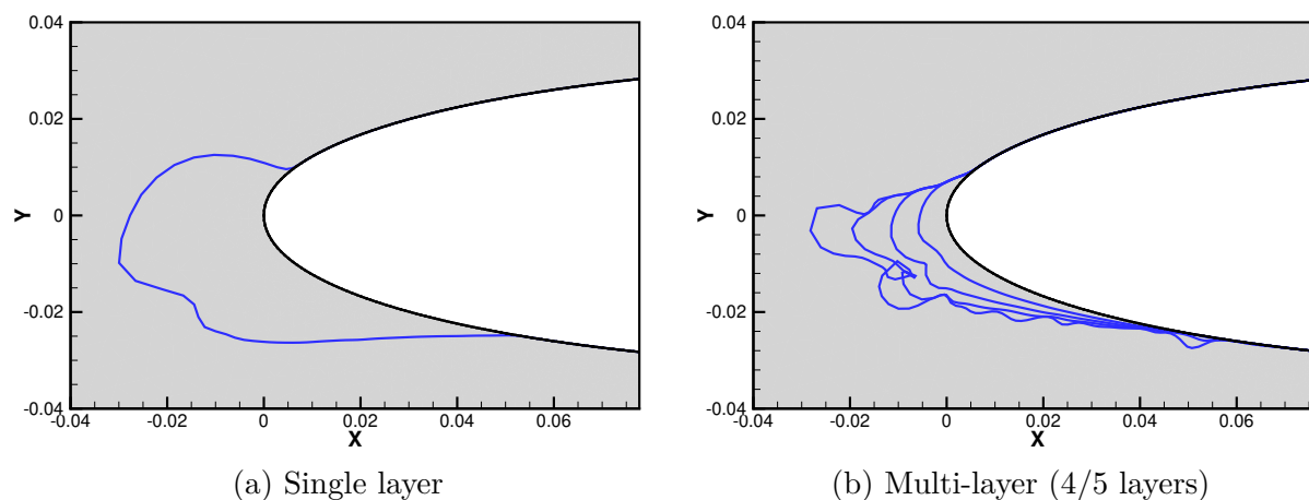
Figure B.2 Exemple d'accrétion de givre pour un cas de givre blanc
