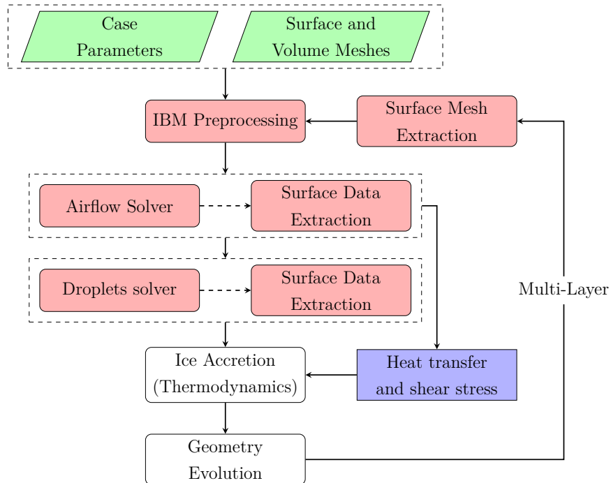
Figure B.13 Simulation de givrage multi-pas. Modifications nécessaires pour une IBM représentées en rouge
