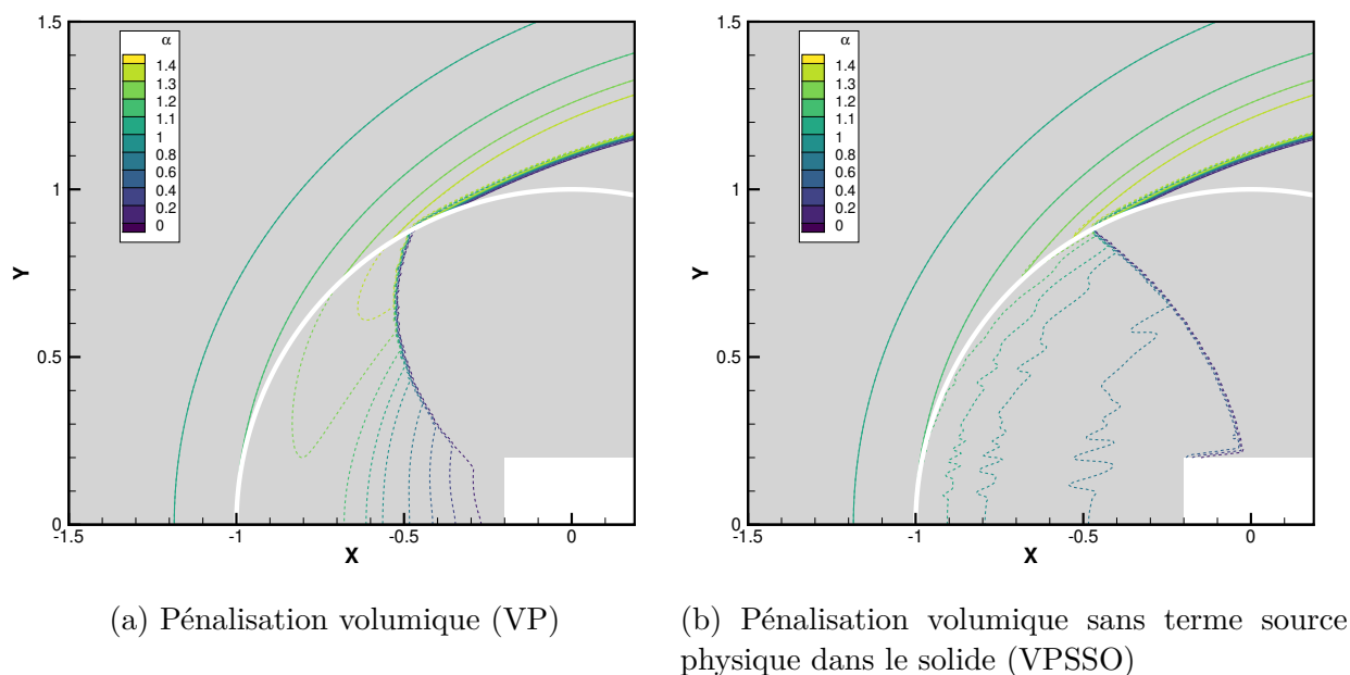
Figure B.22 Champ \alpha pour les méthodes BF et IB. Trait plein : BF, trait pointillé : IB
