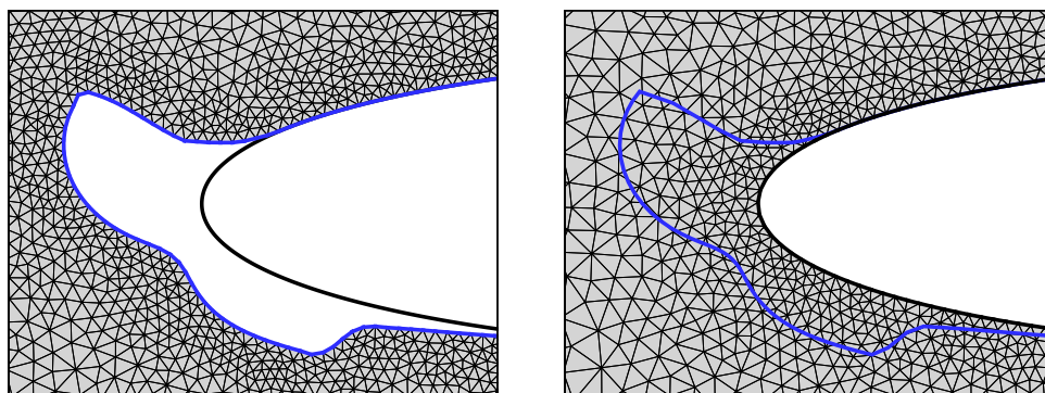
(a) Remaillage pour une approche avec (b) Maillage initial réutilisé avec la méthode de frontières immergées maillages conformes
