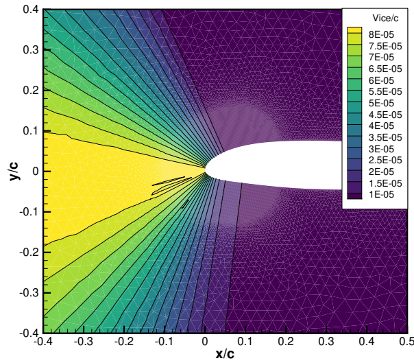
Figure B.26 Exemple de propagation du champ de vitesse
