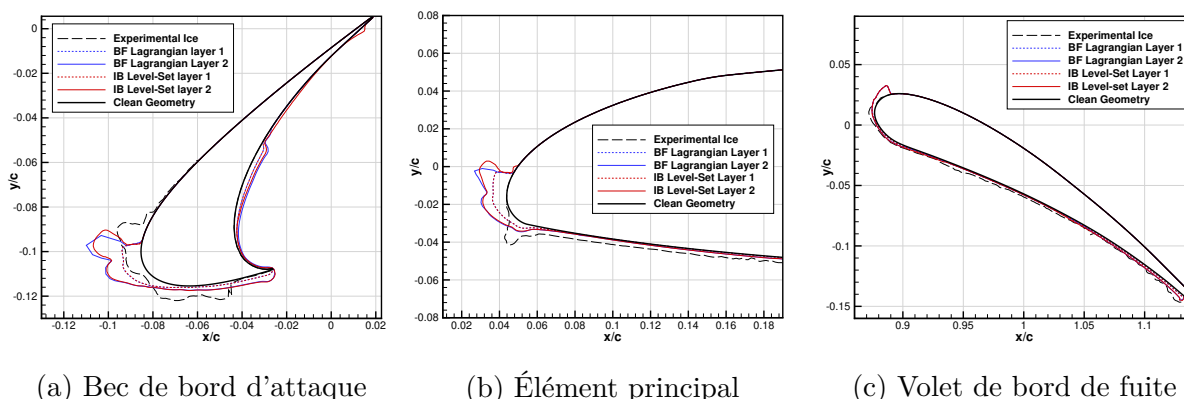
Figure B.32 Accrétion de givre sur 2 couches, profil multi élément MDA LB606b
