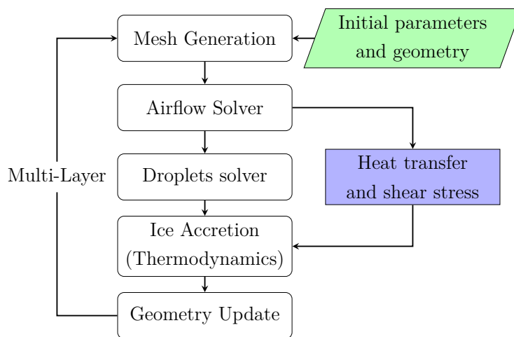
Figure B.1 Processus multicouche de givrage typique
