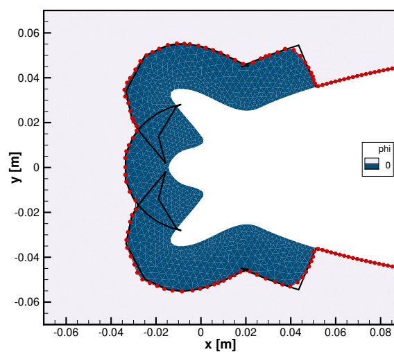
Figure B.29 Comparaison entre les approches lagrangienne et eulérienne ( level-set ).
