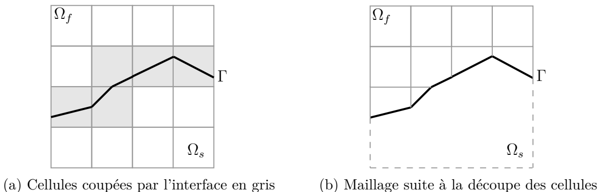
Figure B.4 Représentation de l'approche cut-cell ( \Omega_f : fluide, \Omega_s : solide, \Gamma : interface)
