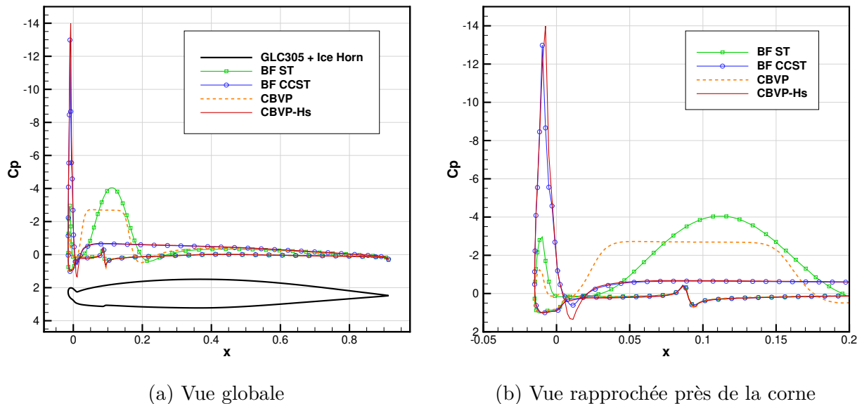
Figure B.17 Coefficients de pression à la paroi pour une corne de glace (taille de cellule près de la corne \Delta x = 2e-3 ).
