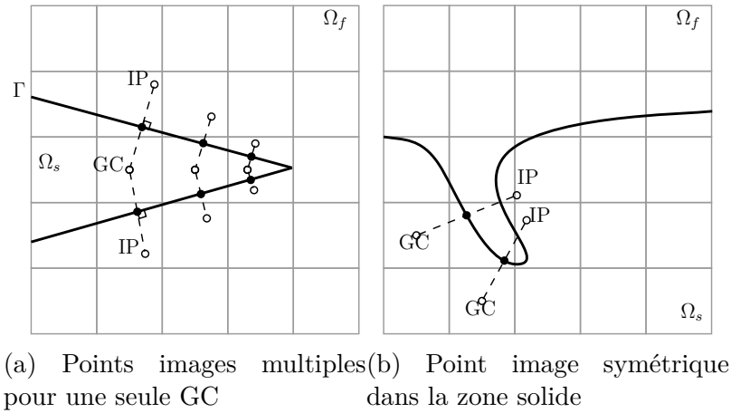
Figure B.9 Exemple de cas pathologiques pour l'approche ghost-cell
