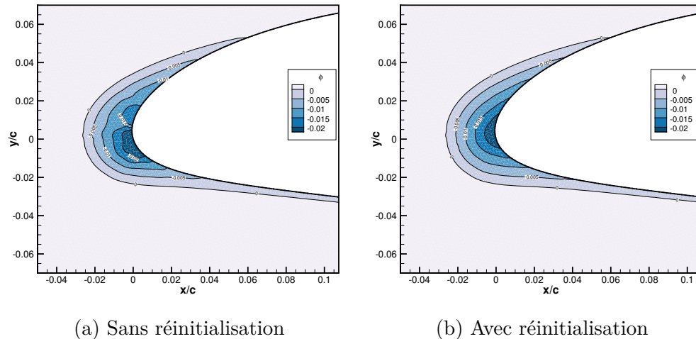
Figure B.27 Exemple de transport de level-set à partir d'un profil NACA23012 non givré
