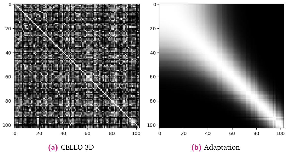
Figure 4.4.: Matrices de poids finales après les entraînements de CELLO 3D par l’algorithme décrit par LANDRY et coll. (a) et par notre adaptation (b) . Les paires de nuages de points ont un bruit gaussien croissant. Pour une paire donnée, les poids les plus forts doivent être attribués aux paires ayant un niveau de bruit similaire.
