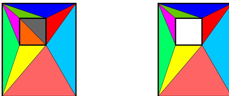
(a) Triangulation contrainte avec les arêtes des polygones externe et interne. (b) Elimination des faces dans le polygone interne.
