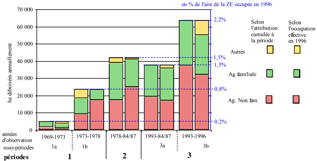
Figure 68 : Évolution du déboisement annuel; évaluation de la participation des principaux secteurs selon l'attribution des terres à la sous-période correspondant à l'année d'observation et selon l'occupation actuelle observée
