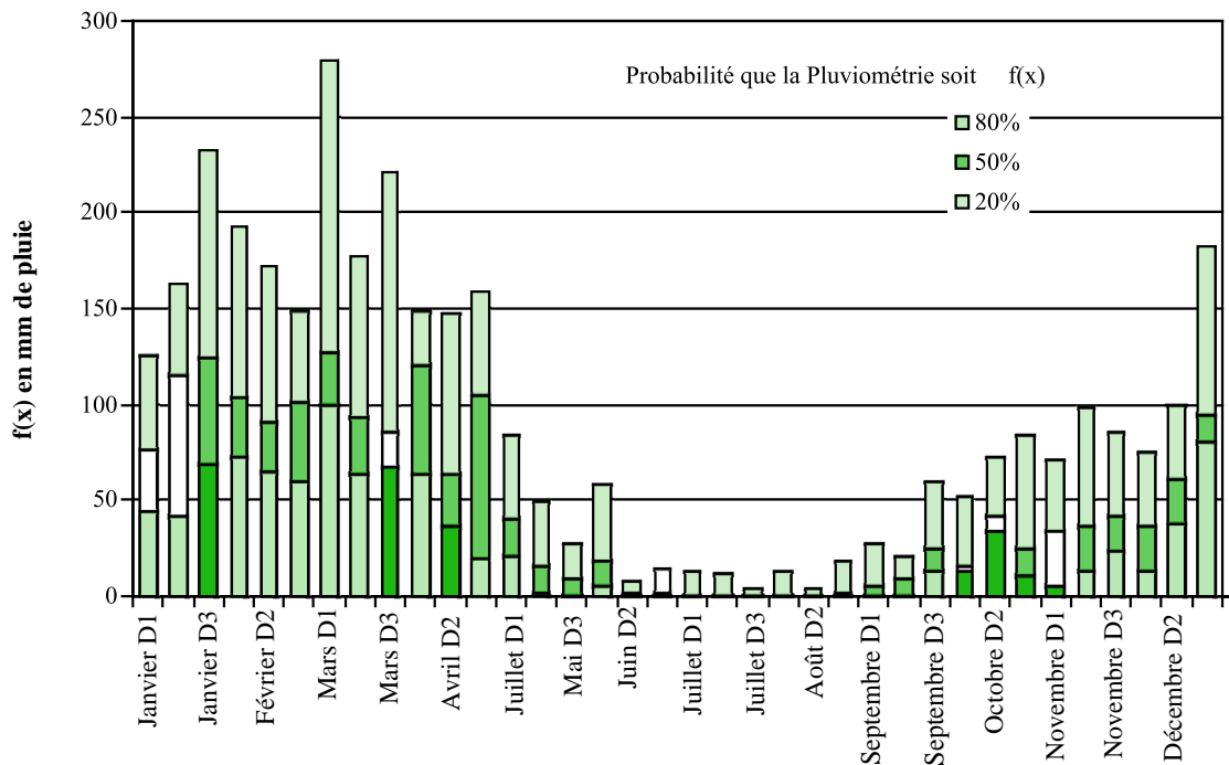
Figure 31 : Analyse fréquentielle de la pluviométrie de Marabá par décade (D) série 1973 -1997
