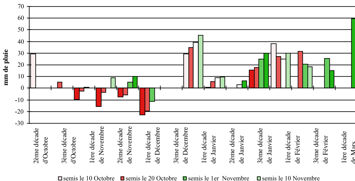
Figure 32 : Déficit et excès hydrique en fonction de la date de semis du riz
