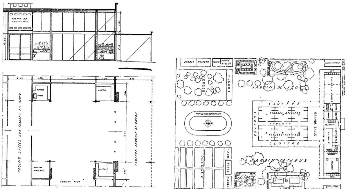
Figure 156 : Projet d'école en plein pour la "Nouvelle Éducation", Tony Fillon architecte. In Encyclopédie de l'architecture : Constructions modernes , Tome XI. Paris : Albert Morancé, 1930-1941, pl. 42.
