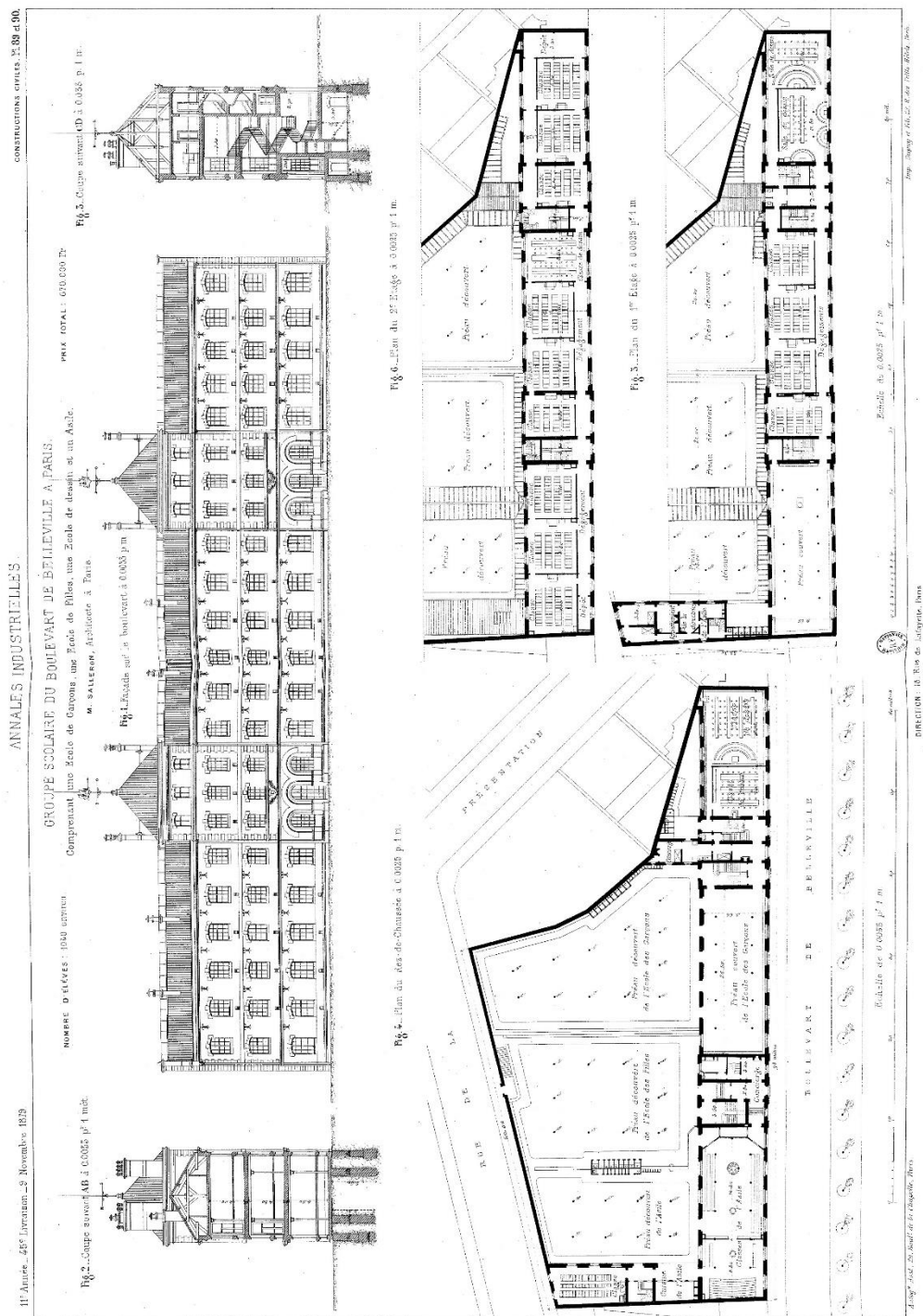
Figure 22 : Groupe scolaire du boulevard Belleville à Paris. M. Salleron, architecte à Paris. In Annales Industrielles , novembre 1879, 11 e année, 45 e livraison, pp11. 89 et 90.
