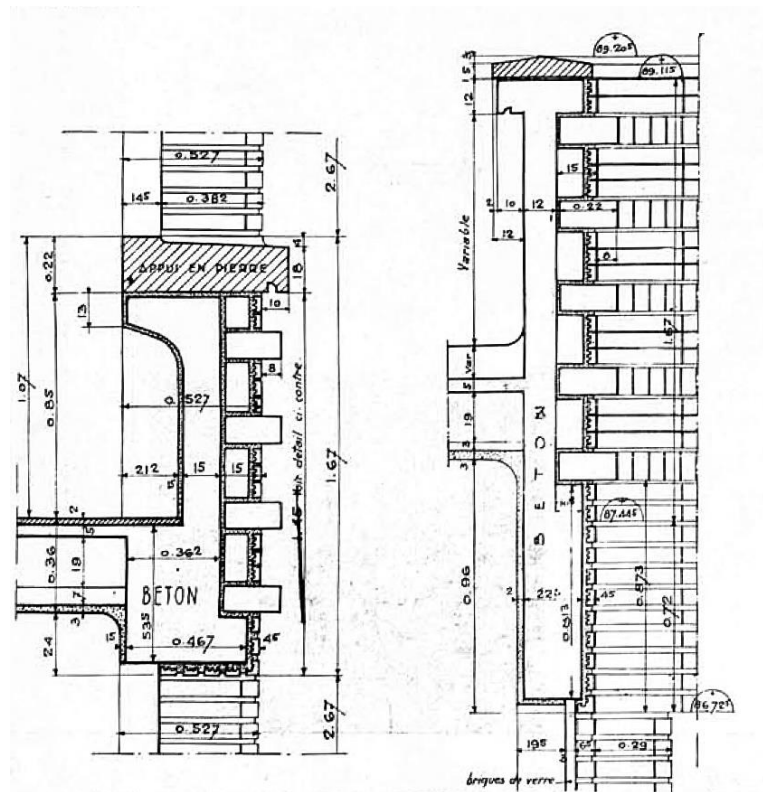
Figure 214 : Groupe scolaire Marius Jacotot, Puteaux (92), les frères Niermans architectes, 1938. In L'Architecture d'aujourd'hui , août 1938, 9 ème année, n°8, p. 14.
