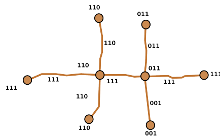
Figure 3.4: STAG associé aux trois snapshots de la figure 3.3, dont les ST-entités sont étiquetées par leur signature temporelle (d'après Benoît Costes [Cos16]).
