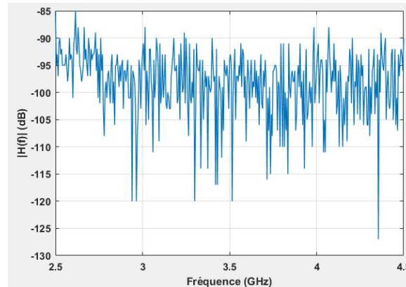
Fig. 3.1. Niveau du bruit d'entrée du VNA
