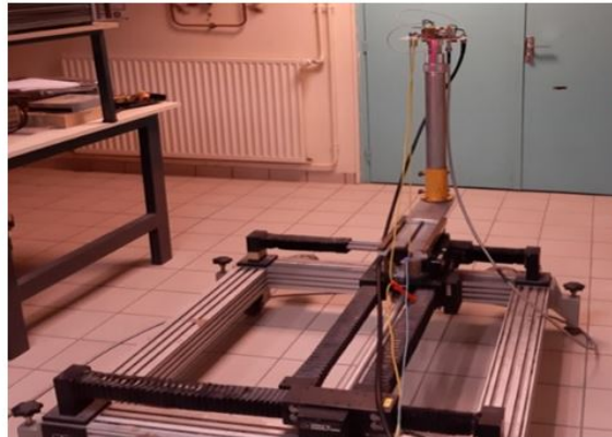
Fig. 4.3. Positionneur d’antenne
