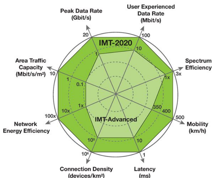
Fig. 1.2. Les principales caractéristiques des IMT-2020 par rapport à celles des IMT avancées [2][3]
