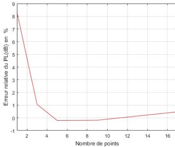
Fig. 5.12. Erreur relative de la position Rx10 en DO pour Tx au coin
