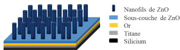
Figure 2.2. Structure idéale d’un échantillon après croissance des NFs de ZnO
