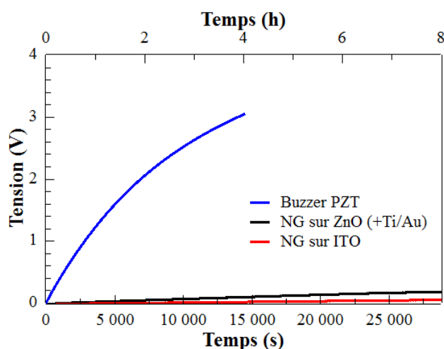
Figure 4.36 – Comparaison des profils de charge du supercondensateur par le buzzer PZT et par les deux NGs, pour une résistance de 100\text{ M}\Omega
