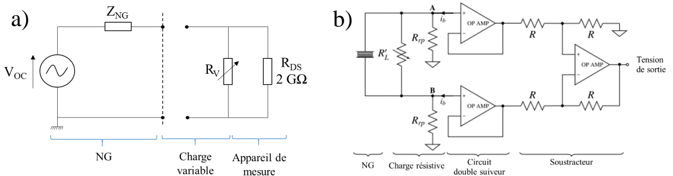
Figure 4.12- a) Circuit équivalent du NG raccordé à une charge variable avec prise en compte du circuit double suiveur et b) schéma complet du double suiveur
