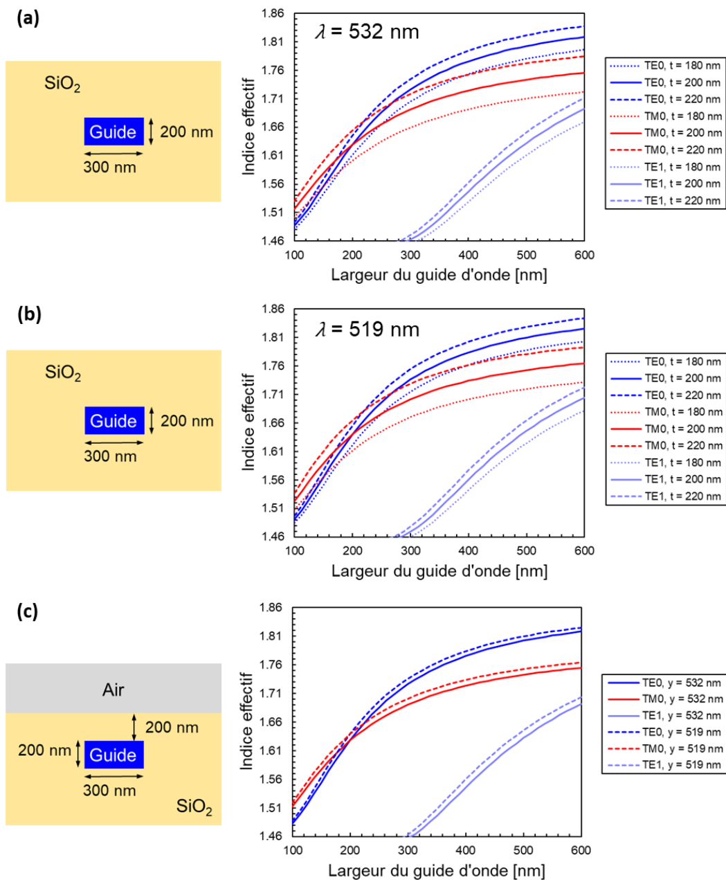
Figure 3-3 Calcul des indices effectifs pour des guides d'onde de différentes épaisseurs t à l'aide de simulations numériques FemSIM dans RSoft lorsque a) \lambda = 532 \text{ nm} et l'encapsulation est « infinie », b) \lambda = 519 \text{ nm} et l'encapsulation est « infinie », c) le guide a une épaisseur 200 nm (valeur nominale) et une encapsulation de 200 nm ( \lambda = 519, 532 \text{ nm} ) correspondant aux conditions réelles de fabrication. Les schémas à gauche représentent l'environnement de simulation (pas à l'échelle) pour le guide aux dimensions nominales.
