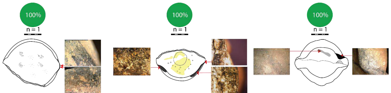
Figure 167 : Les dépôts de suie sur les lampes de types MU 7, 7 bis et 7 ter (de gauche à droite).
