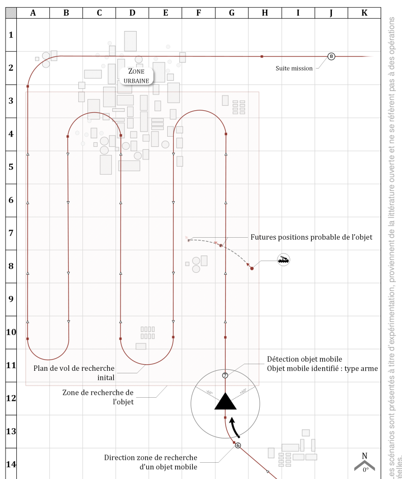
FIGURE 4.4 – Phase de recherche de l'objet mobile dans la zone.
