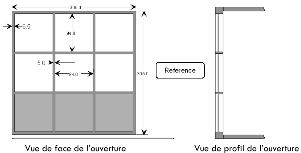
FIGURE II.35. POSITIONNEMENT ET DIMENSIONS (EN MM) DES OUVERTURES DE LA MAQUETTE EXPERIMENTALE DE L'EPFL
