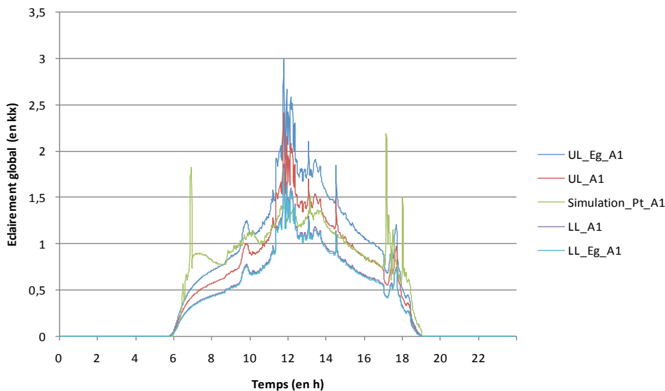
FIGURE II.55. ECLAIREMENT INTERIEUR : JOURNEE TYPE INTERMEDIAIRE SANS DIRECT DU SOLEIL
