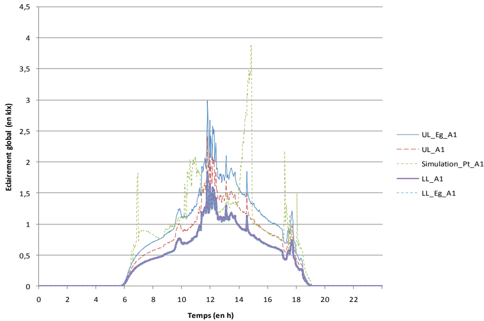
FIGURE II.54. ECLAIREMENT INTERIEUR : JOURNEE INTERMEDIAIRE AVEC DIRECT DU SOLEIL
