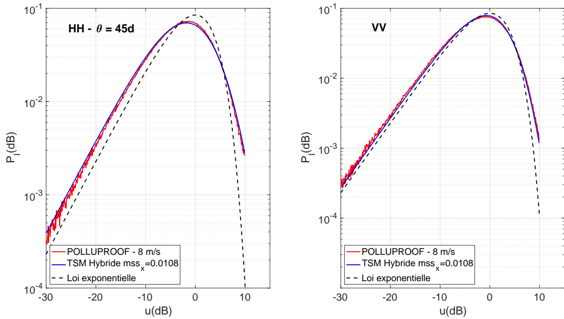
FIGURE 4.47: Distribution des intensités des données POLLUPROOF vol 1 ( U_{10} = 8\text{m/s} , H_s = 0.5\text{m} ), avec le modèle "TSM Hybride" ( m_{ss_x} = 0.0108 ) puis la loi exponentielle
