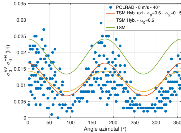
FIGURE 4.34: Différence de polarisation suivant les données POLRAD (8.5 m/s) (●) le modèle TSM (-), le modèle "TSM Hybride" (-) et le modèle "TSM Hybride azimutal" (-) en fonction de l'angle azimutal
