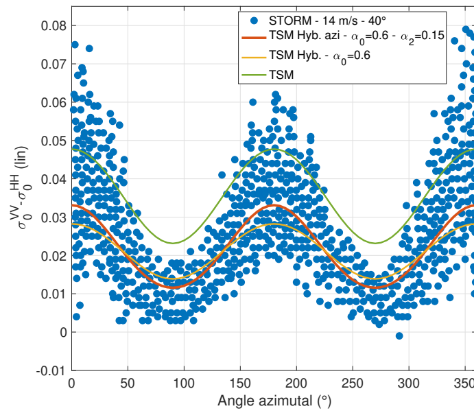
FIGURE 4.31: Différence de polarisation suivant les données STORM (14 m/s) (•) le modèle TSM (-), le modèle "TSM Hybride" (-) et le modèle "TSM Hybride azimuthal" (-) en fonction de l'angle azimutal
