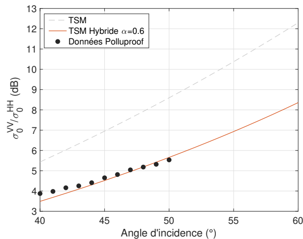
FIGURE 4.19: Rapport de polarisation omnidirectionnel des données POLLUPROOF (8 m/s) ( \bullet ), du modèle TSM ( - - ), du modèle "TSM Hybride" ( - )
