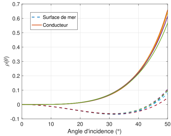
FIGURE 4.52: Évolution de la différence relative de \rho = (PR - PR_{Th})/PR en fonction de l'angle d'incidence pour 9 valeurs de \alpha entre 0.6 et 0.95. La ligne solide correspond au cas conducteur, et les pointillés à la permittivité diélectrique de la surface de mer.
