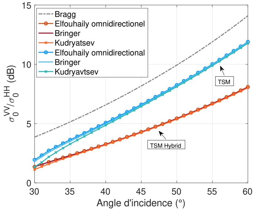
FIGURE 4.11: Rapport de polarisation du modèle TSM et "TSM Hybride" pour différents spectres : Spectre de Bringer, spectre d'Elfouhaily omnidirectionnel et spectre de Kudryatsev. Pour ces simulations nous avons choisi : un vent de 10 m/s avec une mss_x = 0.0124 isotrope, un angle d'incidence de 45^\circ , une distribution Gaussienne anisotrope et une bande de fréquence de 10 GHz (Bande X)
