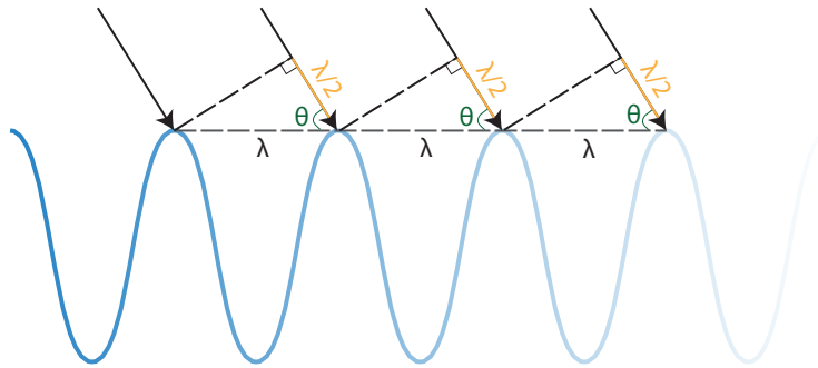
FIGURE 2.6: Représentation schématique de la diffusion de Bragg
