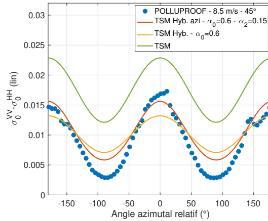
FIGURE 4.33: Différence de polarisation suivant les données omnidirectionnelles POLLUPROOF (8.5 m/s) (●) le modèle TSM (-), le modèle "TSM Hybride" (-) et le modèle "TSM Hybride azimutal" (-) en fonction de l'angle azimutal
