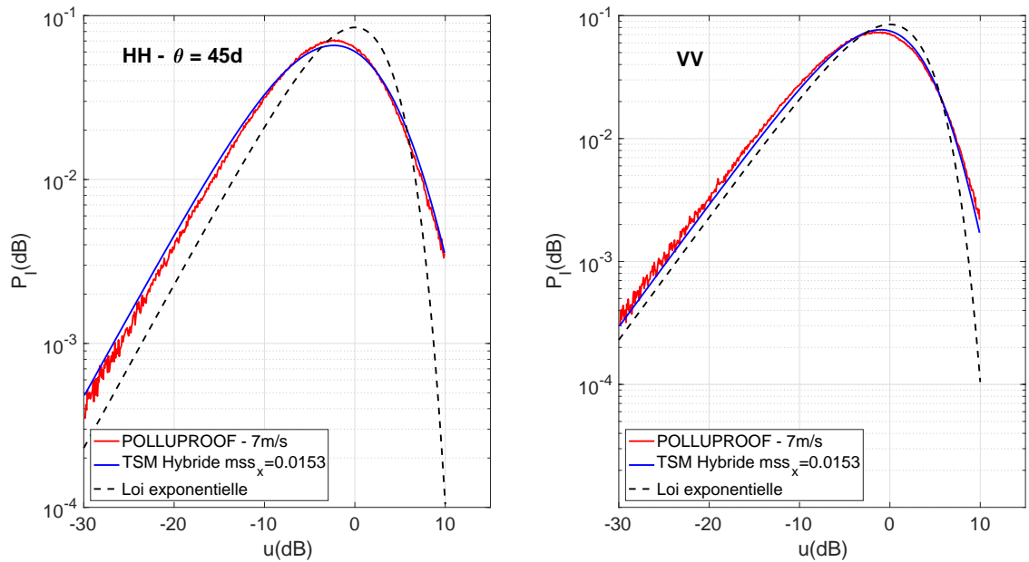
FIGURE 4.48: Distribution des intensités des données POLLUPROOF vol 2 ( U_{10} = 7\text{m/s} , H_s = 2\text{m} ), avec le modèle "TSM Hybride" ( m_{ss_x} = 0.0153 ) puis la loi exponentielle
