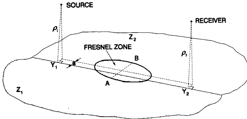
FIGURE 1.10 – Illustration de la zone de Fresnel, déterminée pour une géométrie source-récepteur donnée en présence d'une discontinuité des propriétés du sol (issue de Hothersall et Harriott, 1995).
