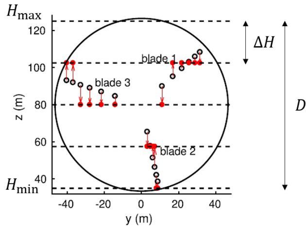
FIGURE 2.7 – Positions exactes (○) et fictives (●) des hauteurs de source distribuées le long des pales, pour la position angulaire \Phi = 48^\circ , avec S = 6 segments et N_h = 5 hauteurs de source fictives représentées par les lignes en pointillé ( \Delta H = 22.5m ). La figure est issue de Cotté [2019]
