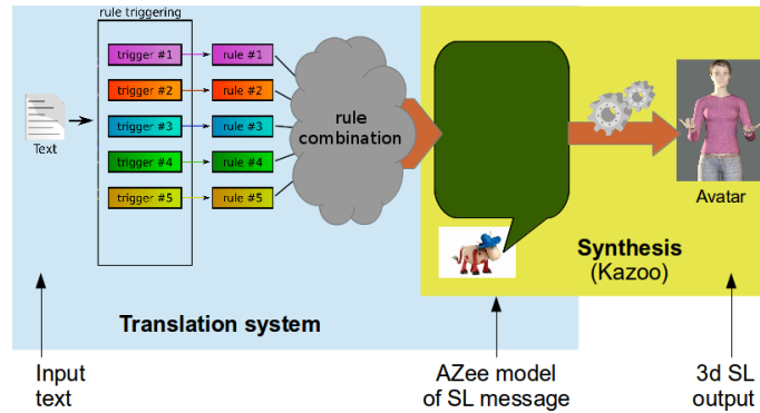
FIGURE 22 – Architecture pour la traduction automatique avec AZee comme pivot
