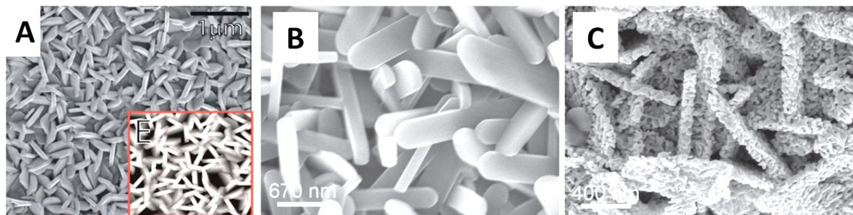
Figure Perspectives.7 (A) \text{V}_2\text{O}_5 nanostructuré déposé par ALD à partir de \text{VO}(\text{thd})_2 et d' \text{O}_3 227 et poudre de \text{V}_2\text{O}_5 avant (A) et après (B) un recuit sous \text{NH}_3 , formant ainsi du VN tout en gardant la structure du \text{V}_2\text{O}_5 119
