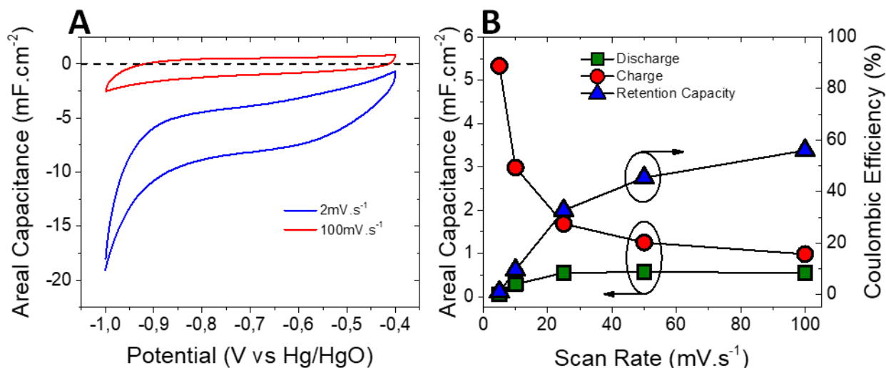
Figure VI.11 (A) CV du dépôt de 120 nm de VN par ALD et (B) évolution de la capacité de charge/décharge et de l'efficacité coulombique en fonction de la vitesse de de balayage
