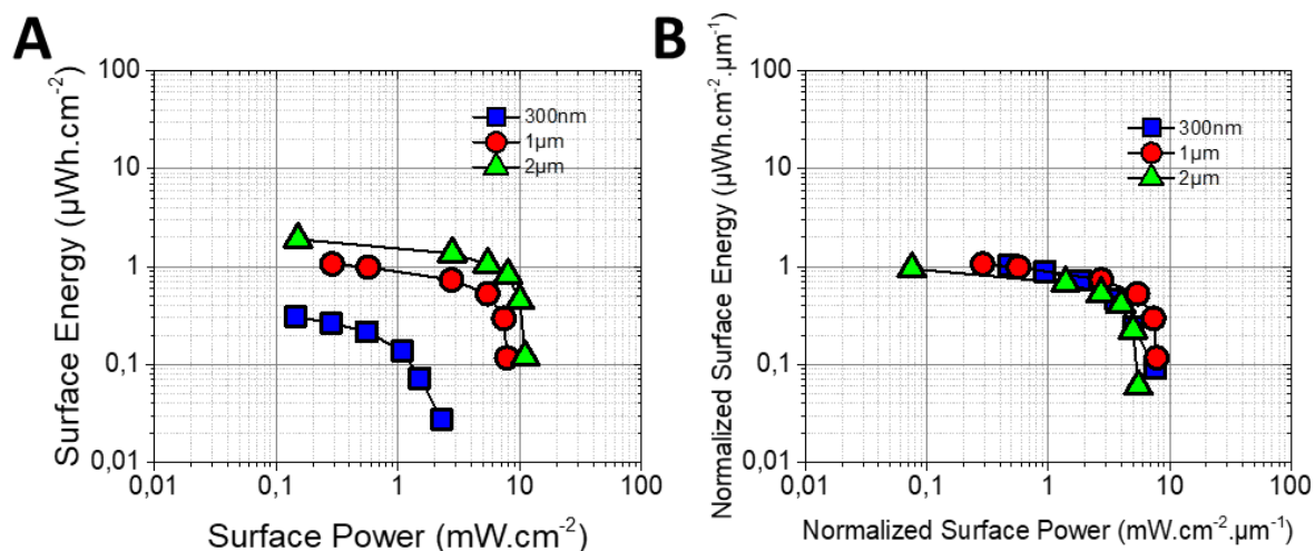
Figure V.20 (A) diagramme de Ragone et (B) diagramme de Ragone normalisé par l'épaisseur des électrodes pour une configuration interdigitée
