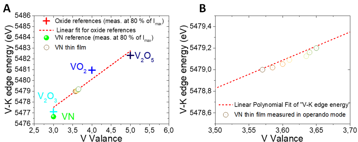
Figure IV.15 (A) Décalage de seuil d'absorption du vanadium en fonction de sa valence et (B) zoom sur les décalages du vanadium lors du cyclage d'une électrode VN
