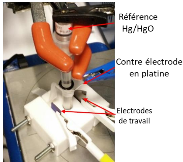
Figure V.2 Photographie d'un montage face / face pour tests électrochimiques
