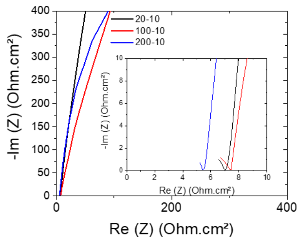
Figure V.15 PEIS de dispositif dont la largeur des doigts est variée
