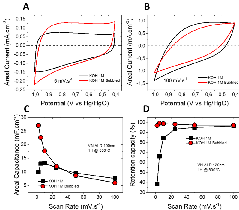
Figure VI.14 CV a 5 mV.s -1 (A) et 100 mV.s -1 (B), capacité de décharge (C) et efficacité coulombique (D) en milieux KOH 1M et KOH 1M bullé d'un film de 120 nm de VN déposé par ALD et recuit à 800 °C sous azote pendant 1h.
