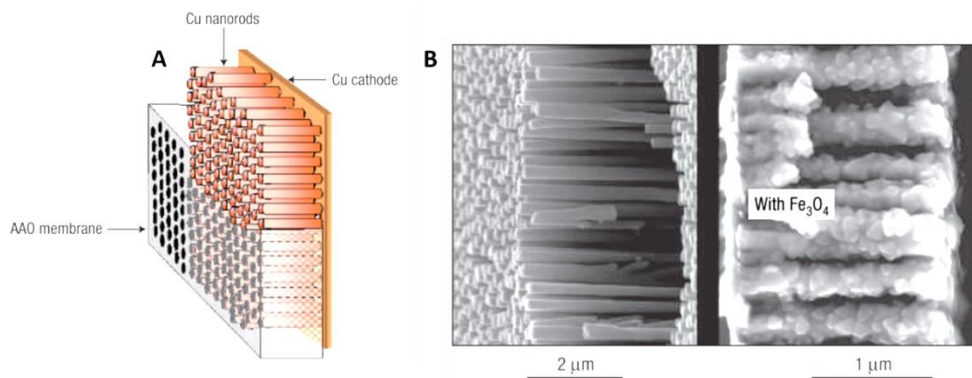
Figure VI.2 (A) Réalisation de nanopiliers de cuivre par template et (B) images MEB des nanopiliers après retrait de la membrane et après dépôt de Fe 3 O 4 par électrodéposition 197
