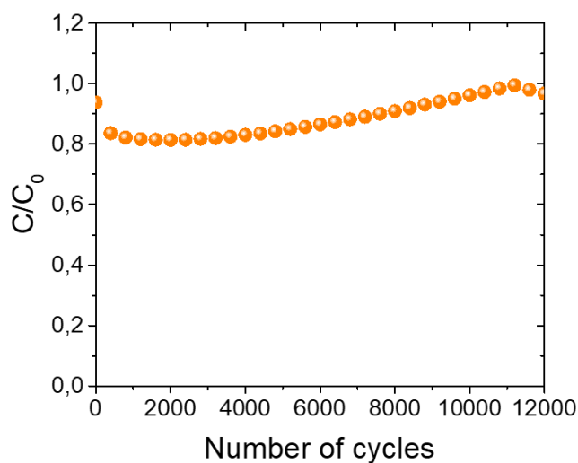
Figure V.21 Capacité de rétention d'un MSC composé de deux électrodes interdigitées de 1 \mu\text{m} d'épaisseur.
