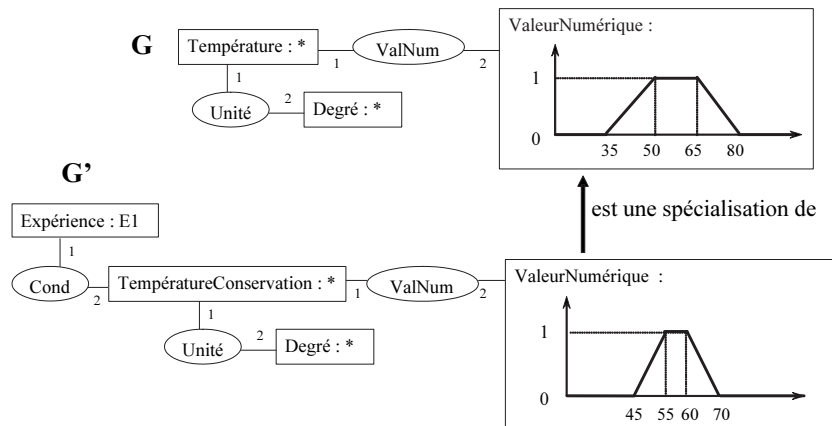
Fig. 4.8 – Un exemple de projection d’un graphe G dans un graphe G' faisant intervenir des marqueurs flous.
