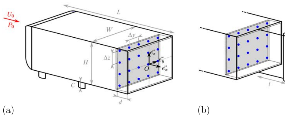
FIGURE 3.5 – Montage du corps d’Ahmed avec cavité et barreau d’Evrard et Cadot pour suppression passive de la bistabilité latérale (Evrard et al., 2016).
