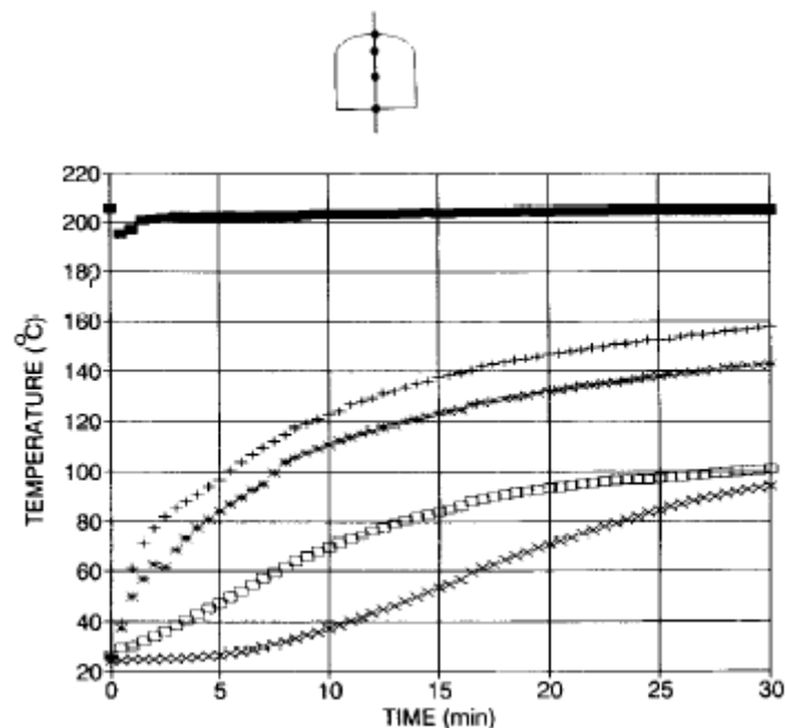
Figure 18 : Variations des températures pendant la cuisson de pain: température du four (■), température surface pâte à pain (+), température de la surface au contact du support(*), à 1 cm sous la surface haute (□) et dans la mie (x) (Zanoni et al, 1993).
