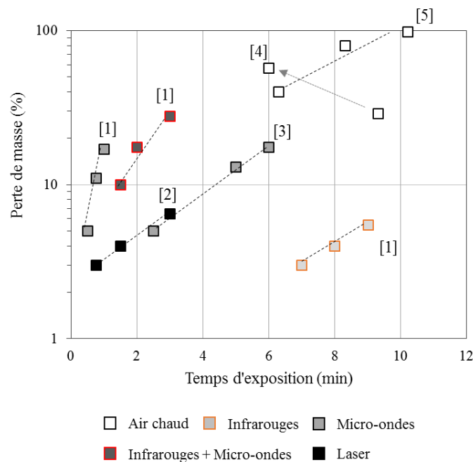
Figure 7 : Perte de masse (%) de pâtes céréalieres en fonction du temps d'exposition pour différentes techniques de chauffe. D'après les données de [1] : Ozge-Keskin et al., 2004; [2] : Blutinger et al., 2019 ; et [3] : Sumnu et al., 1999, [4] : Baik et Marcotte, 2002 ; [5] : Sakin et al., 2007.
