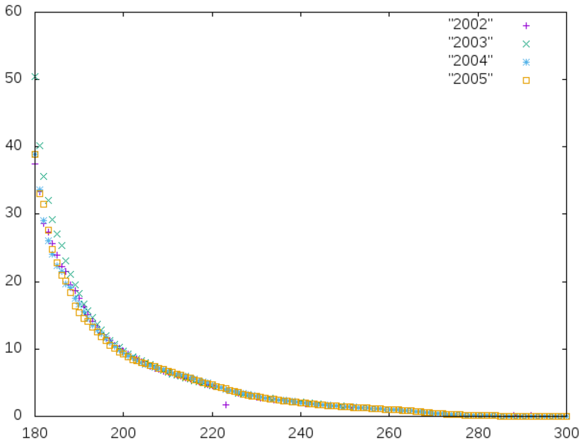
Figure 2.4.4.a: Intensité moyenne de précipitation (mm/h) en fonction de la température de brillance (K) à 10.8 \mu\text{m} . Courbes tracées pour quatre années successives.
