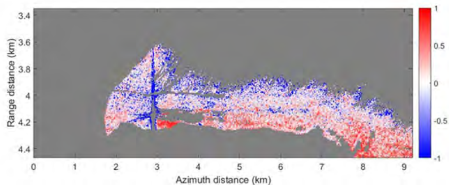
Fig. 42 : Image du paramètre M (Mixing Index) estimée sur les données SAR acquises en bande L par SETHI lors de l'exercice NOFO-2015 – déversement d'hydrocarbures – 09 juin 2015 10:02 UTC.
