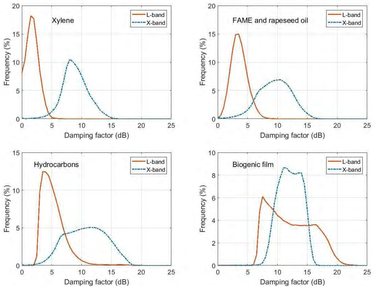
Fig. 45 : Histogrammes des valeurs de Damping Ratio mesurées en bande X (trait pointillé bleu) et en bande L (trait rouge) sur des nappes de xylène, de FAME, d'huile de colza, d'hydrocarbures et d'huile biogénique
