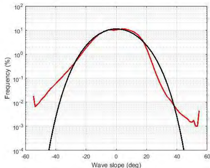
Fig. 28 : Distributions des pentes pour un cas Gaussien de référence (courbe noire) et pour les mesures en souffleries [68] (courbe rouge)
