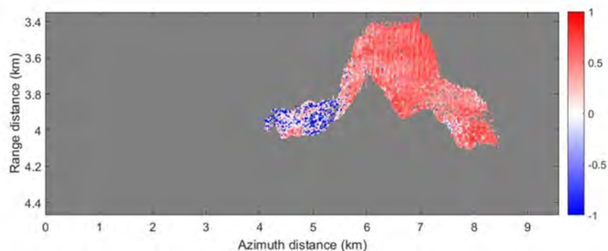
Fig. 41 : Image du paramètre M (Mixing Index) estimée sur les données SAR acquises en bande L par SETHI lors de l'exercice POLLUPROOF-2015 – déversement de FAME et d'huile de colza – 22 mai 2015 16:07 UTC.
