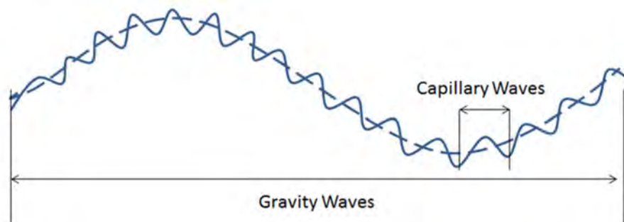
Fig. 17 : Profil de la surface océanique
