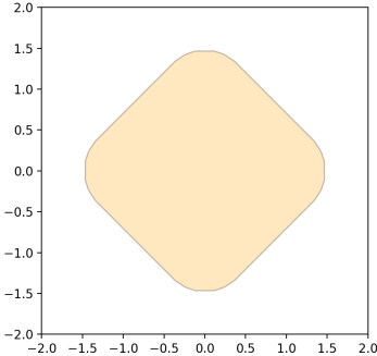
(d) Lovasz distance with f_2
