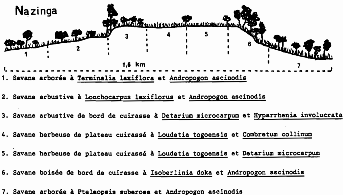
FIGURE II.3. Deux exemples de la répartition de la végétation en fonction de la topographie en Afrique de l'Ouest: Ouango-Fitini en Côte d'Ivoire (d'après FOURNIER et al., 1982) et Nazinga au Burkina Faso (d'après OUEDRAOGO, 1985).
