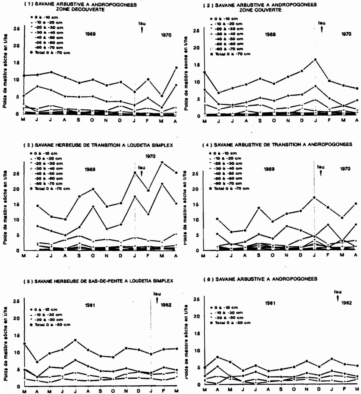
FIGURE X.11. Cycle saisonnier de la phytomasse des racines dans six faciès des savanes de Lamto (06°13'N, 05°02'W) en Côte d'Ivoire, d'après CESAR (1971 b) et ABBADIE (1983).
