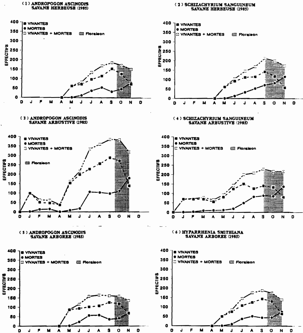
FIGURE VII.2. Evolution saisonnière des effectifs de feuilles chez trois espèces de Graminées pérennes des savanes de Nazinga au Burkina Faso.
