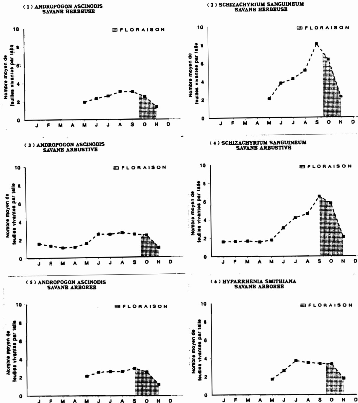
FIGURE VII.5. Evolution saisonnière du nombre moyen de feuilles par talle chez trois espèces de Graminées pérennes des savanes de Nazinga au Burkina Faso.
