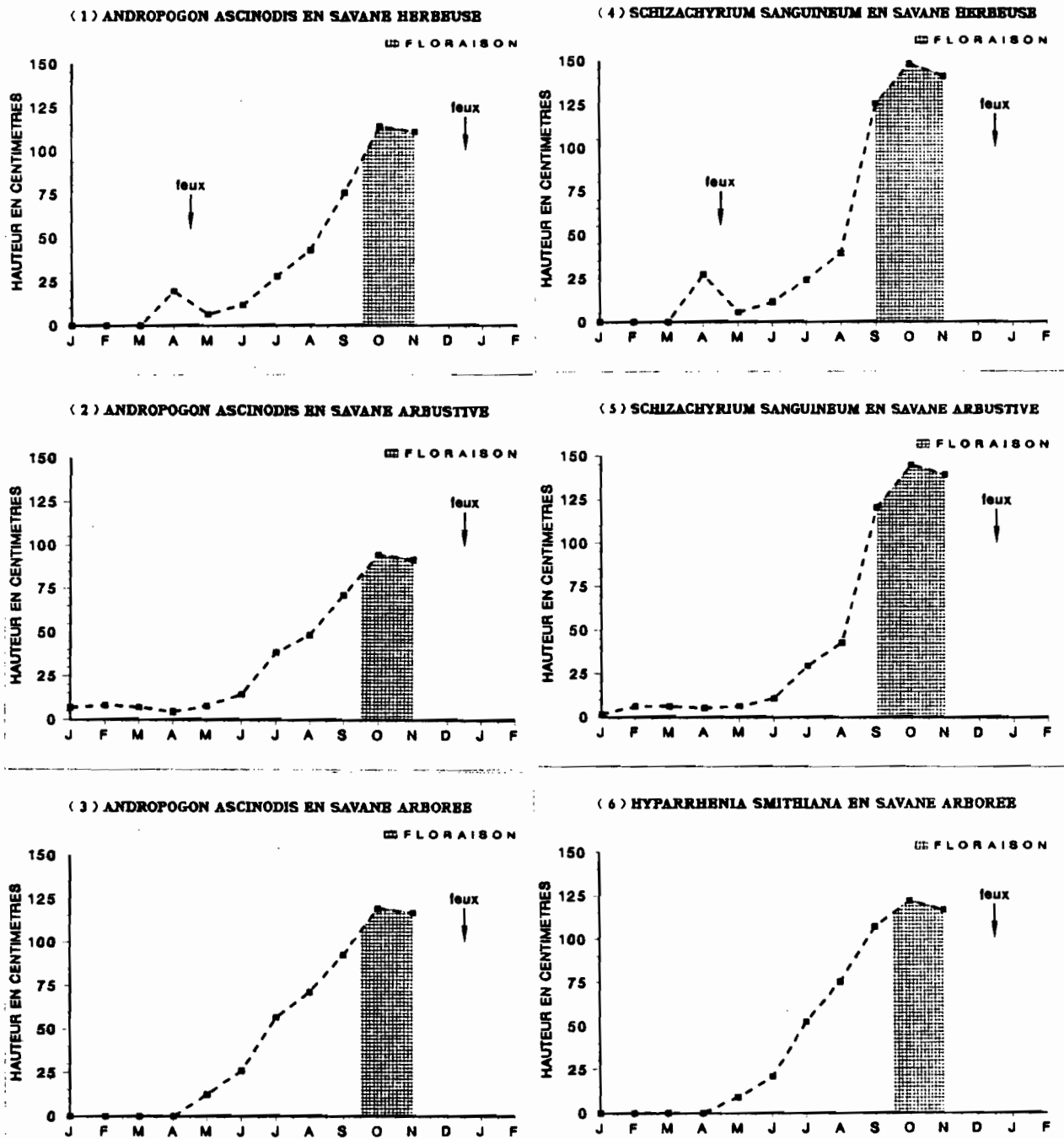
FIGURE IV.1. Croissance en hauteur de quelques Graminées pérennes à Nazinga (11° 09' 36"N, 01° 36' 00"W) en 1985.
