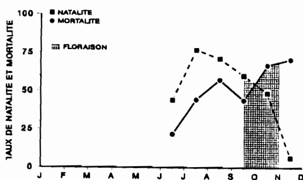
FIGURE VII.7. Evolution saisonnière de la natalité et de la mortalité dans les populations de feuilles de trois espèces de Graminées pérennes des savanes de Nazinga au Burkina Faso en 1985.
