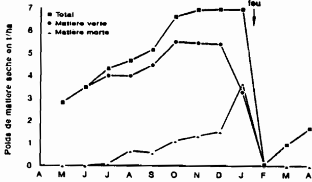
( 7 ) SAVANE HERBEUSE A LOUDETIA SIMPLEX CYCLE DES PHYTOMASSES
