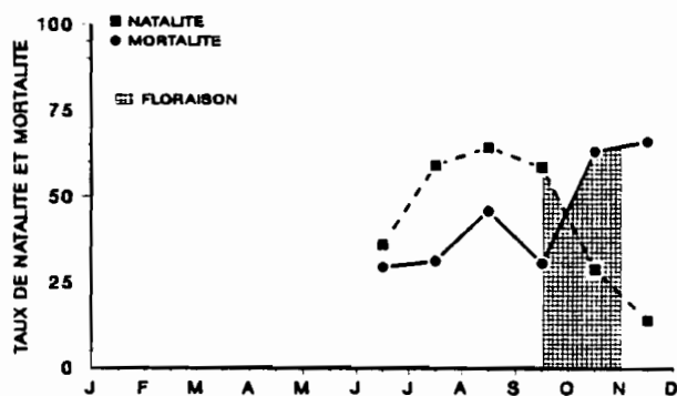
(3) ANDROPOGON ASCINODIS EN SAVANE ARBUSTIVE
