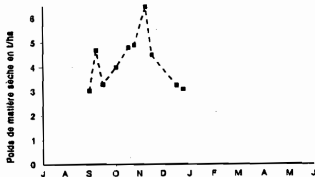
FIGURE X.1. Variation saisonnière de la phytomasse herbacée aérienne dans trois faciès des savanes de Gampéla (12°25'N, 01°22'W) au Burkina Faso, d'après N'GARSARI (1983).
