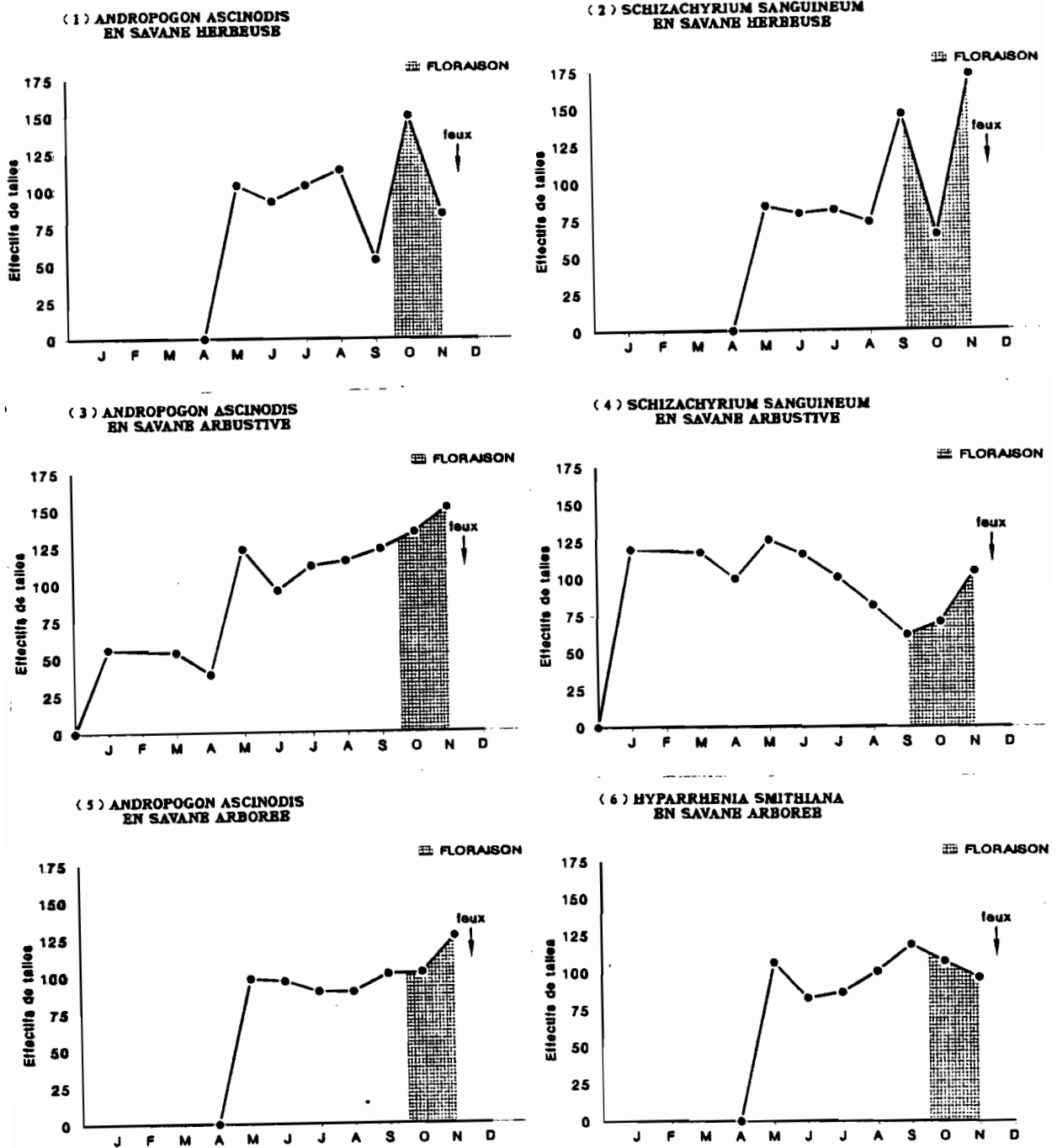
FIGURE VII.4. Variation saisonnière de l'effectif des talles chez trois espèces de Graminées pérennes des savanes de Nazinga au Burkina Faso.
