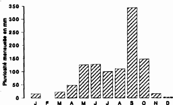
(5) PLUVIOSITE MENSUELLE A OUANGO-FITINI EN 1977 TOTAL 964 mm
