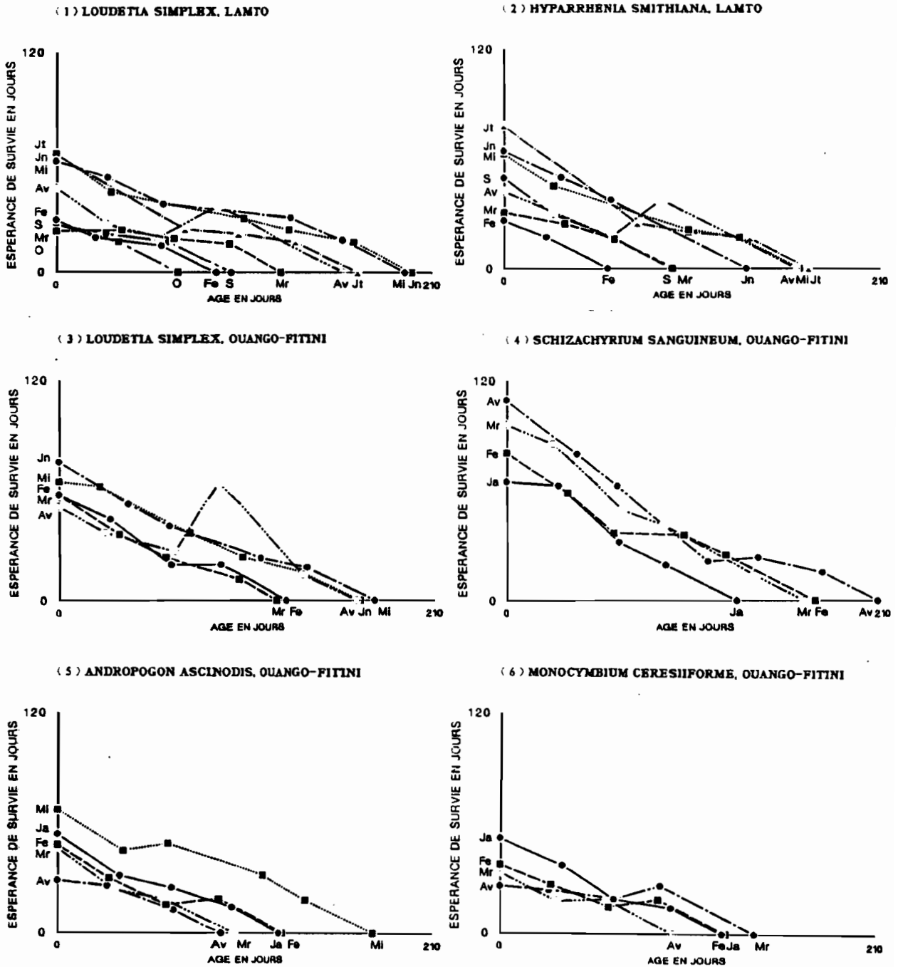
FIGURE VII.12. Espérance de survie des cohortes successives de feuilles chez cinq espèces de Graminées pérennes des savanes de Côte d'Ivoire en 1980 (d'après FOURNIER, 1982, a, 1983 a, 1984).
