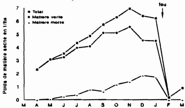
( 9 ) SAVANE HERBEUSE A LOUDETIA SIMPLEX CYCLE DES PHYTOMASSES
