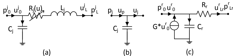
Figure 2.6 - Circuit électrique équivalent à (a) un échangeur, (b) une chambre et (c) un régénérateur
