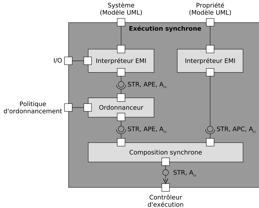
FIGURE 9.3 – Composant d'exécution de modèles avec composition synchrone.
