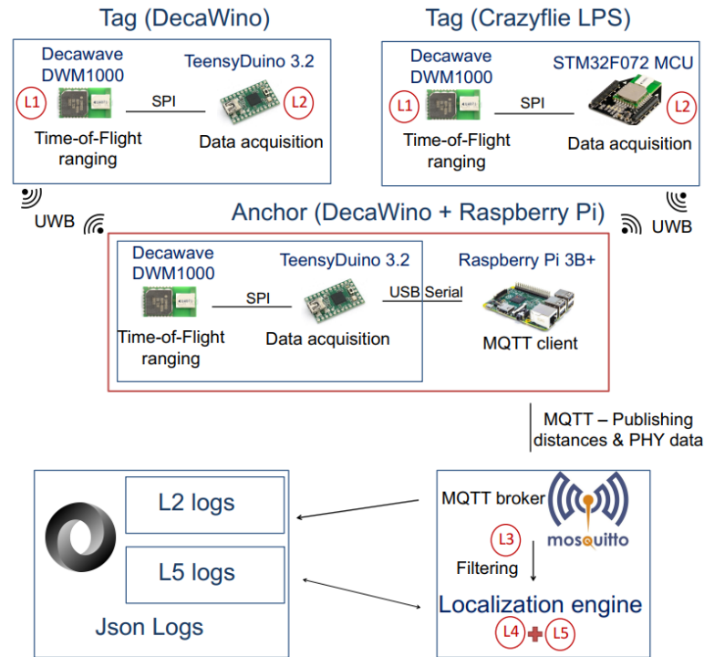
Fig. 12. SecureLoc Architecture
