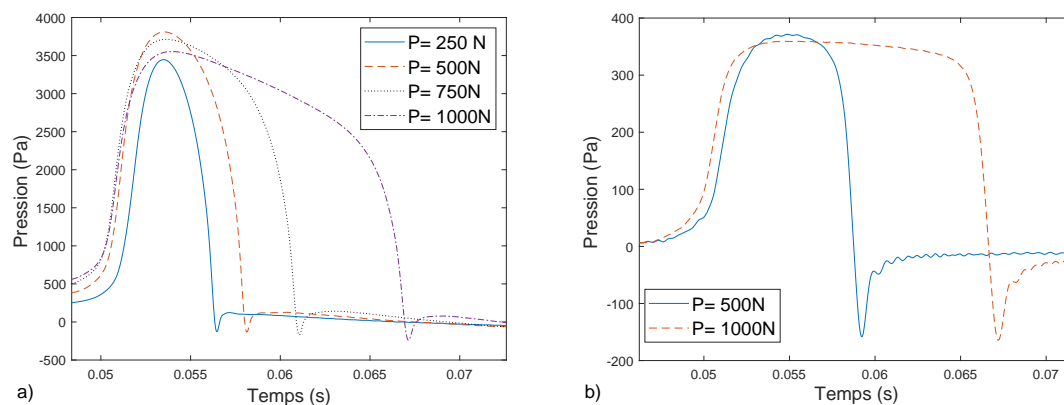
Figure 3.19 – Variation de la pression au fond de la cavité en fonction de la charge appliquée ( d = 5 mm, v = 2,5 m/s) a) L_0 = 1 mm, b) L_0 = 30 mm.
