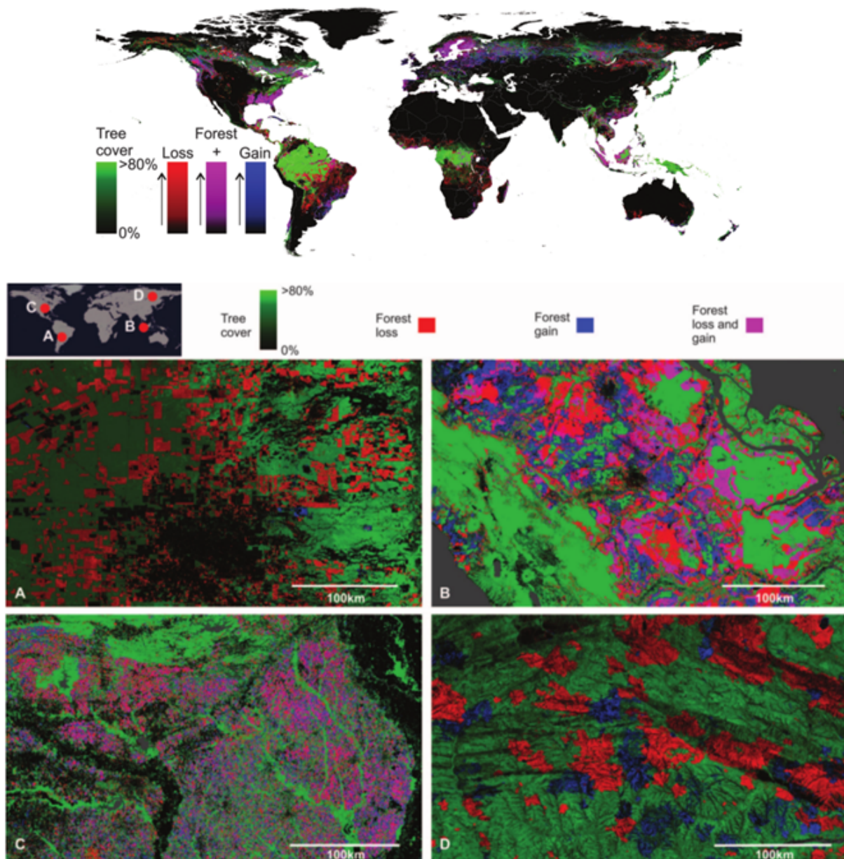
Figure 36 : Illustration de la « carte de Hansen ». Carte mondiale des changements de couverture arborée pour la période 2000-2012. Extrait de Hansen et al, 2013.
