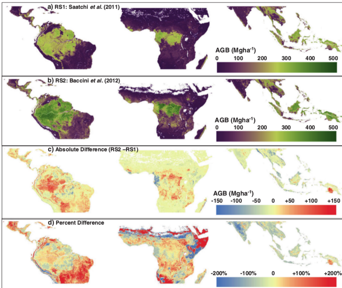
Figure 7. Comparaison de deux cartographies de la biomasse aérienne (AGB) par satellites dans la ceinture inter-tropicale : a) AGB de la carte de Saatchi et al 2011. b) Carte AGB de Baccini et al, 2012. c) la différence absolue entre a et b. d) le pourcentage de différence entre les deux cartes. Extrait de Mitchard et al, 2013.
