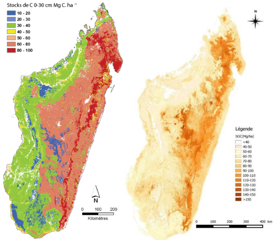
Figure 39 : Cartographie des stocks de carbone dans le sol sur 0-30 centimètres. A Gauche Grinand et al, 2009 et à droite, Ramifehiarivo et al, 2016.
