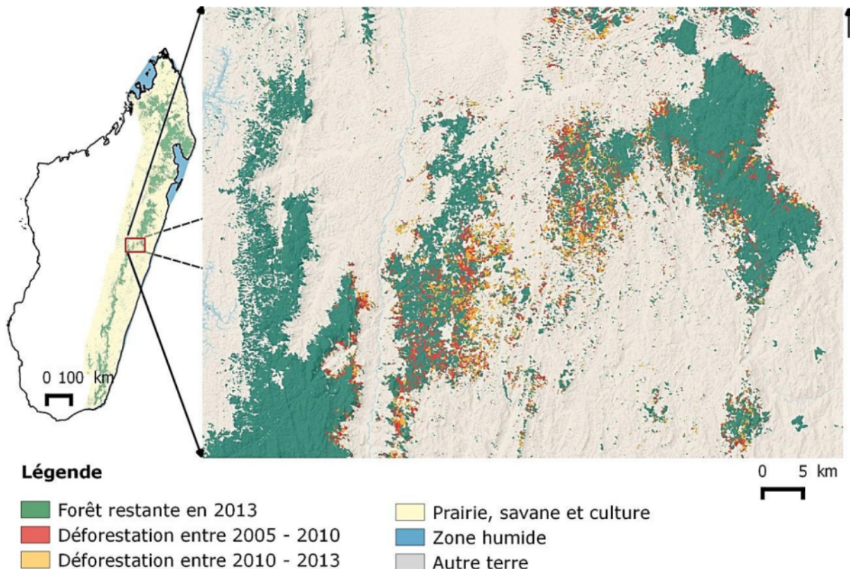
Figure 37 : Carte de l'historique de la déforestation dans l'écorégion humide de l'Est de Madagascar avec un zoom sur une zone à forte intensité (hot spot) de déforestation. Extrait de Rakotomalala et al, 2015
