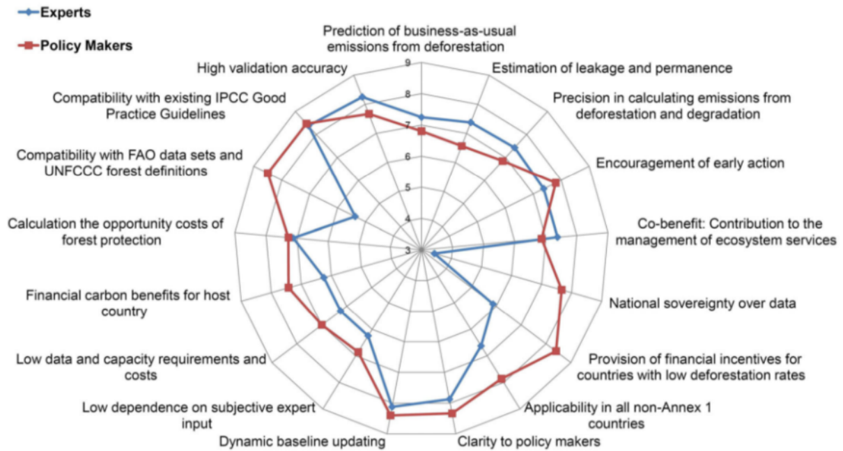
Figure 44 : Résultats de l'évaluation des critères d'importance pour le choix des méthodes d'établissement de scénario de référence REDD+ nationaux, selon les experts scientifiques (en bleu) et les décideurs (en rouge). Les valeurs à 0 indique une faible importance et les valeurs à 10 une forte importance. Extrait de Huettner et al, 2009.
