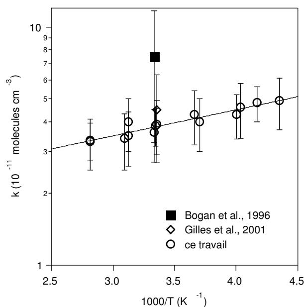
Figure 4 : Dépendance en température du coefficient de vitesse de la réaction BrO + OH
