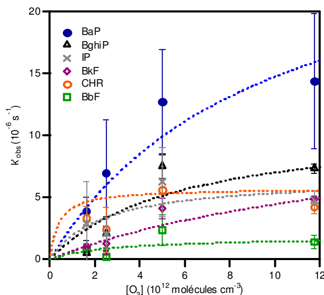
Figure 16 : Coefficient de vitesse de pseudo-premier ordre ( s^{-1} ) à 288 K pour 6 HAP adsorbés sur des particules réelles en fonction de la concentration en ozone (molécules cm^{-3} ) ( n = 4 ; incertitude : \pm 1\sigma )
